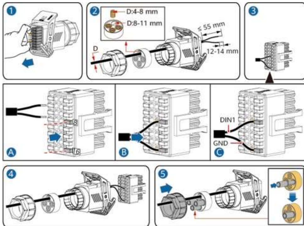
Figura 5-32 Instalarea cablului
