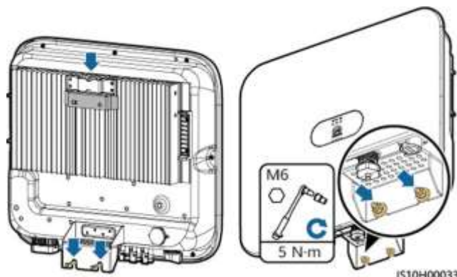
Figura 4-11 Instalarea unui invertor SUN2000
