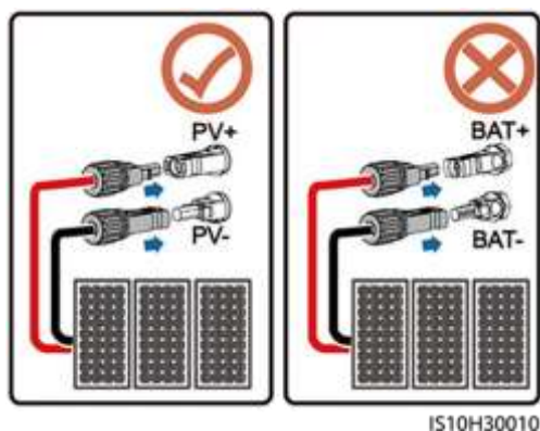
Figura 5-12 Cablarea corectă a bornelor
