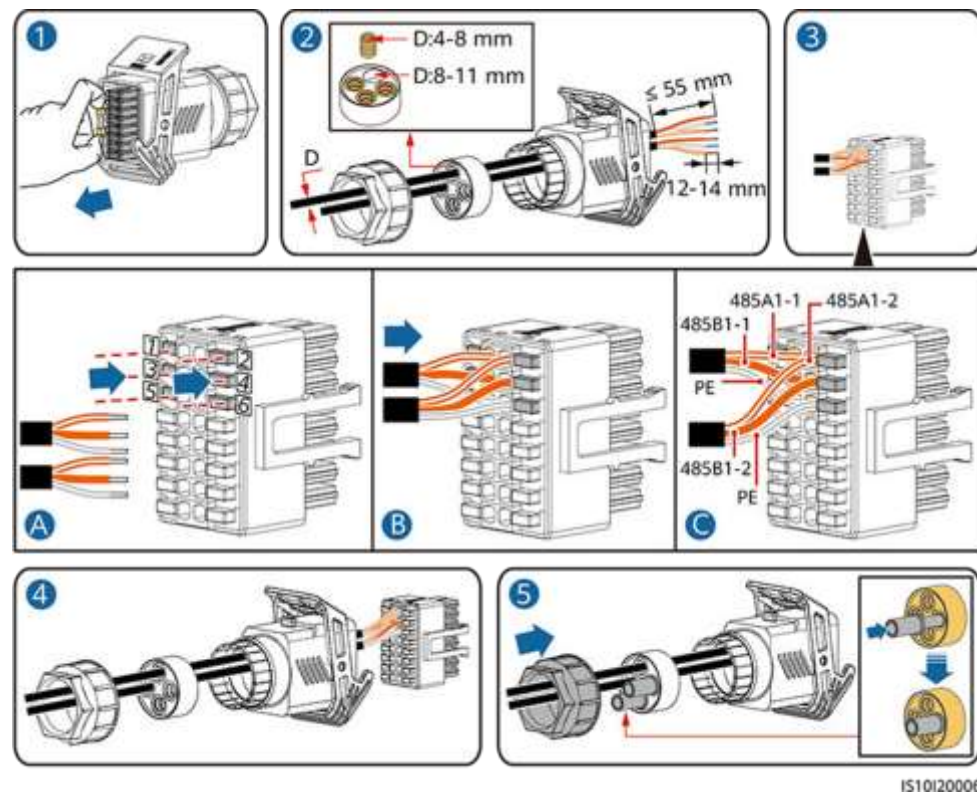
Figura 5-21 Instalarea cablului
