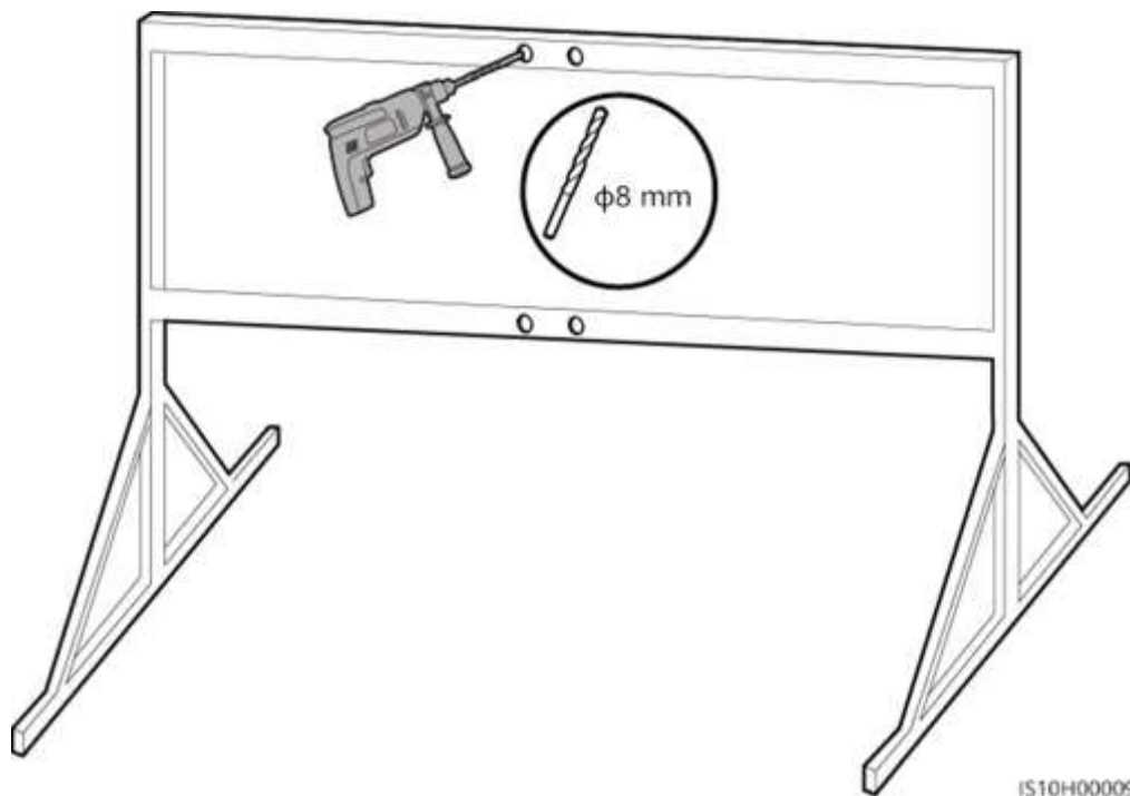
Figura 4-14 Efectuarea găurilor
