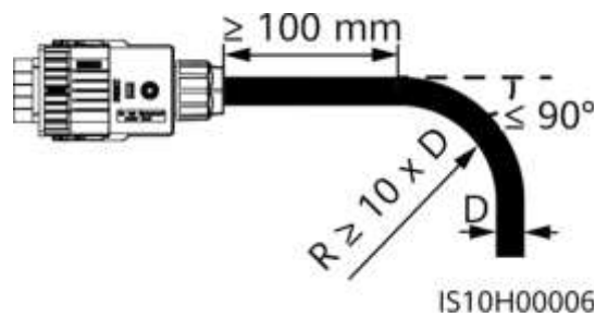
Figura 5-10 Traseul cablului
