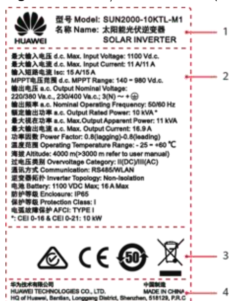
Figura 2-5 Plăcuța de identificare (folosind SUN2000-10KTL-M1 ca exemplu)
