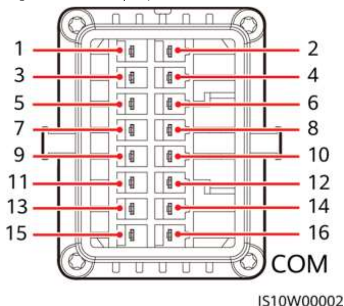
Figura 5-18 Definițiile pinilor
