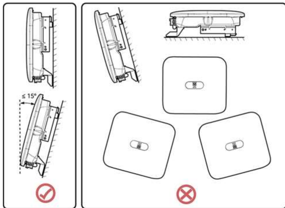
Figura 4-1 Unghiurile de instalare
