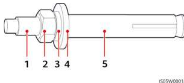
Figura 4-8 Componenta șurubului conexpand
