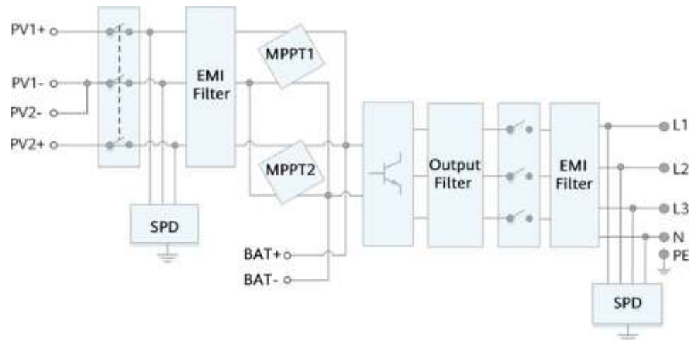
Figura 2-6 Schema conceptuală a invertorului SUN2000
