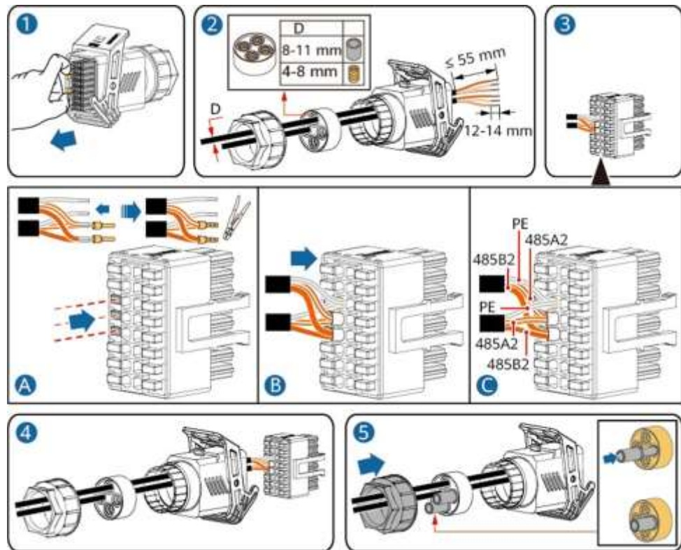
Figura 5-27 Instalarea cablului
