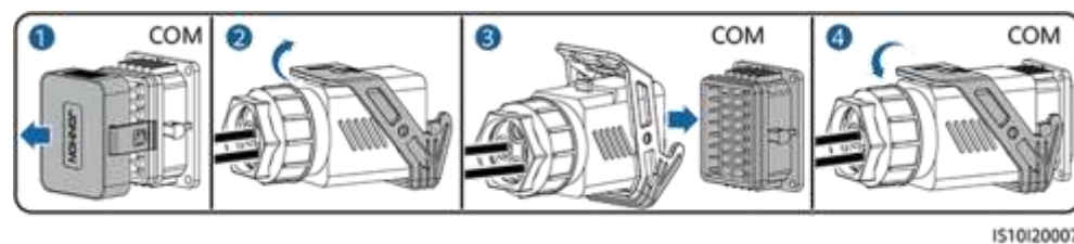
Figura 5-22 Fixarea conectorului cablului de semnal
