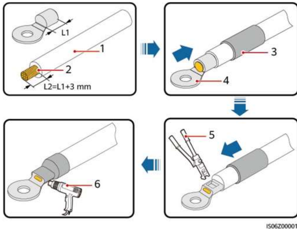
Figura 5-2 Sertizarea bornei OT
