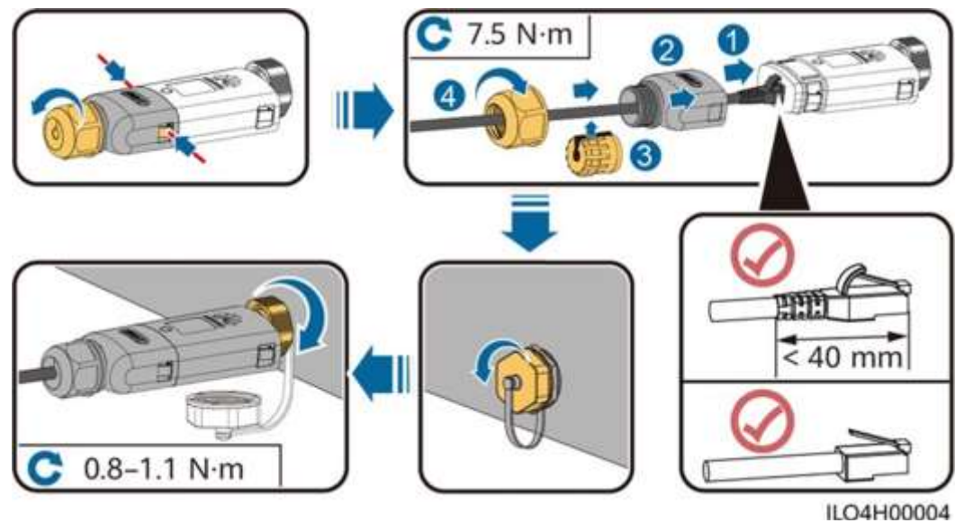
Figura 5-16 Instalarea unui WLAN-FE Smart Dongle (comunicare FE)
