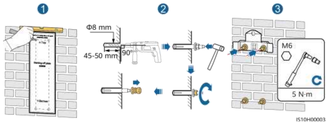
Figura 4-9 Instalarea suportului de montare
