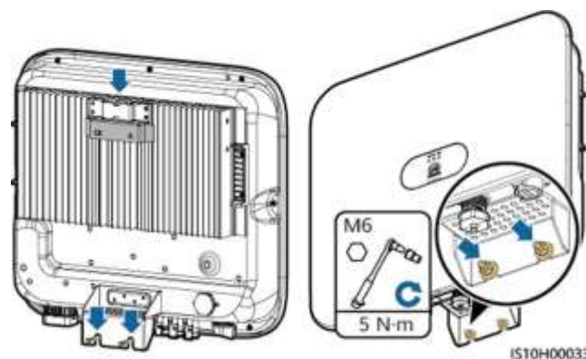
Figura 4-17 Instalarea unui invertor SUN2000
