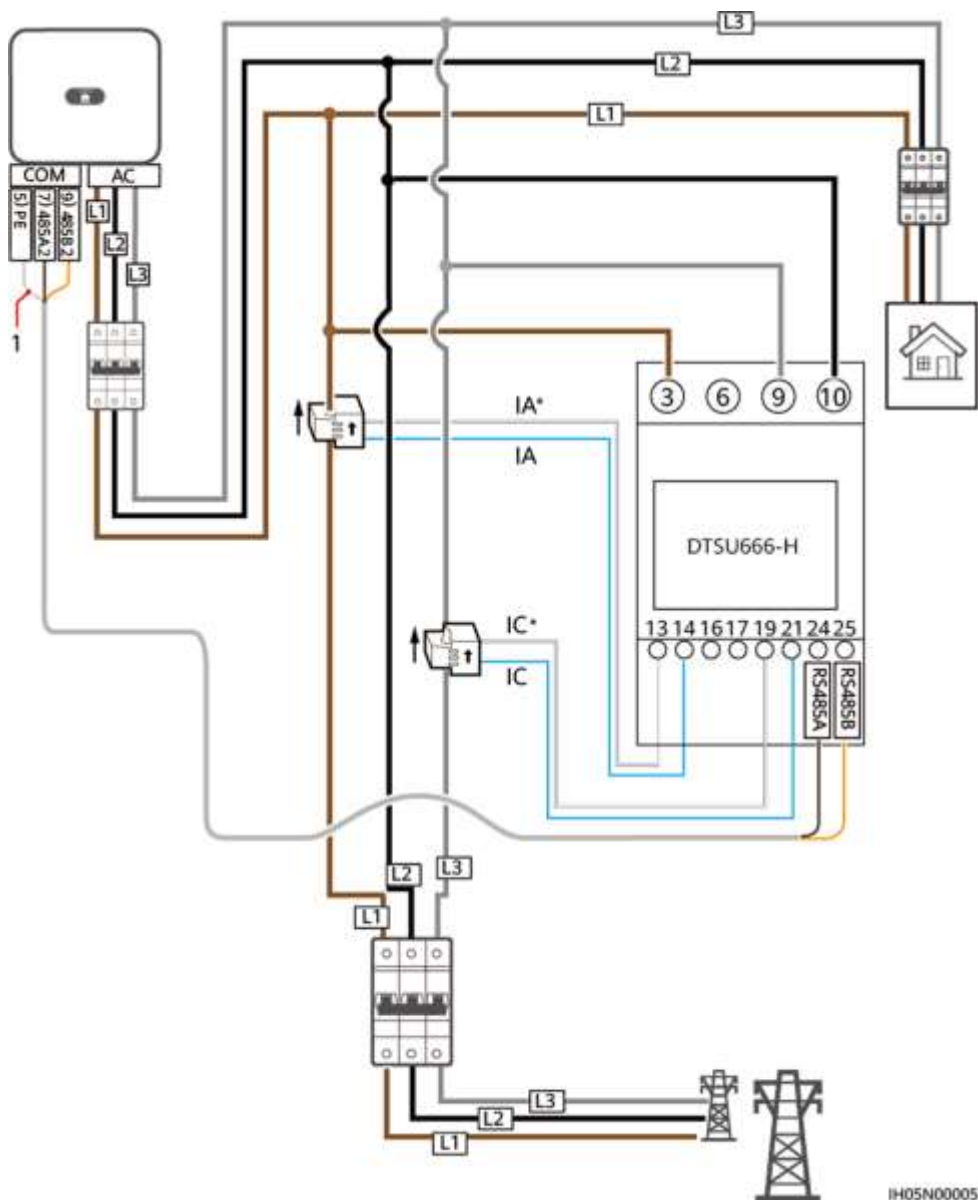
Figura 5-23 Conexiunea cablului (trifazat cu trei fire)
