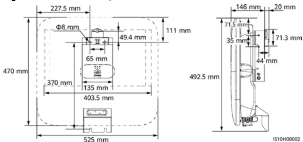
Figura 4-7 Dimensiunile suportului de montare
