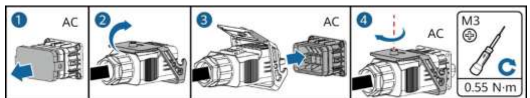
Figura 5-9 Fixarea conectorului de curent alternativ
