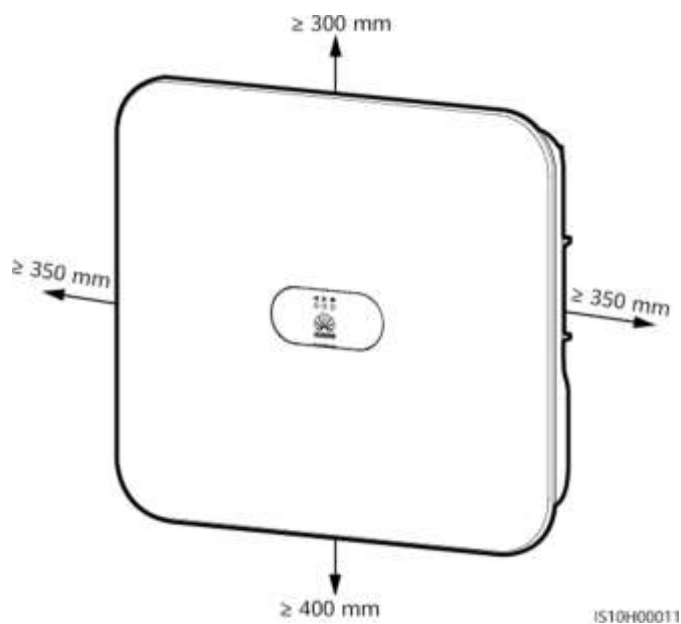
Figura 4-2 Spațiu de instalare
