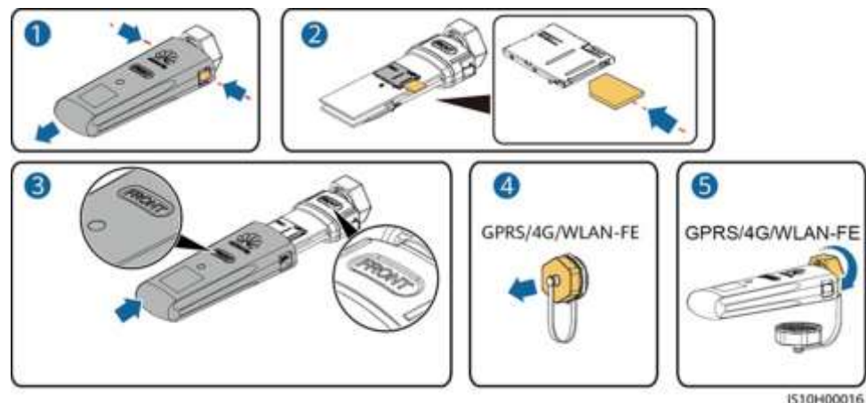
Figura 5-17 Instalarea unui 4G Smart Dongle
