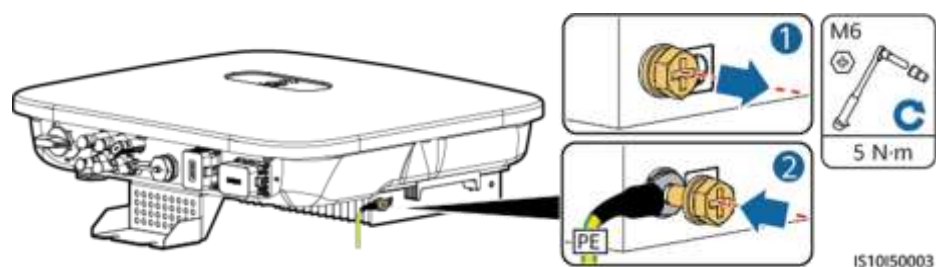
Figura 5-3 Conectarea cablului PE
