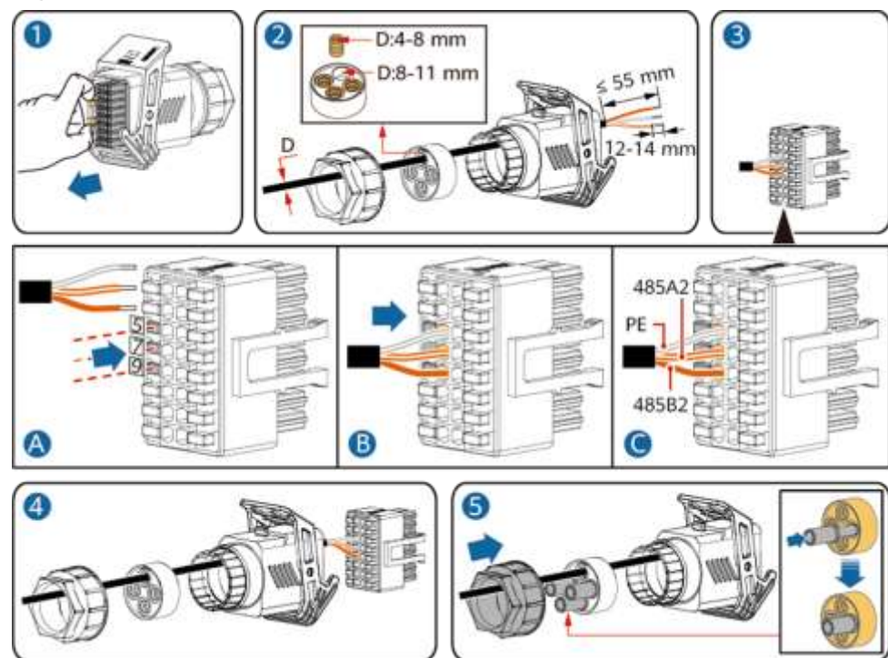
Figura 5-25 Instalarea cablului
