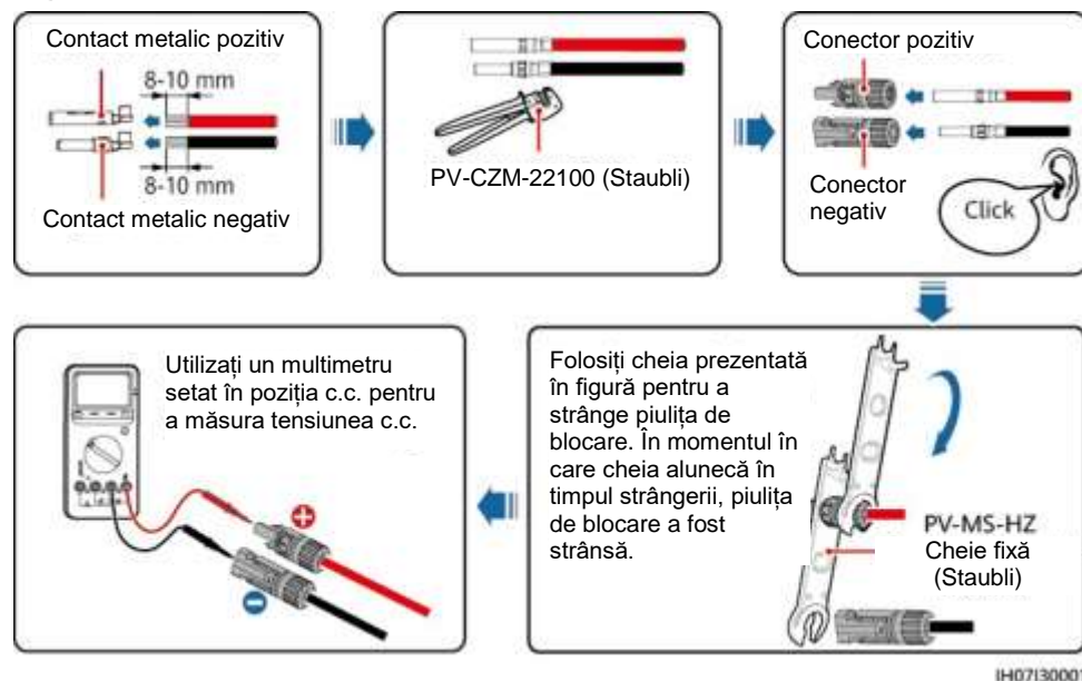
Figura 5-13 Instalarea cablurilor de alimentare de intrare c.c.
