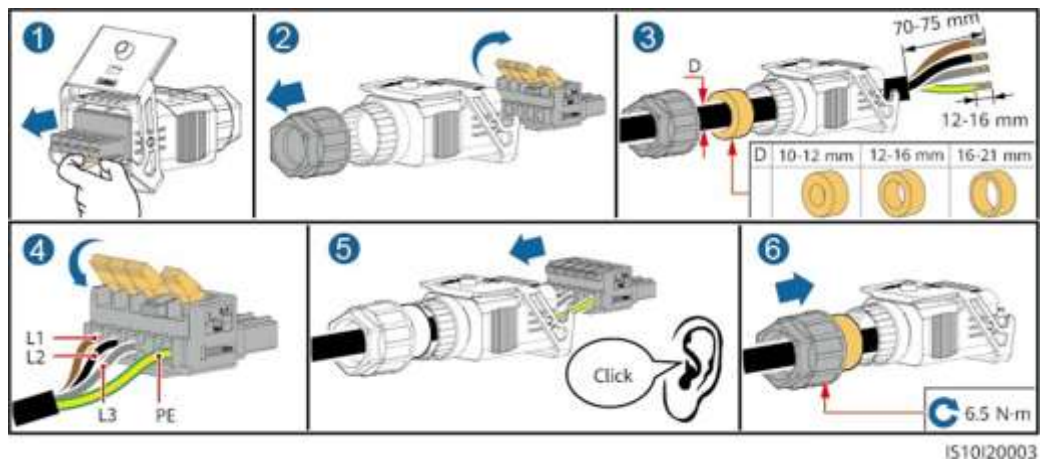
Figura 5-6 Cablu cu patru fire (L1, L2, L3 și PE)
