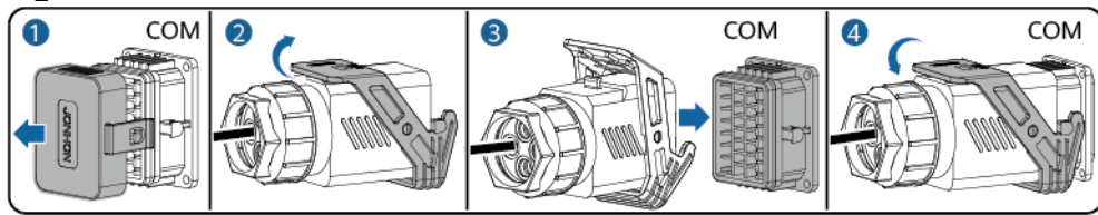
Figura 5-33 Fixarea conectorului cablului de semnal
