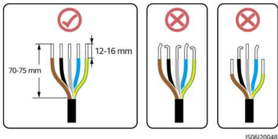
Figura 5-4 Cerințe privind dezizolarea
