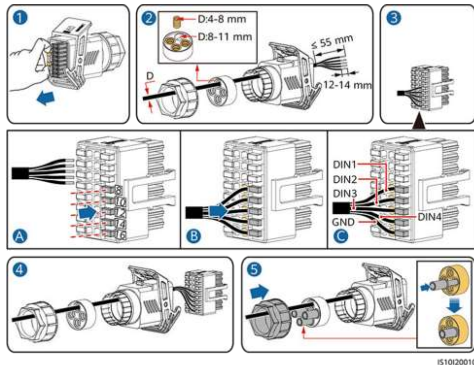
Figura 5-30 Instalarea cablului
