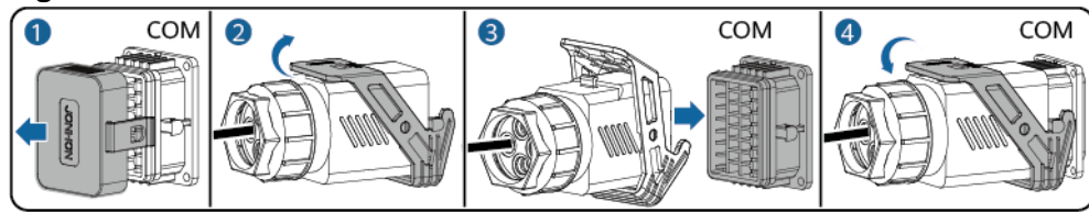
Figura 5-31 Fixarea conectorului cablului de semnal
