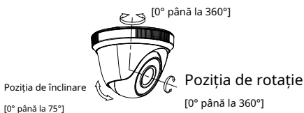
Figura 2-7 Reglarea 3-Aixs
