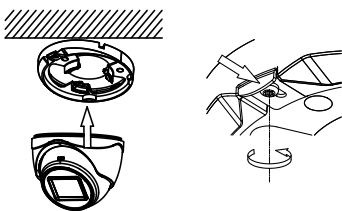
Figura 2-18 Instalați camera
