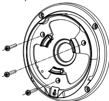
Figura 2-21 Șuruburi de fixare pe capacul cutiei de jonctiune
