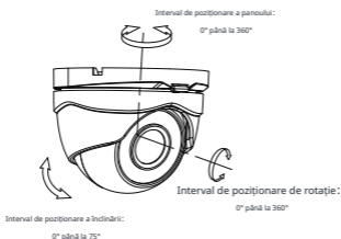
Figura 2. 8 Reglare pe 3 axe
