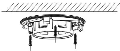
Figura 2. 10 Atașați baza de montare la tavan
