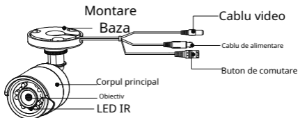
Figura 1. 1 Prezentare generală a camerei de tip I
