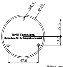
Figura 2. 1 Șablon de foraj
