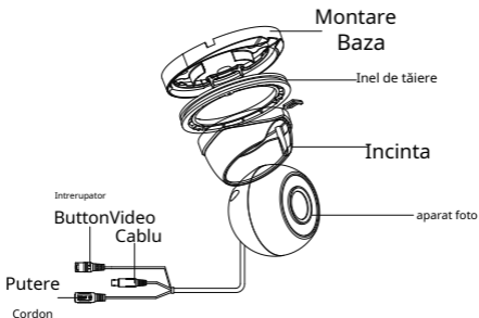
Figura 1. 2 Prezentare generală a camerei de tip II
