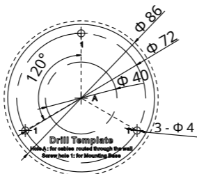
Figura 2. 9 Șablon de foraj
