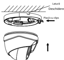
Figura 2. 7 Asigurați camera cu baza de montare
