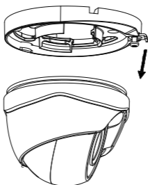
Figura 2. 4 Dezasamblați camera
