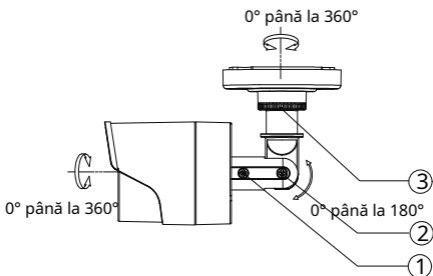
Figura 2. 3 Ajustarea pe 3 axe
