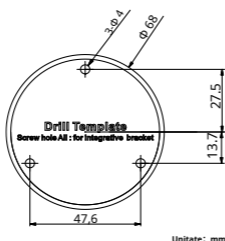
Figura 2. 5 Șablon de foraj
