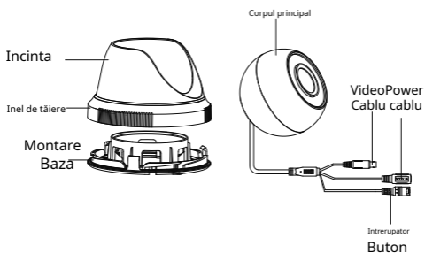
Figura 1. 3 Prezentare generală a camerei de tip III
