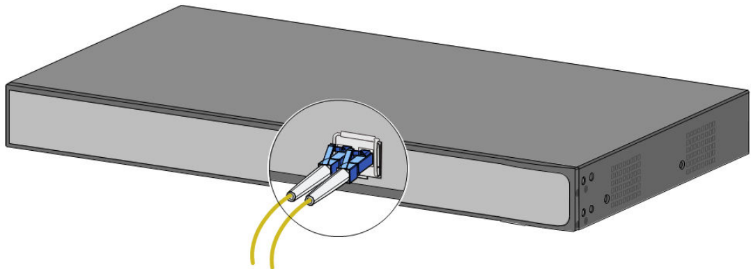
Figura 4-5 Conectarea fibrei optice
