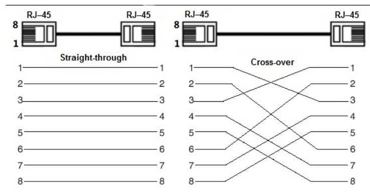
Figura 4-3 Descrierea pinului
