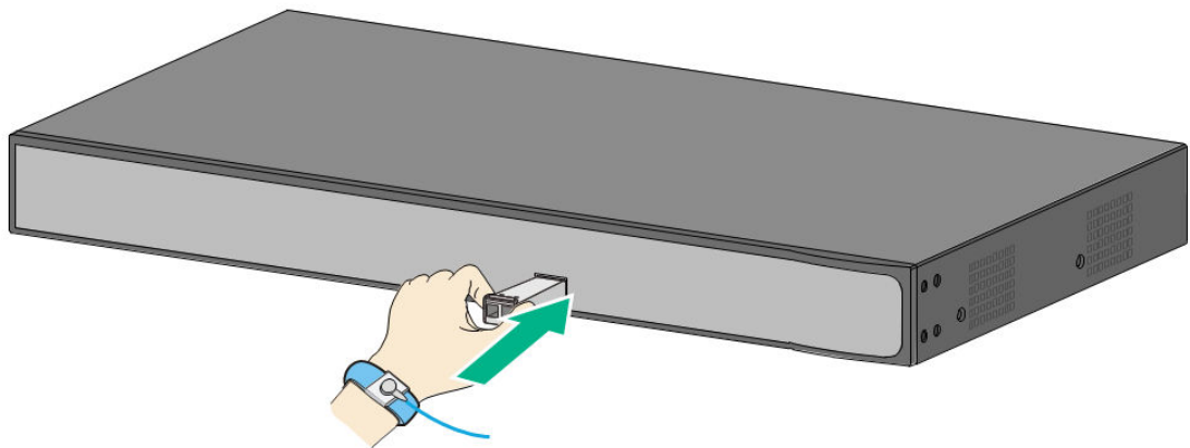
Figura 4-4 Instalați modulul SFP
