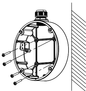
Figura 2-19 Asigurați corpul cutiei de joncțiune
