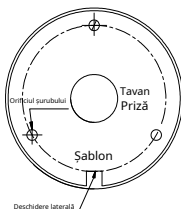
Figura 2-8 Șablon de foraj
