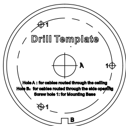
Figura 2-13 Șablon de foraj
