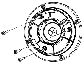
Figura 2-18 Fixați șuruburile pe capacul cutiei de joncțiune
