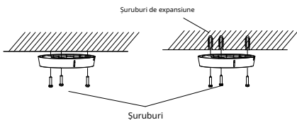
Figura 2-14 Atașați baza de montare la tavan
