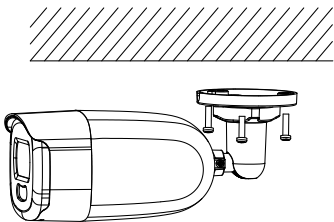
Figura 2-9 Fixați camera de tavan
