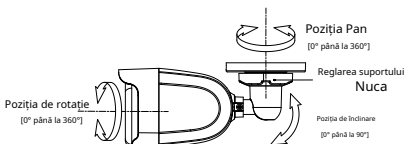
Figura 2-3 Ajustarea pe 3 axe
