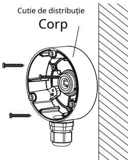
Figura 2-6 Fixați cutia de joncțiune pe perete/tavan
