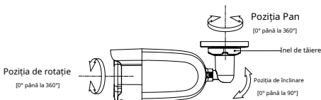
Figura 2-10 Ajustarea pe 3 axe
