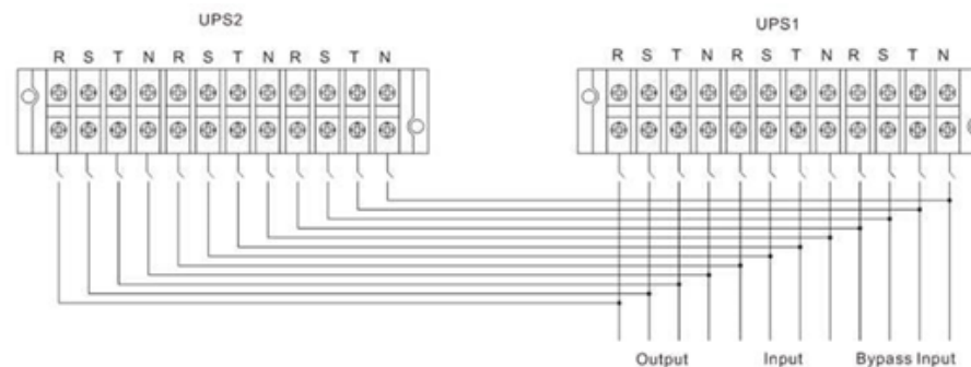
Diagrama pentru sistemul paralel Garun 10KL, 15KL, 20KL
