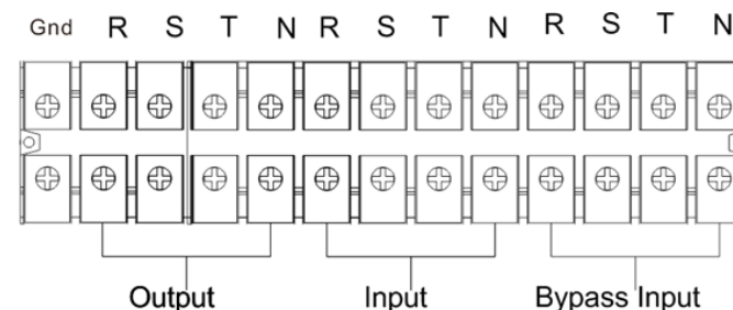
Diagrama 2: Schema de conectare cabluri pentru Garun 10KL/15KL/20KL (configurație faze 3:3)
