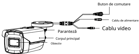
Figura 1-2 Prezentare generală a camerei de tip II
