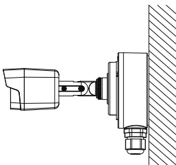
Figura 2-7 Fixați capacul cutiei de joncțiune înapoi la el Corp
