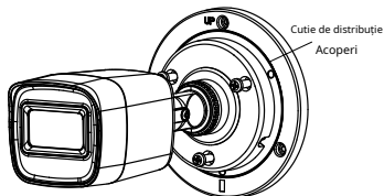
Figura 2-5 Fixați camera pe capacul cutiei de joncțiune
