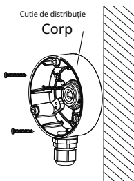
Figura 2-6 Fixați cutia de joncțiune pe perete/tavan
