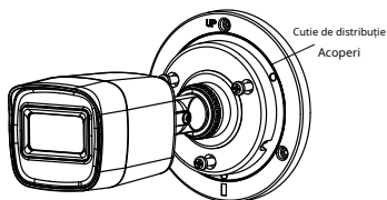
Figura 2-5 Fixați camera pe capacul cutiei de joncțiune
