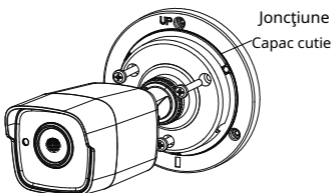
Figura 2-5 Fixați camera pe capacul cutiei de joncțiune
