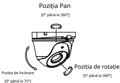
Figura 2-10 Reglare pe 3 axe
