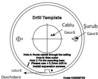
Figura 2-2 Șablon de foraj
