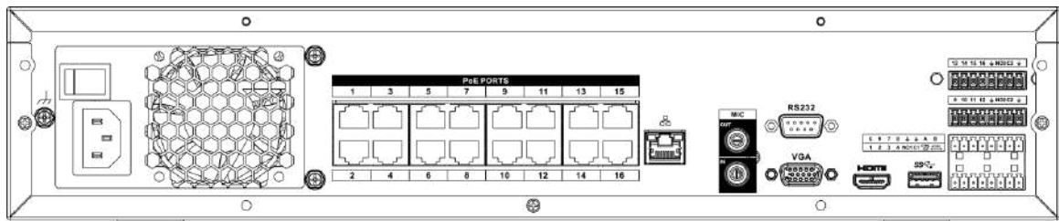
Figura 2-77 Panoul din spate
