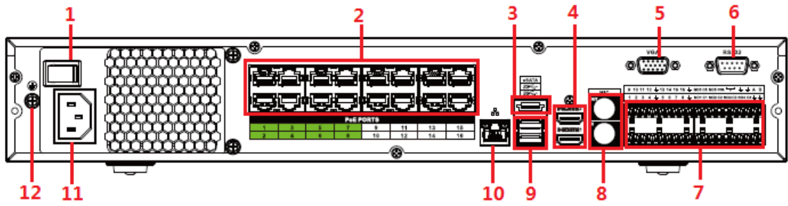
Figura 2-100 Panoul din spate (2)
