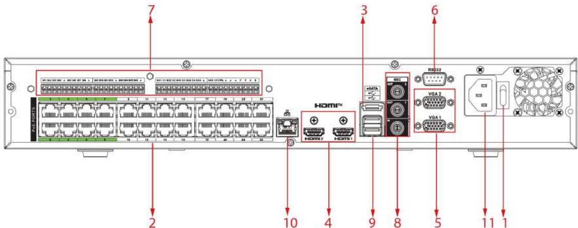
Figura 2-102 Panoul din spate (4)
