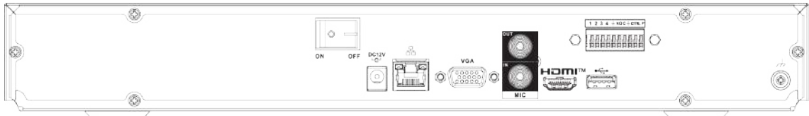
Figura 2-69 Panoul din spate
