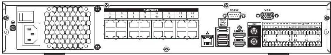
Figura 2-62 Panoul din spate
