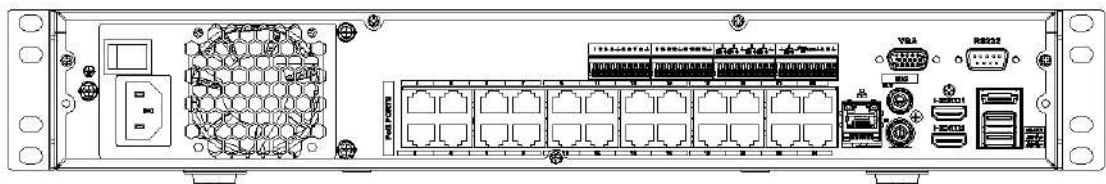
Figura 2-63 Panoul din spate
