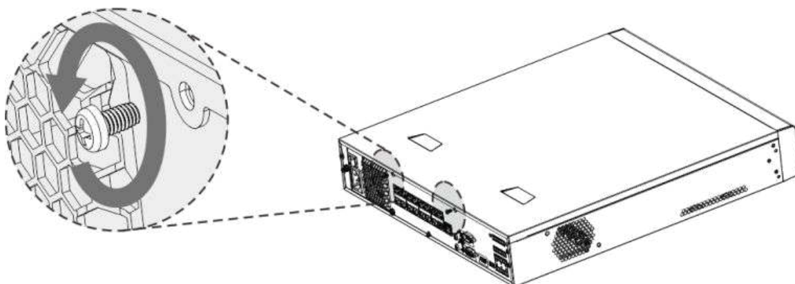
Figura 3-18 Scoateți șuruburile
