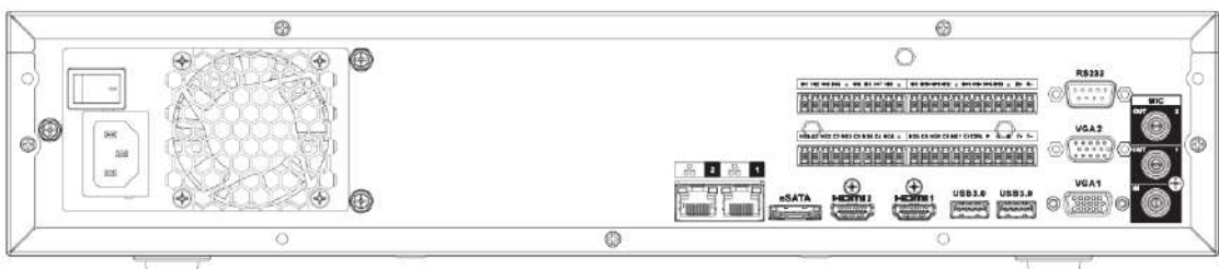
Figura 2-119 Panoul din spate
