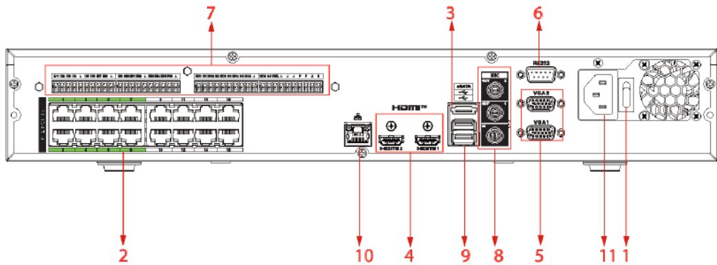
Figura 2-102 Panoul din spate (4)
