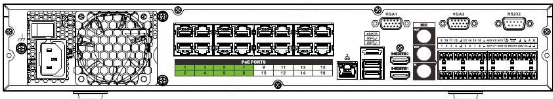
Figura 2-64 Panoul din spate
