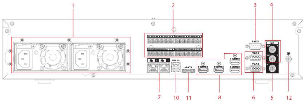
Figura 2-110 Panoul din spate (5)
