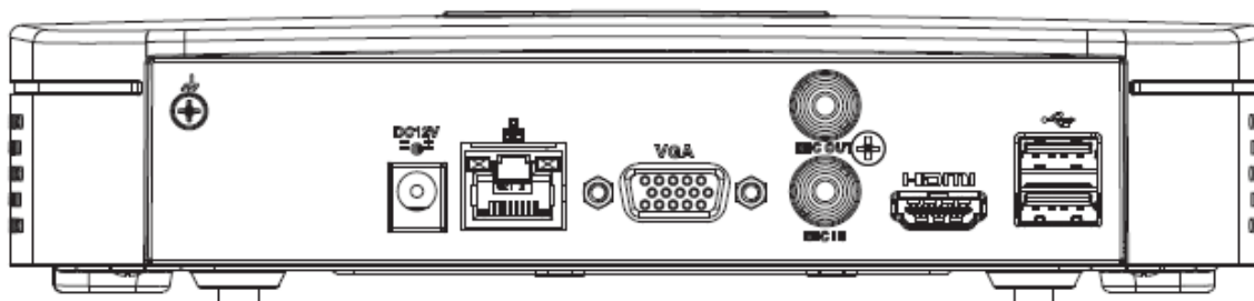
Figura 2-66 Panoul din spate
