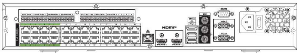
Figura 2-124 Panoul din spate
