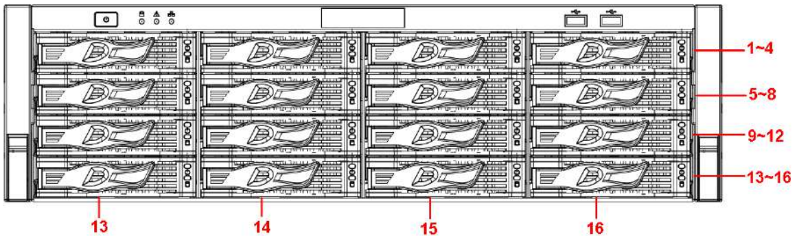
Figura 2-34 Panoul frontal
