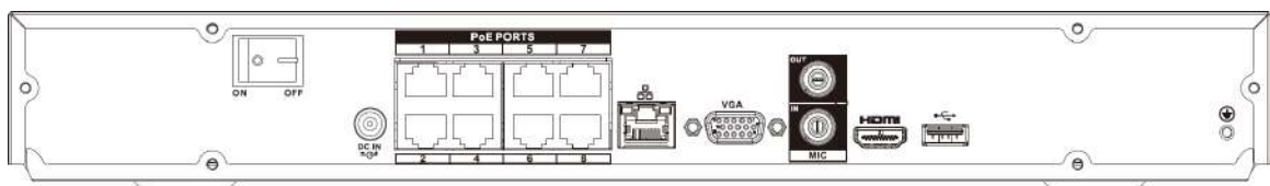
Figura 2-89 Panoul din spate
