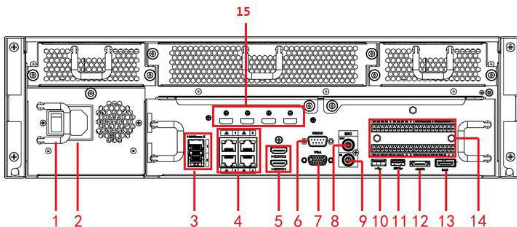
Figura 2-112 Panoul din spate
