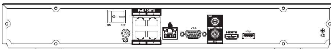
Figura 2-87 Panoul din spate
