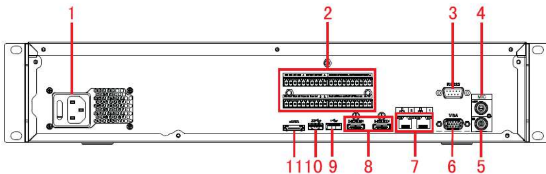
Figura 2-107 Panoul din spate (2)
