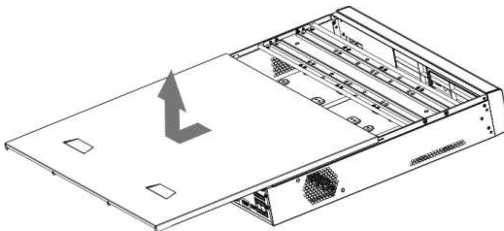
Figura 3-19 Scoateți capacul
