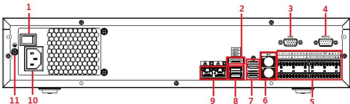
Figura 2-97 Panoul din spate (1)
