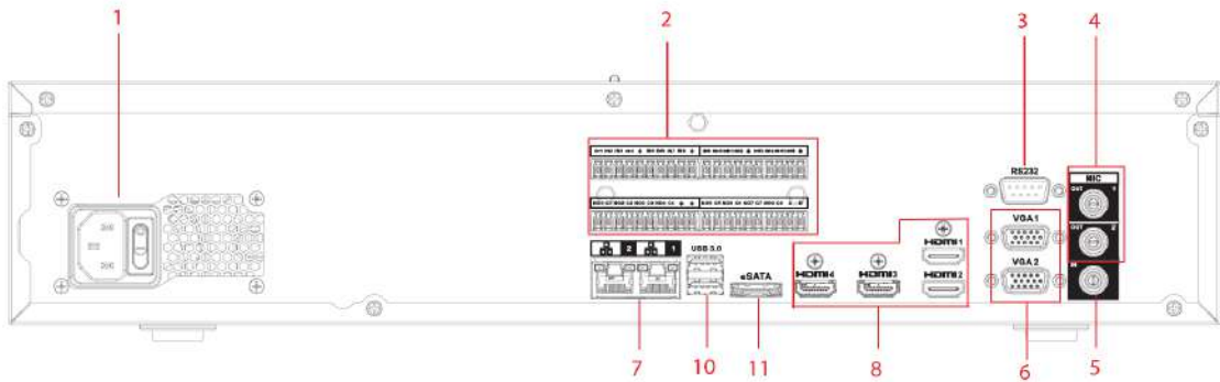
Figura 2-109 Panoul din spate (4)
