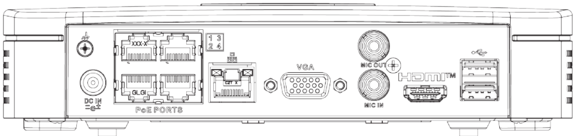
Figura 2-38 Panoul din spate
