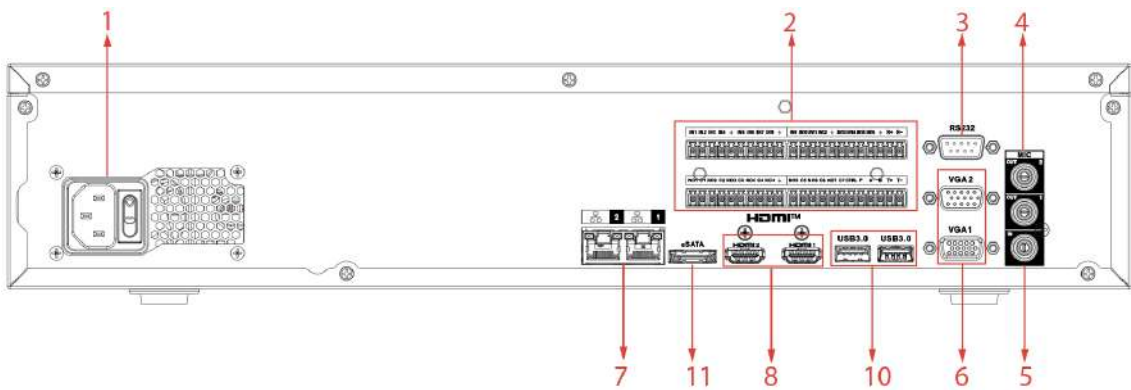
Figura 2-109 Panoul din spate (4)
