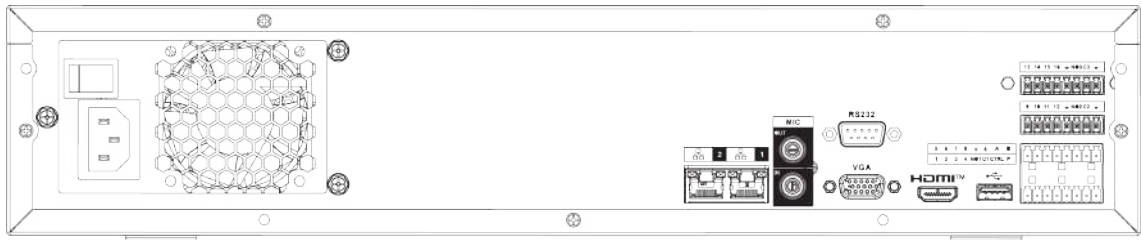
Figura 2-76 Panoul din spate
