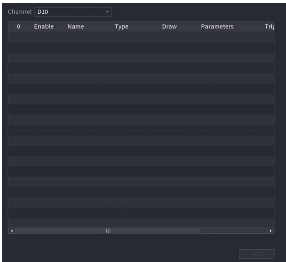
Figura 5-190 Densitatea vehiculului
