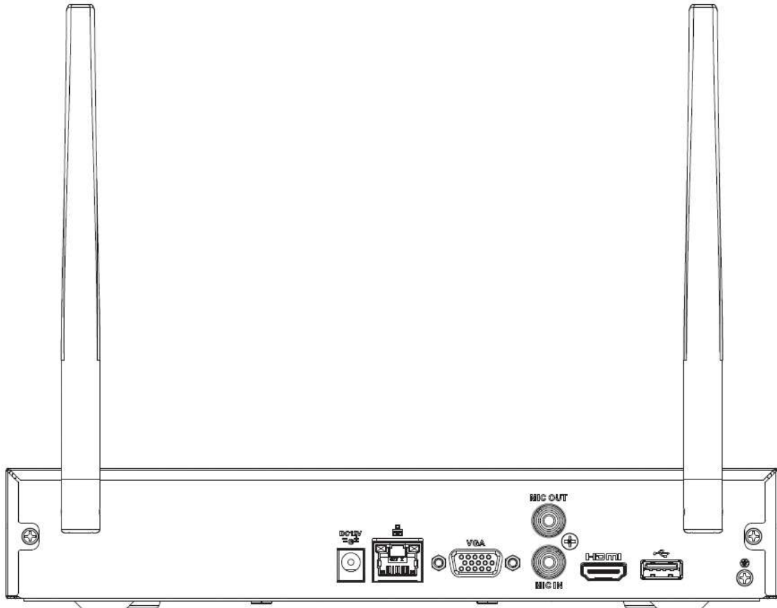
Figura 2-117 Panoul din spate
