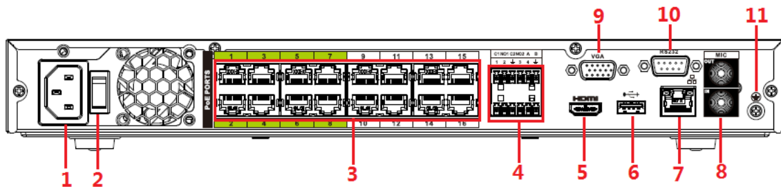
Figura 2-103 Panoul din spate
