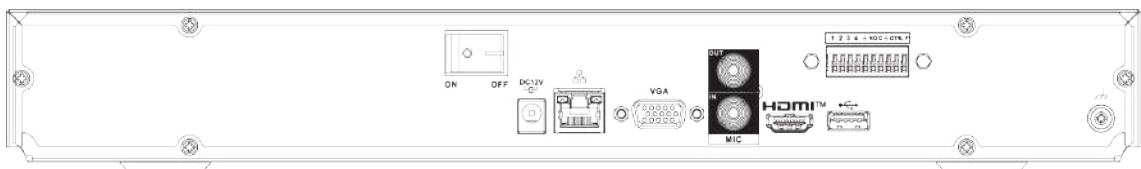
Figura 2-84 Panoul din spate (3)
