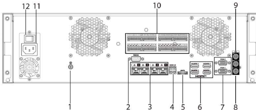
Figura 2-114 Panoul din spate
