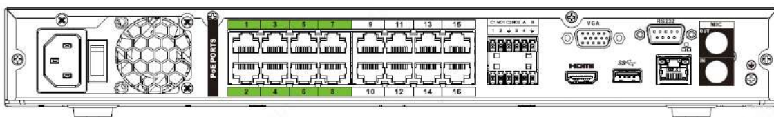
Figura 2-54 Panoul din spate
