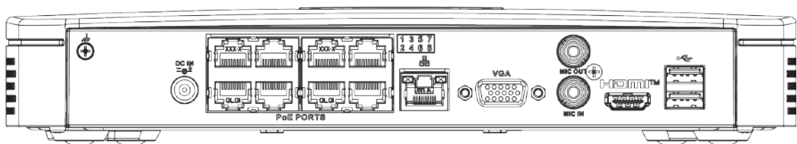
Figura 2-88 Panoul din spate
