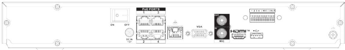
Figura 2-70 Panoul din spate
