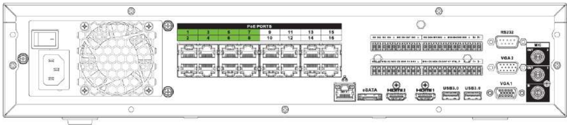
Figura 2-121 Panoul din spate
