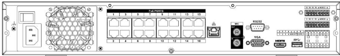
Figura 2-74 Panoul din spate
