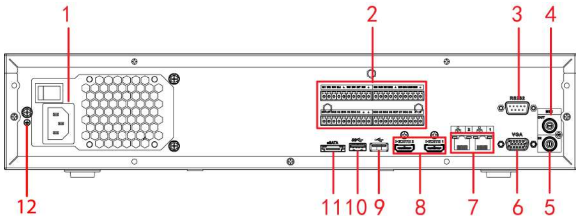
Figura 2-106 Panoul din spate (1)
