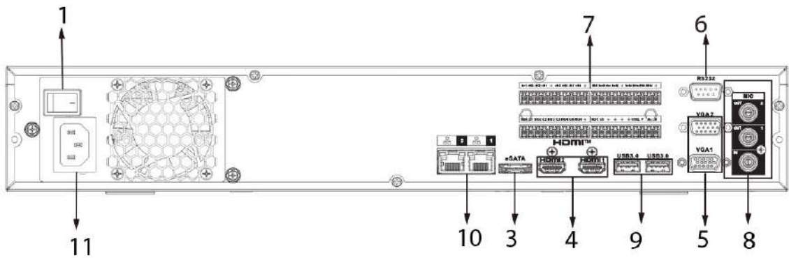
Figura 2-101 Panoul din spate (3)
