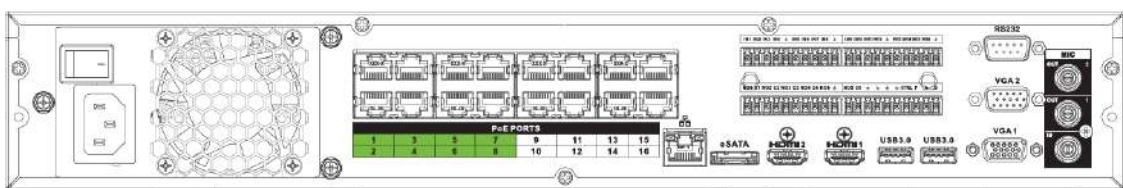
Figura 2-120 Panoul din spate
