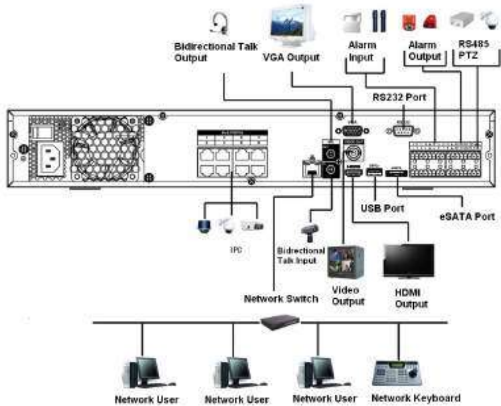
Figura 3-54 Conexiune tipică
