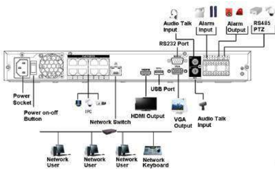
Figura 3-52 Conexiune tipică
