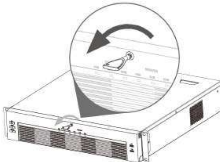
Figura 3-29 Fixați HDD
