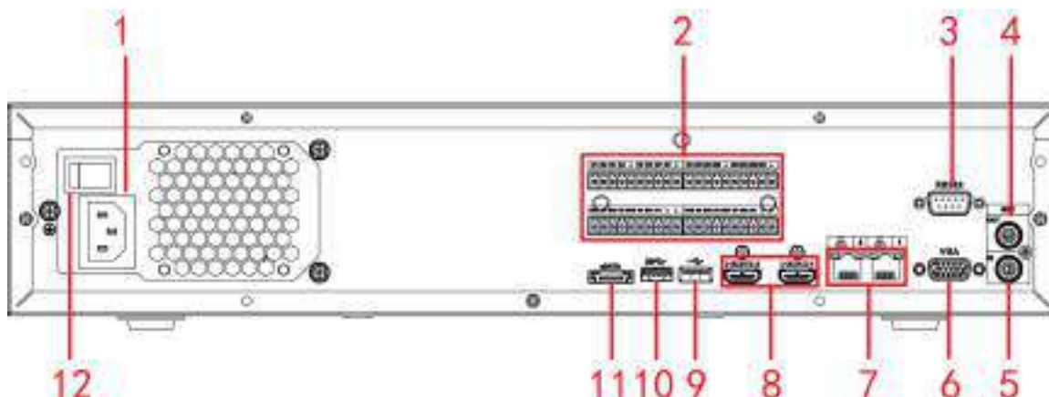
Figura 2-85 Panoul din spate (1)
