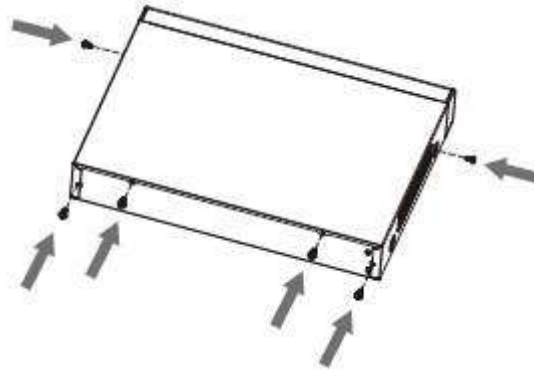
Figura 3-10 Puneți capacul înapoi
