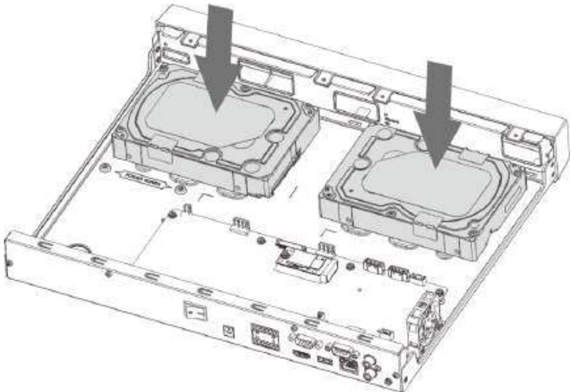
Figura 3-13 Aliniați HDD
