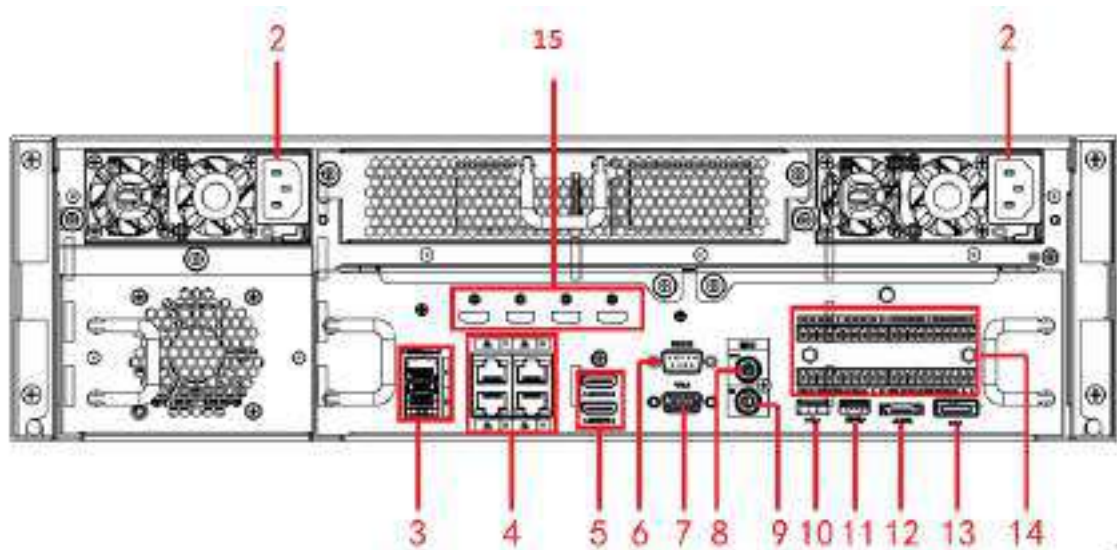
Figura 2-90 Panoul din spate
