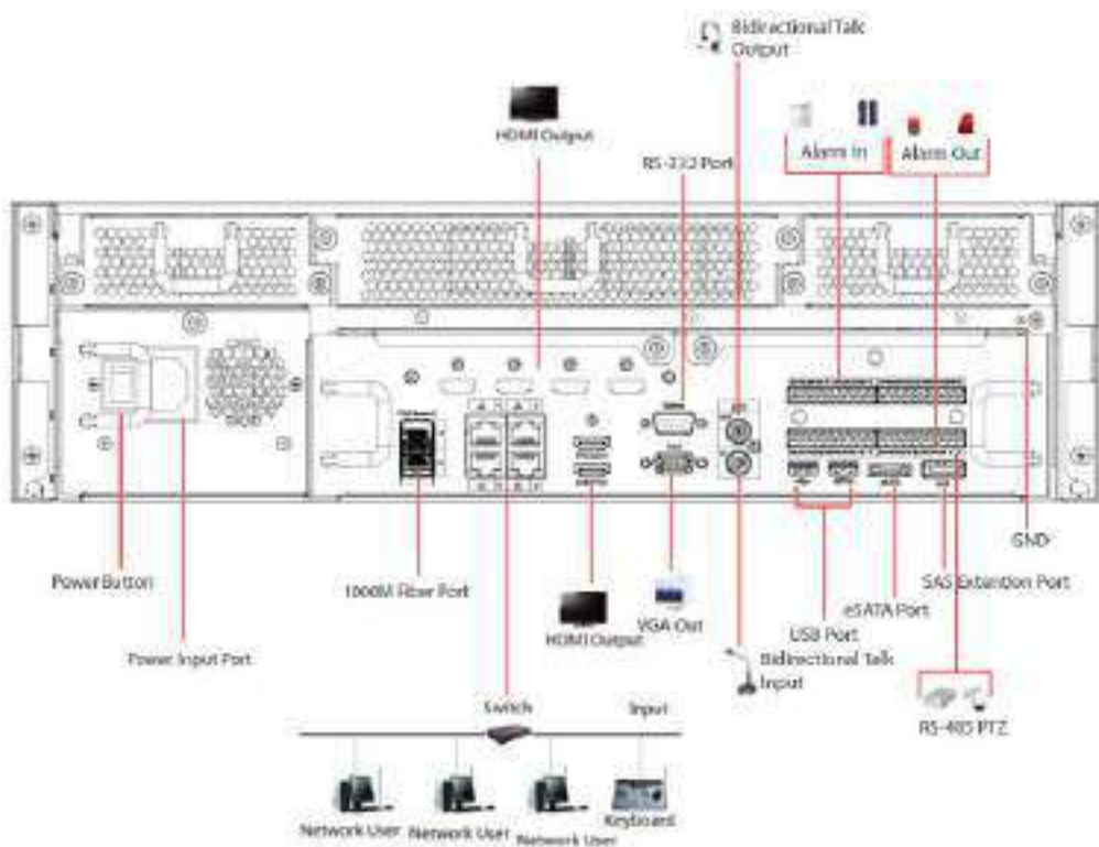
Figura 3-61 Conexiune tipică
