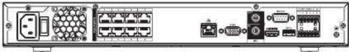
Figura 2-38 Panoul din spate
