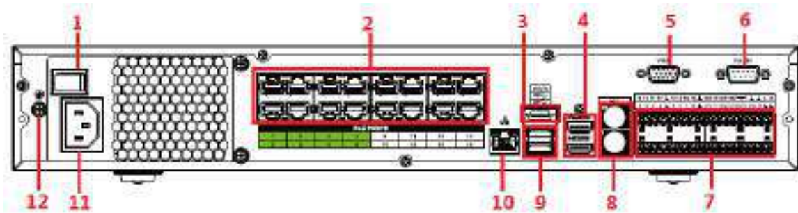
Figura 2-81 Panoul din spate
