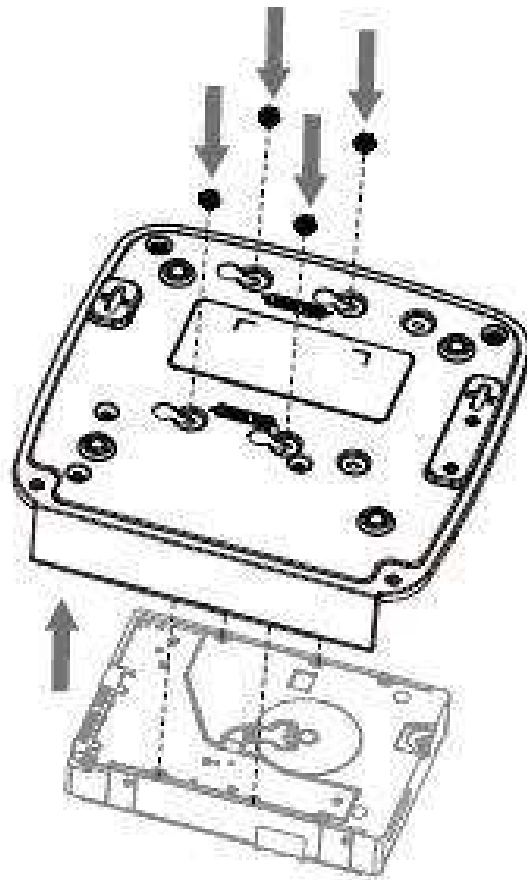
Figura 3-3 Fixați șuruburile
