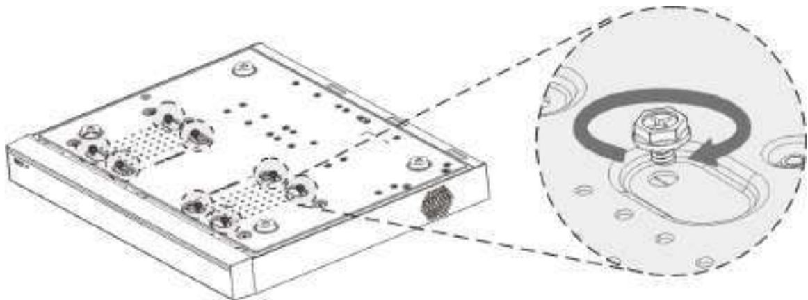
Figura 3-14 Fixați șuruburile
