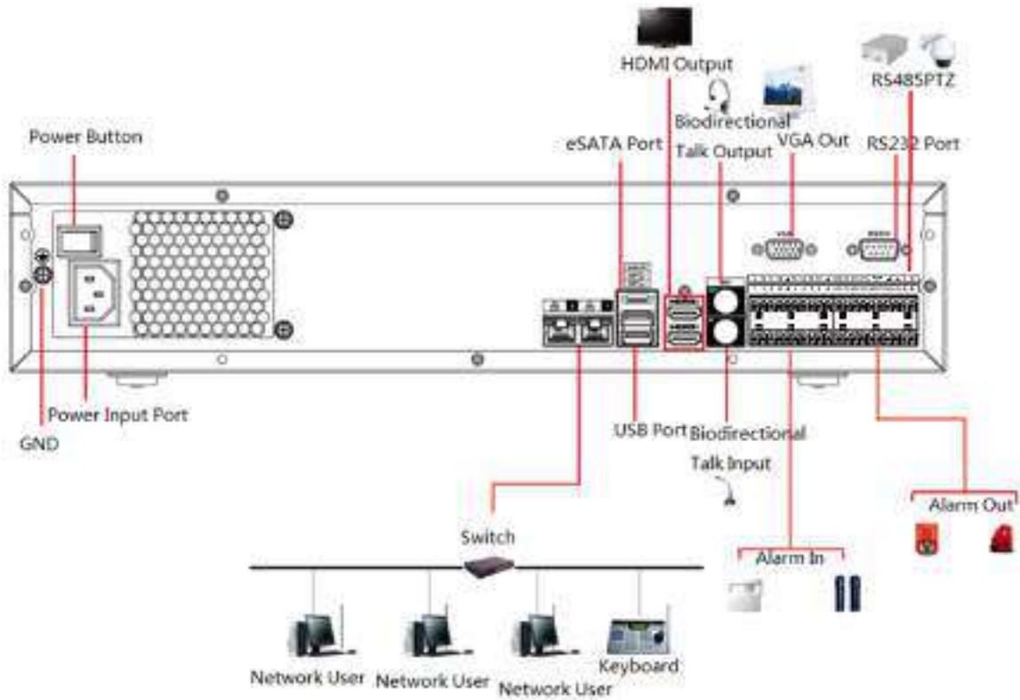
Figura 3-56 Conexiune tipică
