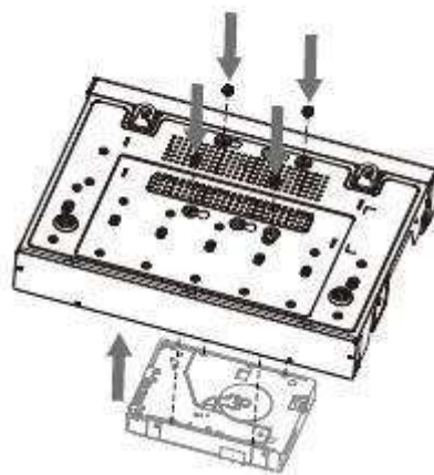
Figura 3-8 Aliniere HDD
