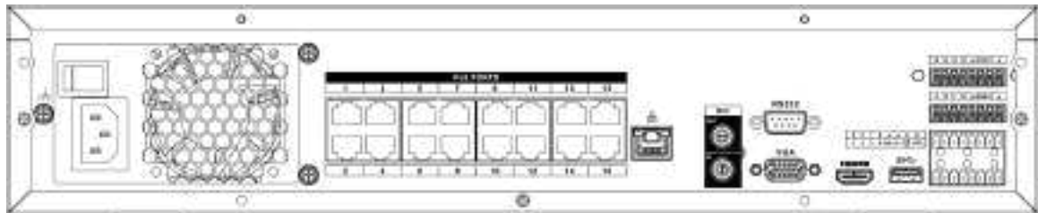
Figura 2-61 Panoul din spate
