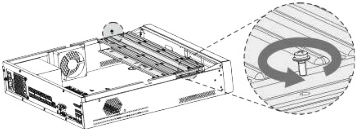
Figura 3-20 Scoateți șuruburile (2U)
