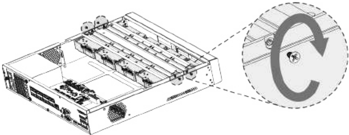
Figura 3-24 Fixați șuruburile
