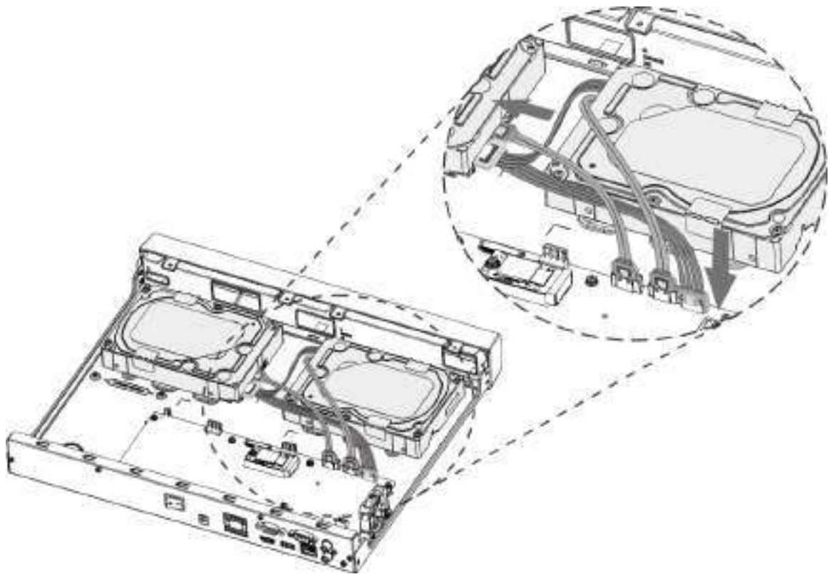
Figura 3-15 Conectați cablurile
