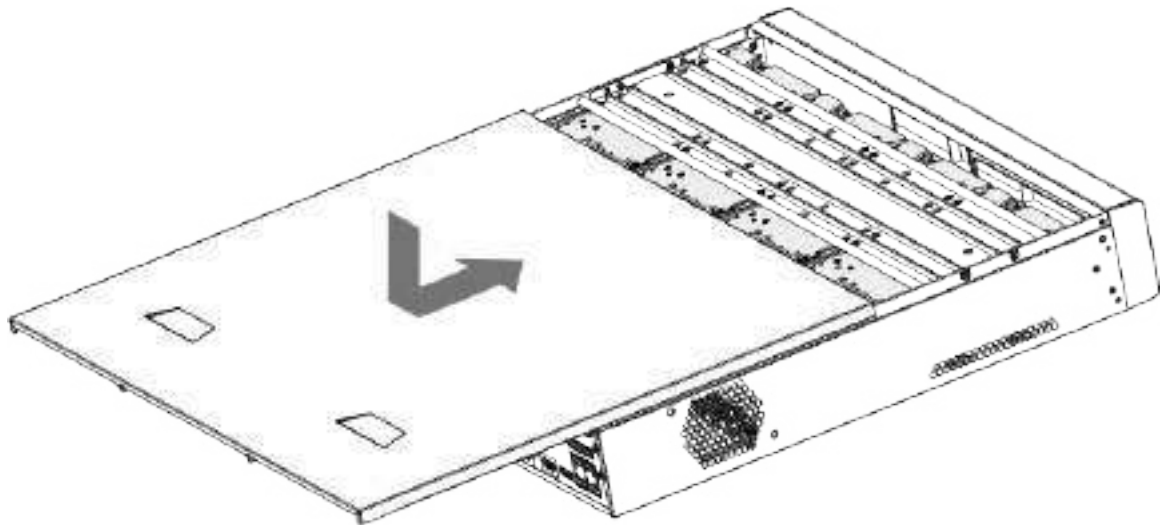
Figura 3-26 Fixați șuruburile
