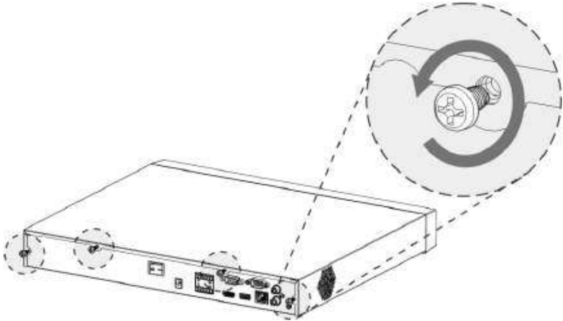
Figura 3-11 Scoateți șuruburile
