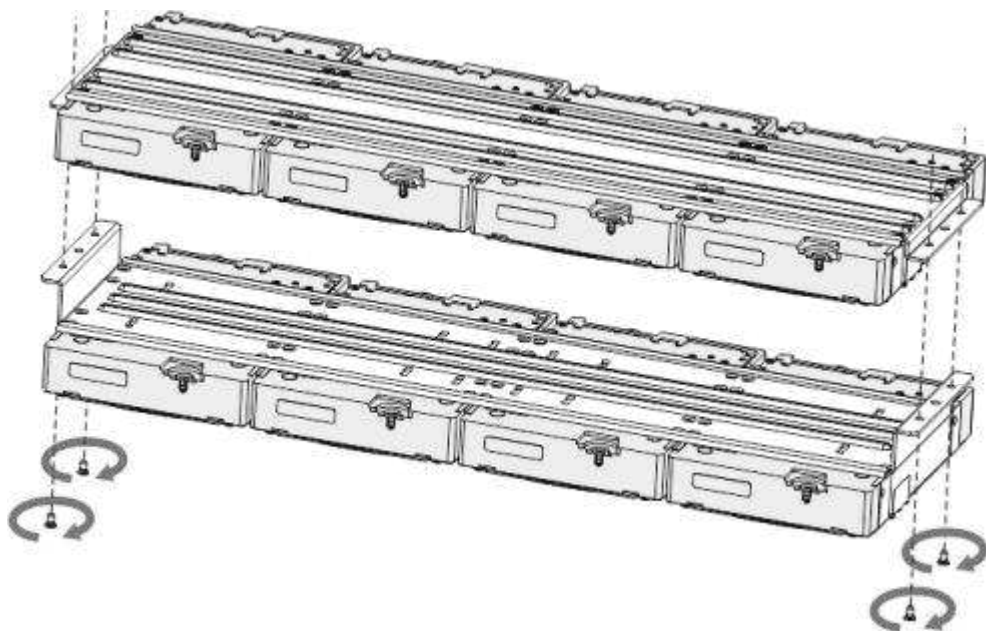
Figura 3-23 Blocare paranteze
