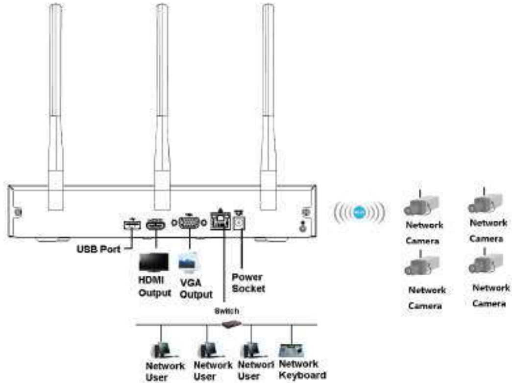
Figura 3-48 Conexiune tipică
