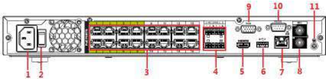
Figura 2-82 Panoul din spate
