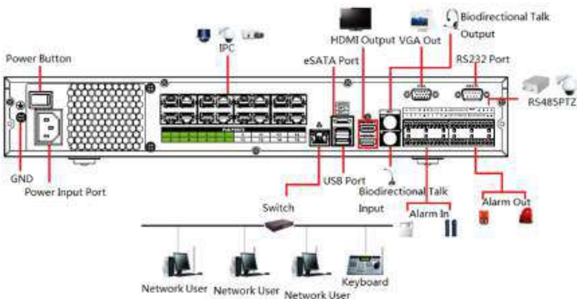
Figura 3-57 Conexiune tipică
