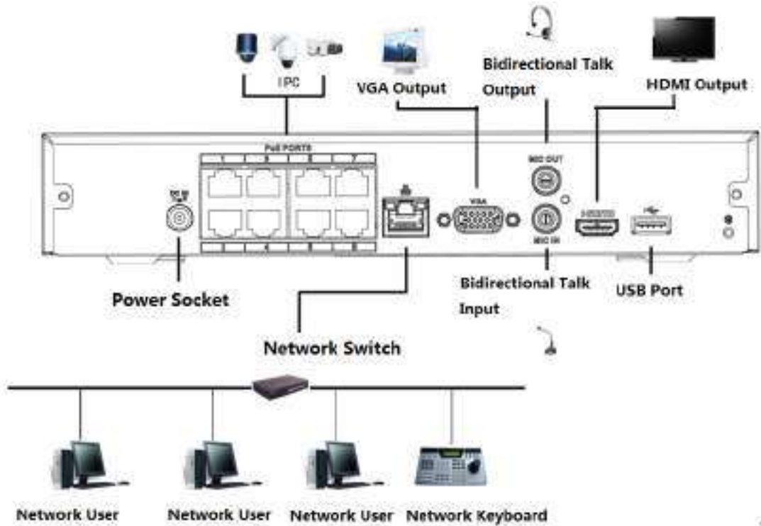
Figura 3-49 Conexiune tipică
