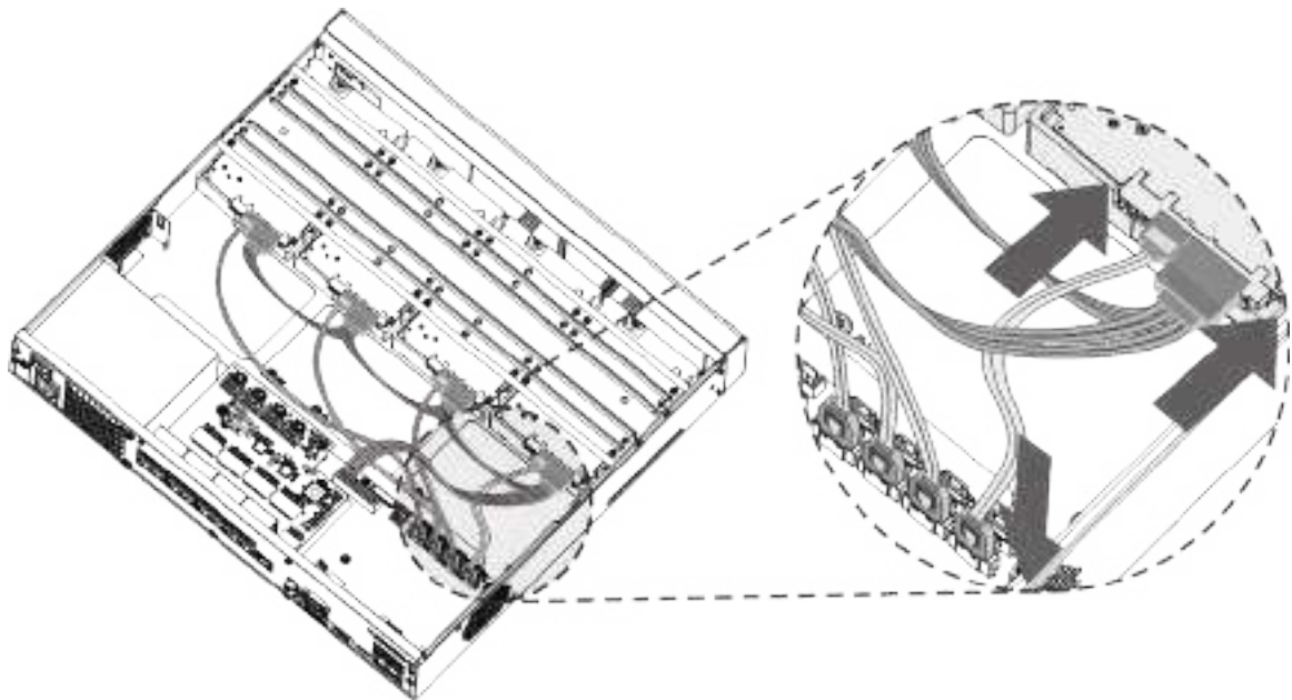
Figura 3-25 Conectați cablurile
