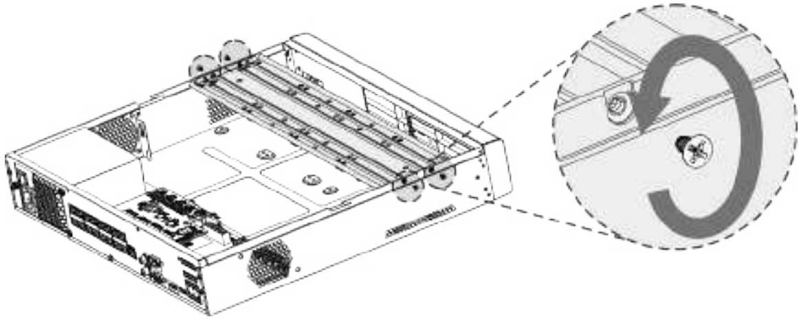
Figura 3-20 Scoateți șuruburile (2U)
