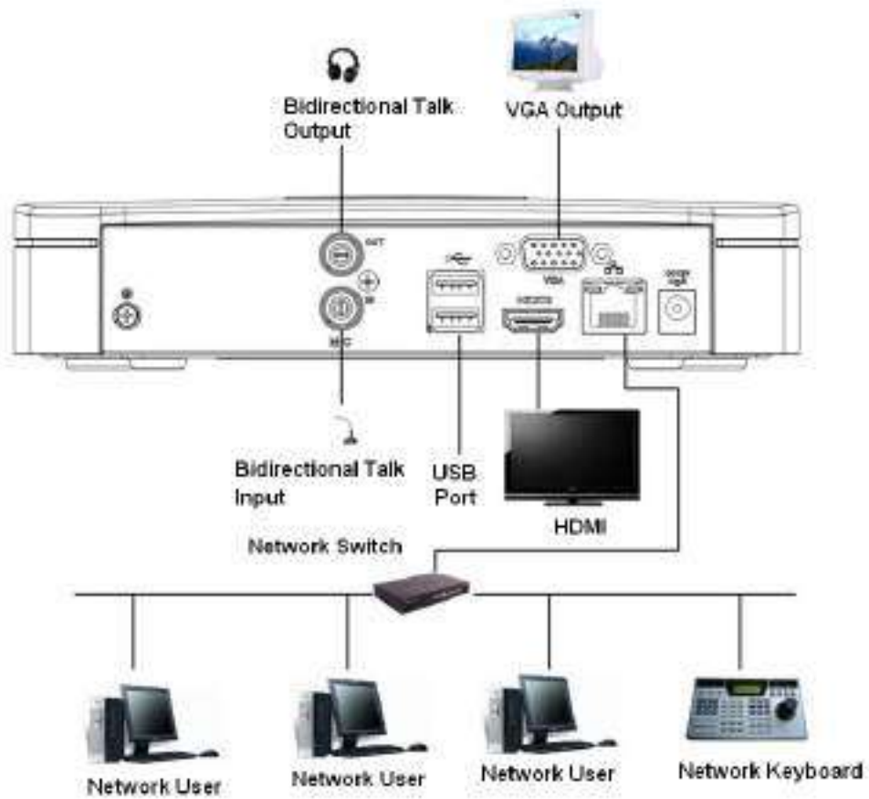
Figura 3-47 Conexiune tipică
