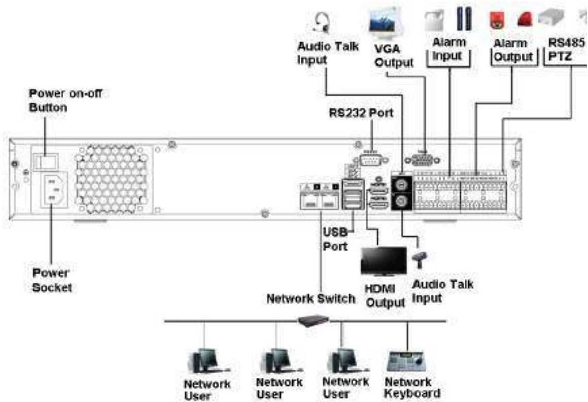
Figura 3-53 Conexiune tipică
