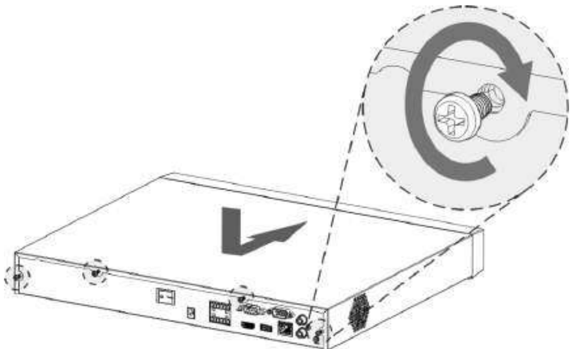
Figura 3-16 Puneți capacul din spate
