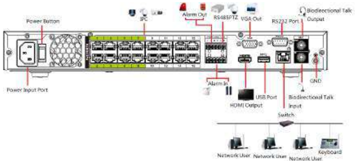
Figura 3-58 Conexiune tipică
