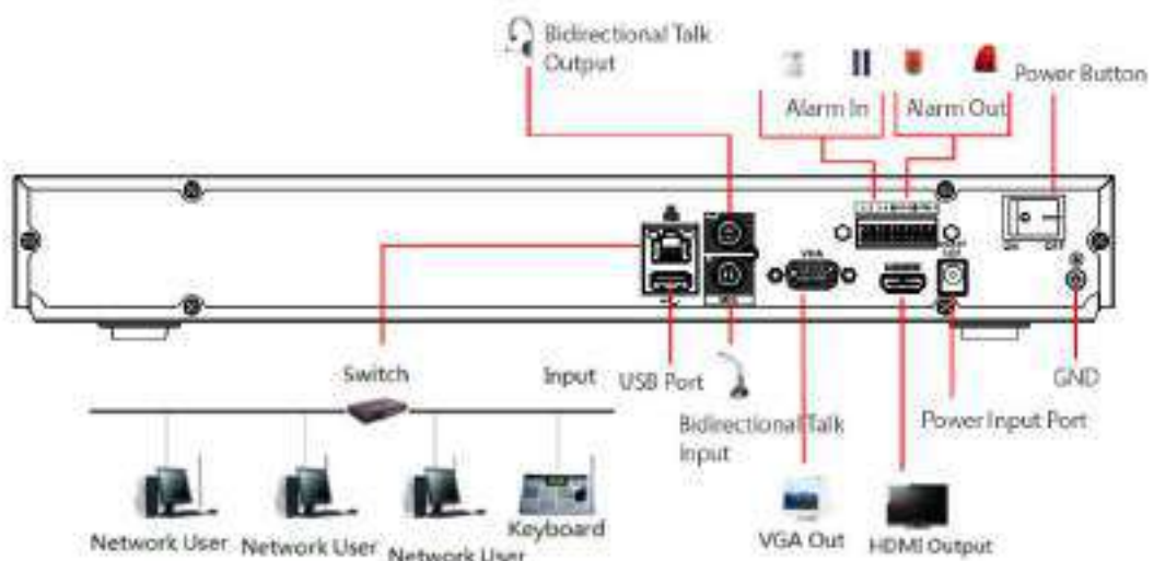
Figura 3-59 Conexiune tipică
