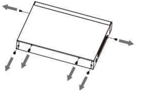
Figura 3-7 Scoateți capacul
