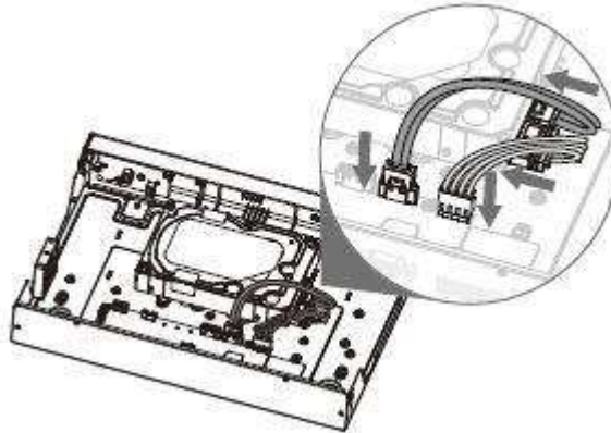
Figura 3-9 Conectați cablurile
