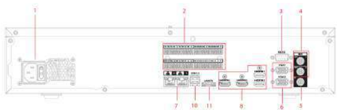
Figura 2-87 Panoul din spate (3)
