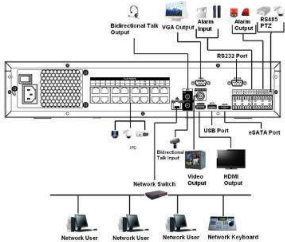
Figura 3-55 Conexiune tipică
