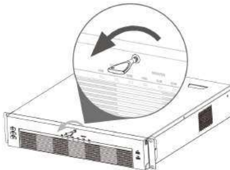
Figura 3-27 Deblocați panoul frontal
