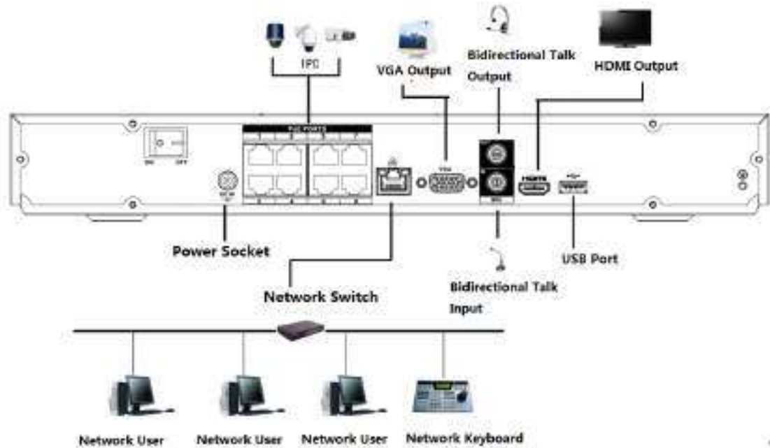
Figura 3-50 Conexiune tipică
