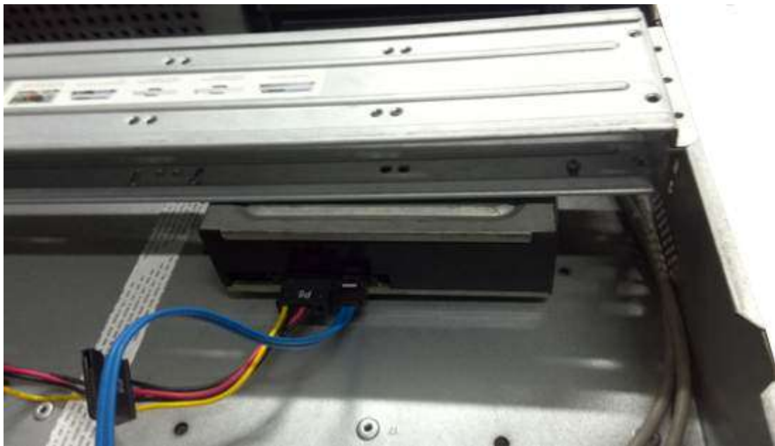
Figura 3-45 Conectați cablurile
