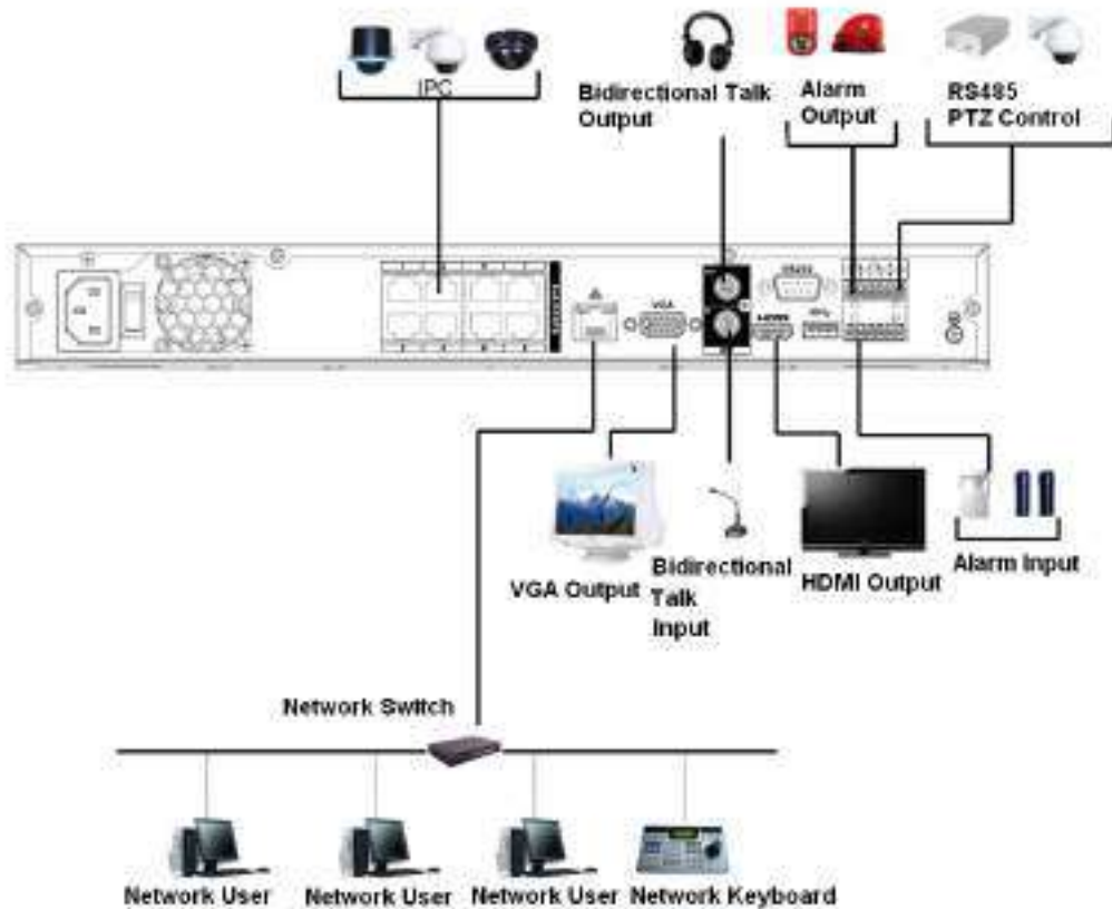
Figura 3-51 Conexiune tipică
