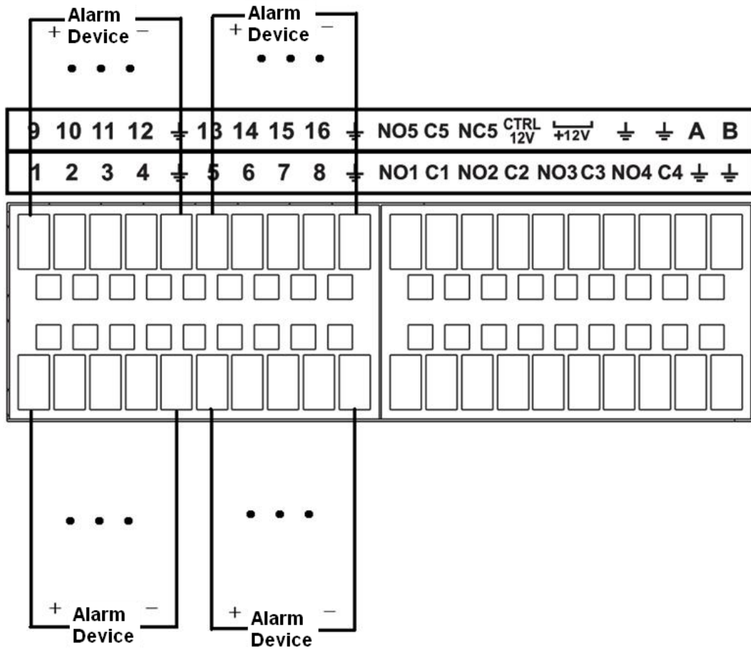
Figura 2-98 Port de intrare alarmă (1)
