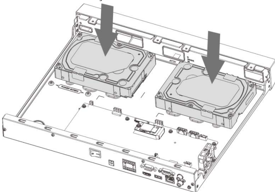
Figura 3-14 Aliniere HDD
