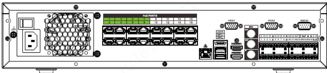
Figura 2-49 Panoul din spate
