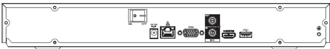
Figura 2-34 Panoul din spate
