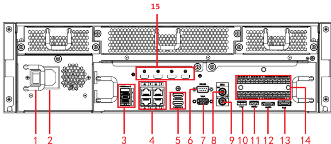
Figura 2-89 Panoul din spate
