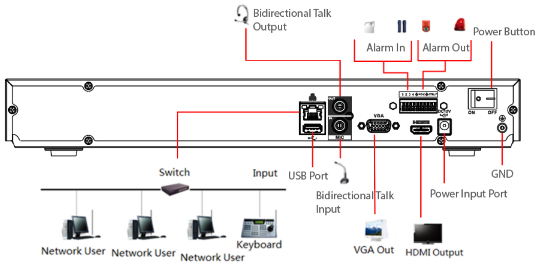
Figura 3-60 Conexiune tipică
