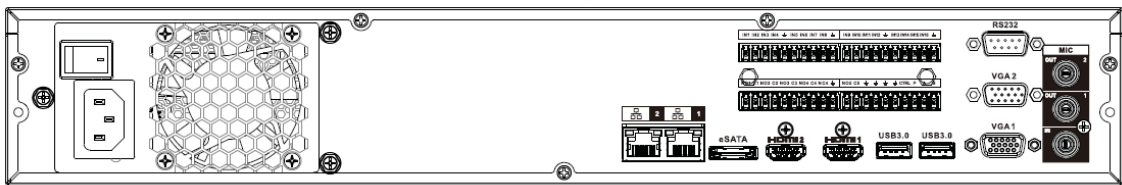
Figura 2-92 Panoul din spate
