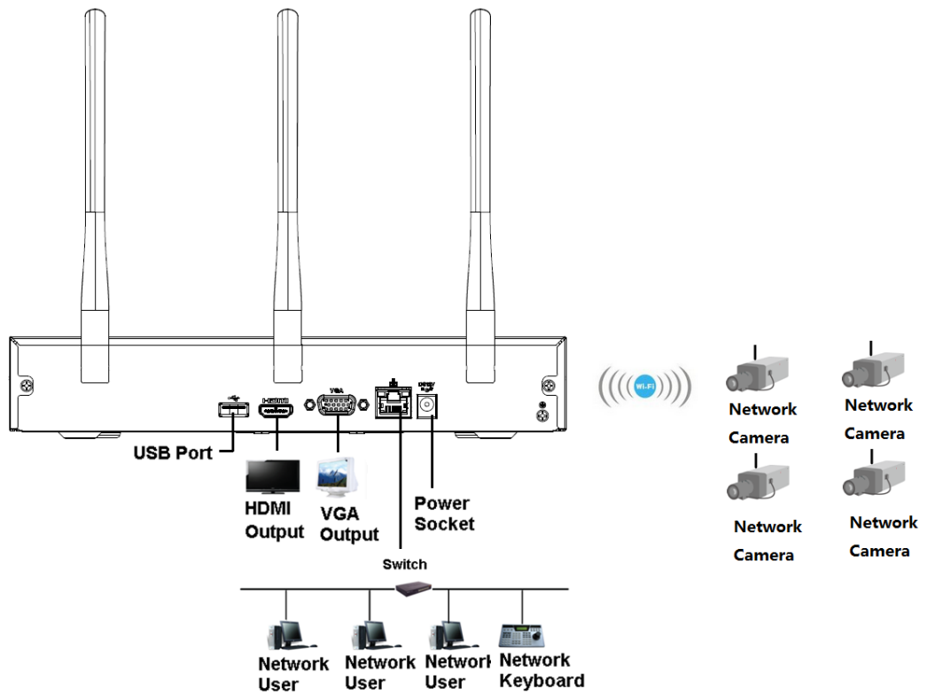
Figura 3-49 Conexiune tipică
