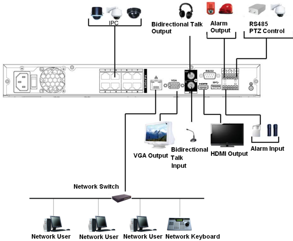
Figura 3-52 Conexiune tipică
