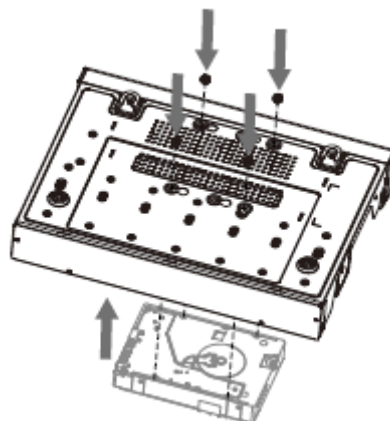
Figura 3-9 Aliniați HDD
