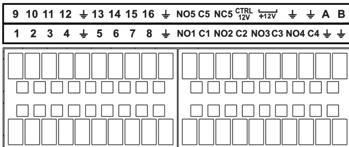
Figura 2-97 Port de alarmă
