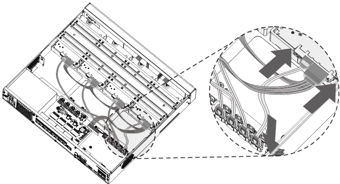
Figura 3-26 Conectați cablurile
