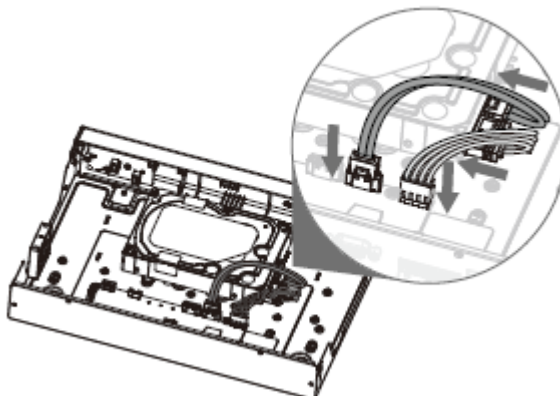
Figura 3-10 Conectați cablurile
