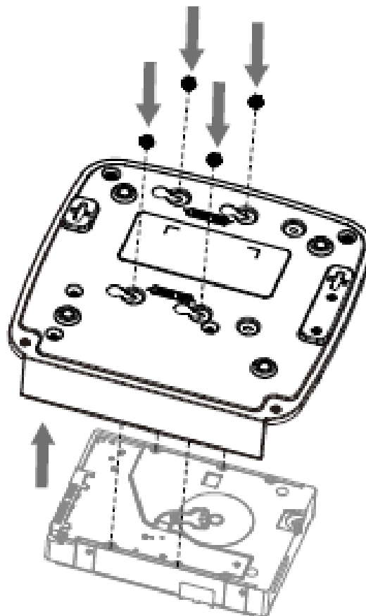
Figura 3-4 Fixați șuruburile
