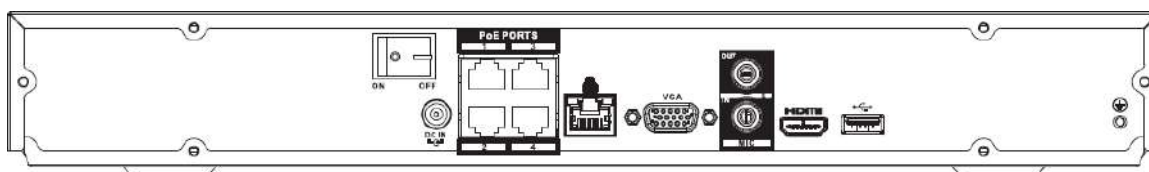
Figura 2-82 Panoul din spate
