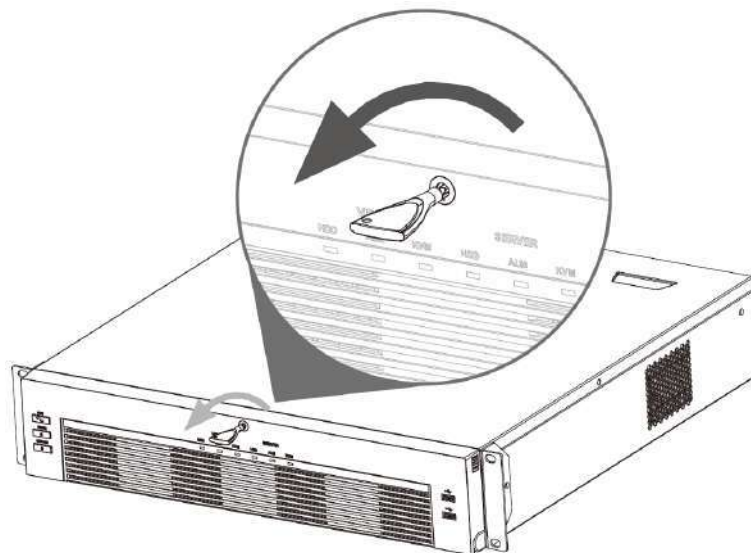
Figura 3-30 Fixați HDD
