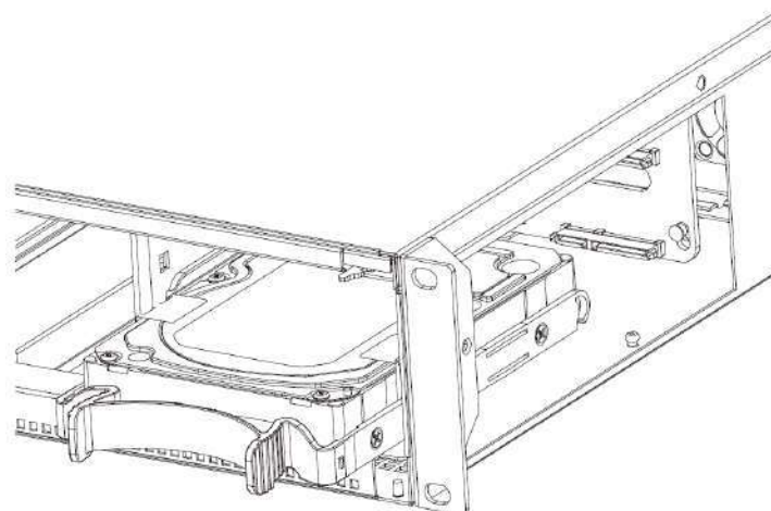
Figura 3-31 Deblocarea panoului frontal
