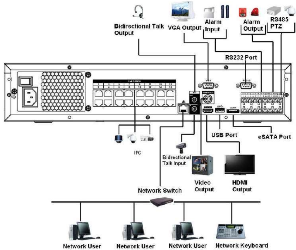
Figura 3-56 Conexiune tipică
