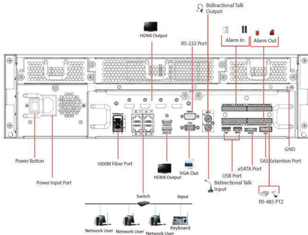
Figura 3-62 Conexiune tipică
