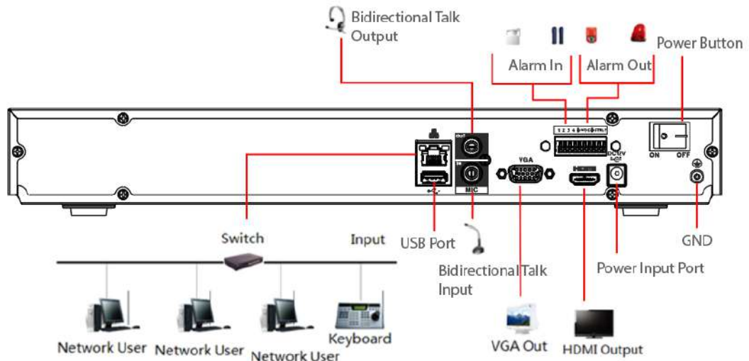
Figura 3-60 Conexiune tipică
