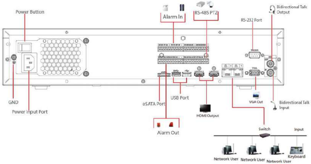
Figura 3-61 Conexiune tipică
