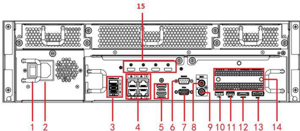
Figura 2-104 Panoul din spate
