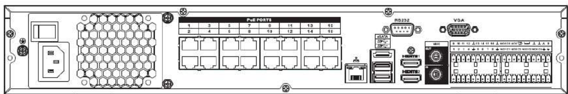
Figura 2-58 Panoul din spate
