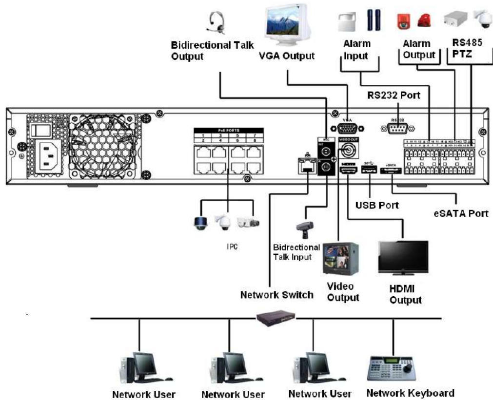
Figura 3-55 Conexiune tipică
