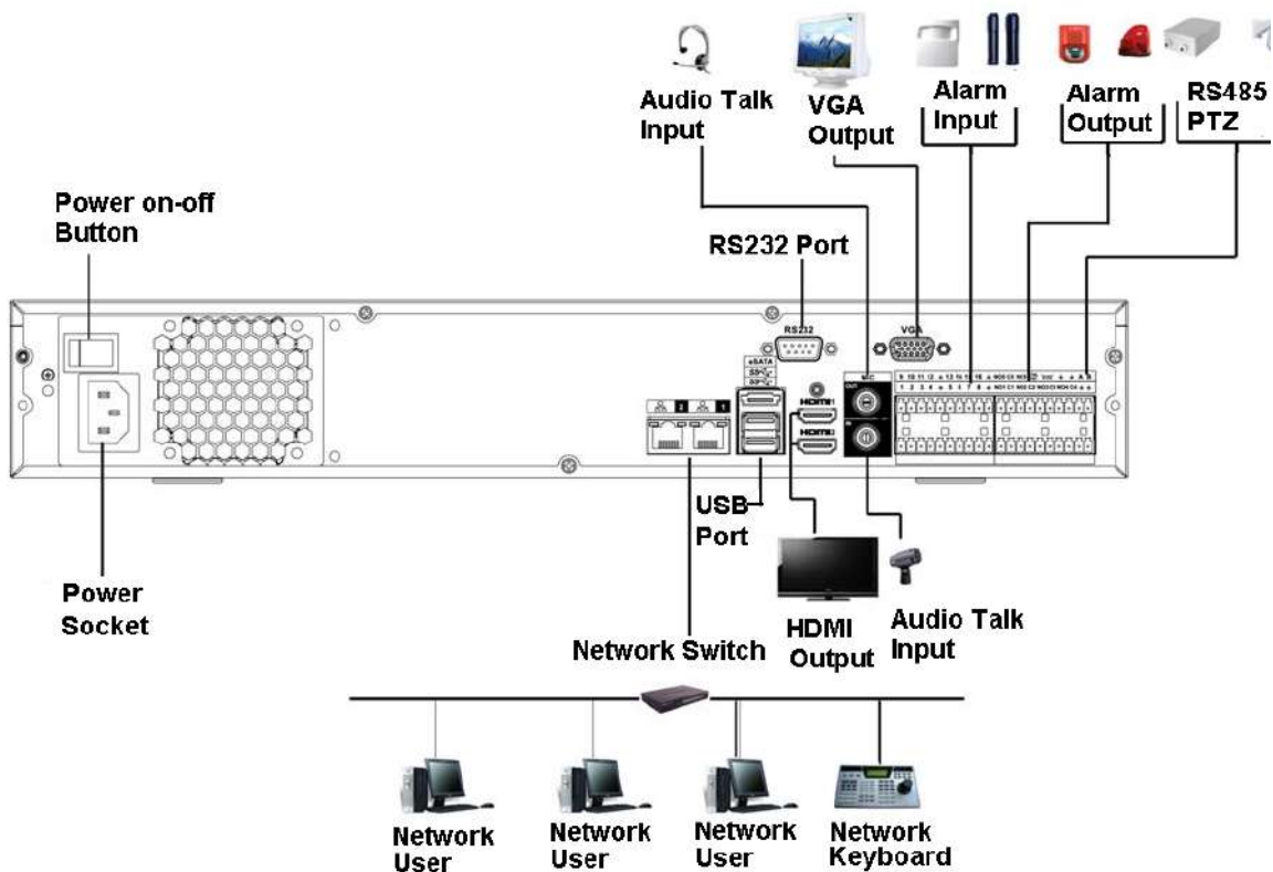
Figura 3-54 Conexiune tipică
