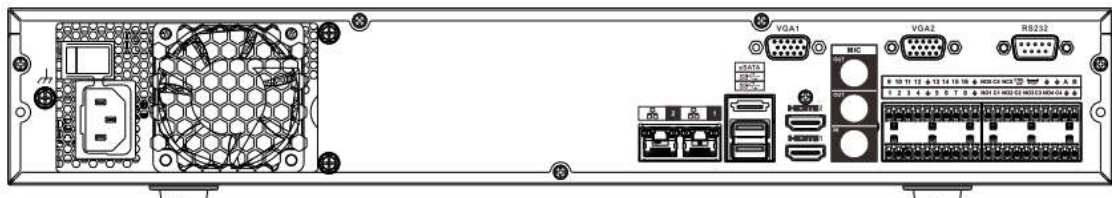
Figura 2-57 Panoul din spate
