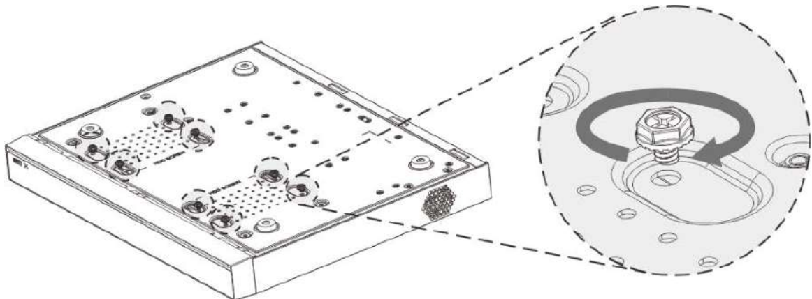
Figura 3-15 Fixați șuruburile
