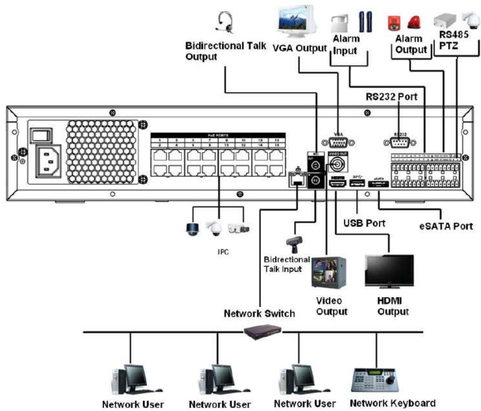
Figura 3-56 Conexiune tipică
