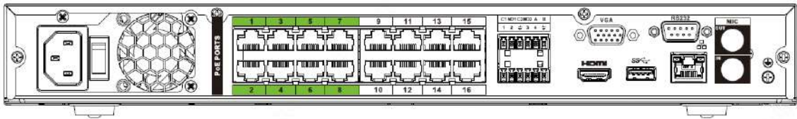
Figura 2-50 Panoul din spate
