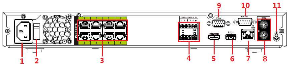
Figura 2-98 Panoul din spate
