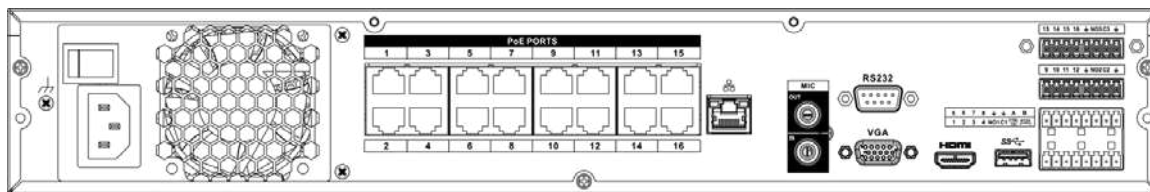
Figura 2-70 Panoul din spate
