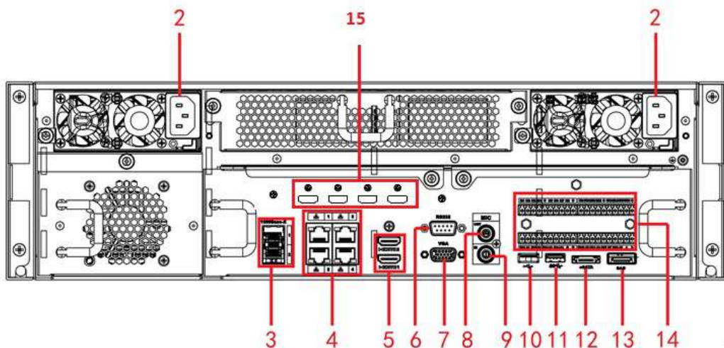
Figura 2-105 Panoul din spate
