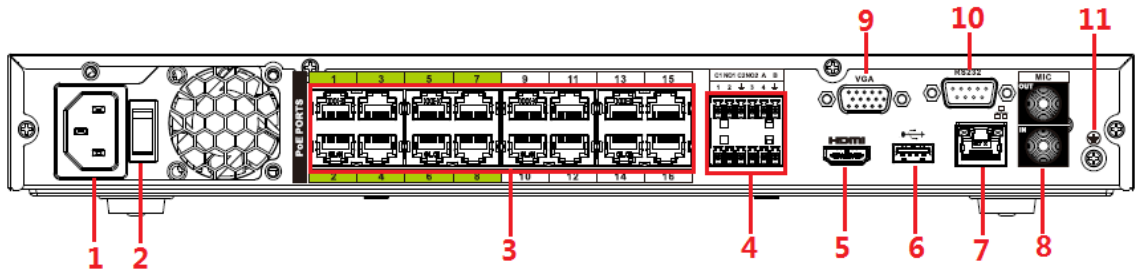
Figura 2-97 Panoul din spate
