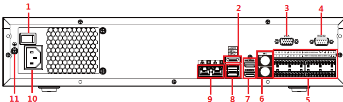
Figura 2-94 Panoul din spate
