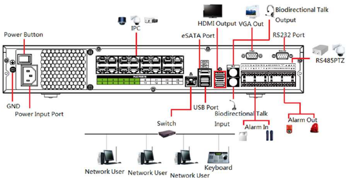
Figura 3-58 Conexiune tipică
