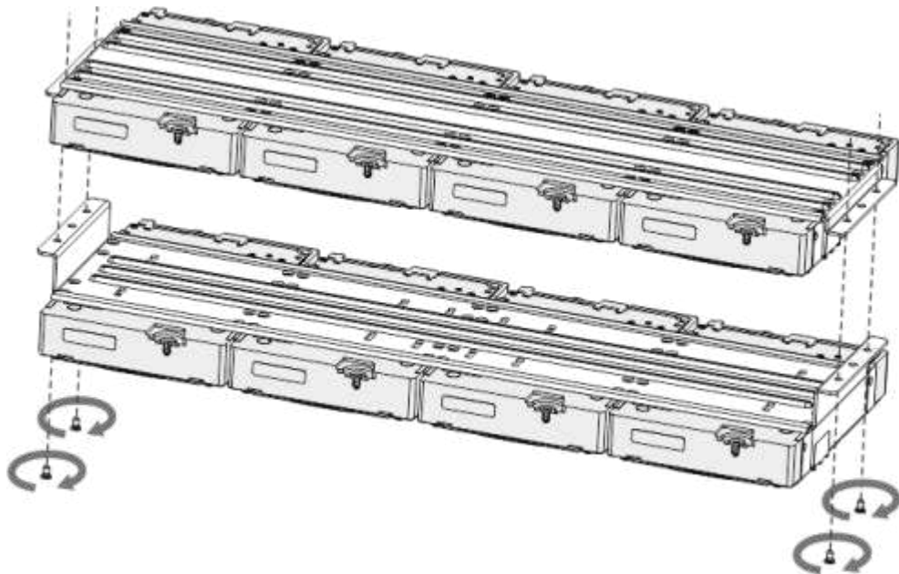
Figura 3-24 Blocare paranteze
