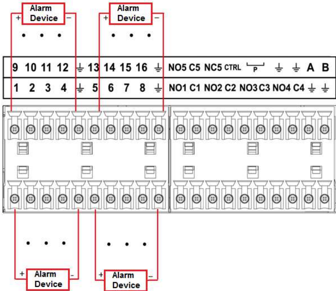
Figura 2-119 Port de intrare alarmă (2)
