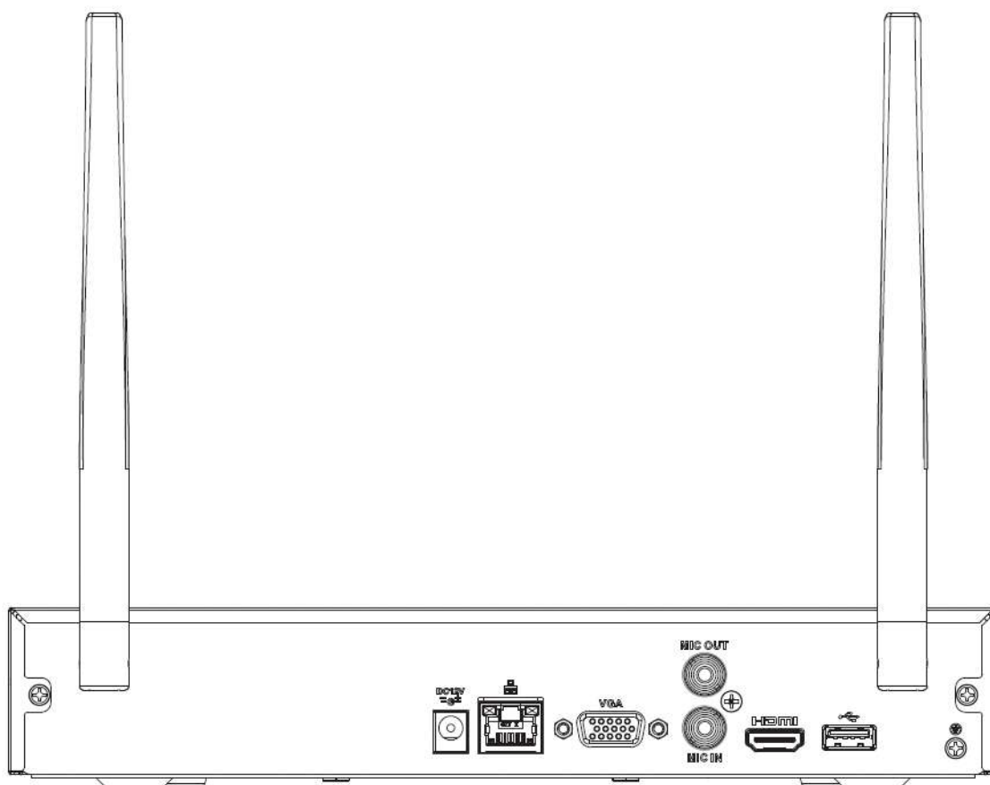
Figura 2-109 Panoul din spate
