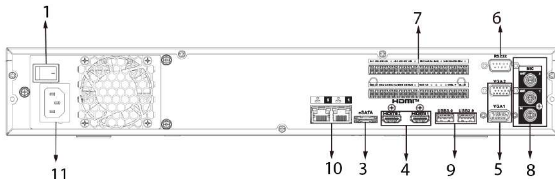
Figura 2-96 Panoul din spate
