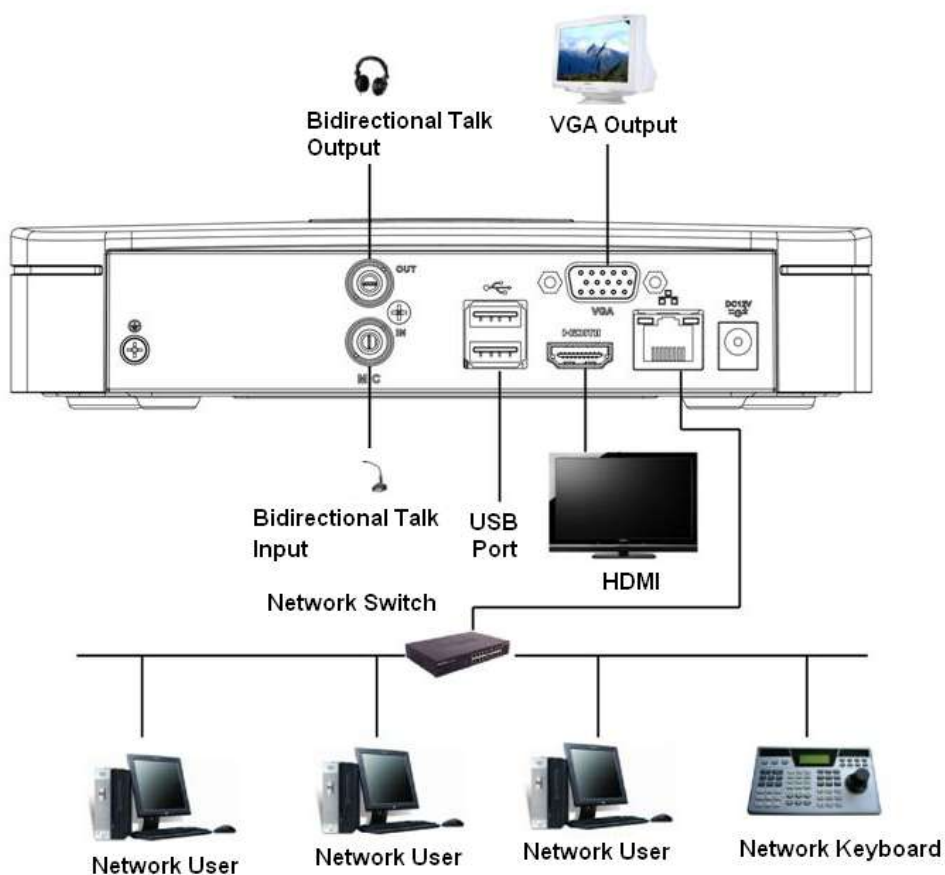
Figura 3-48 Conexiune tipică
