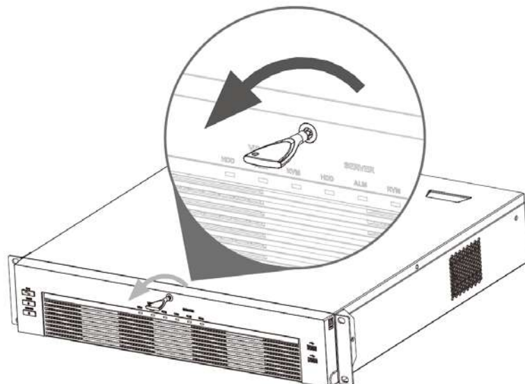
Figura 3-30 Fixați HDD
