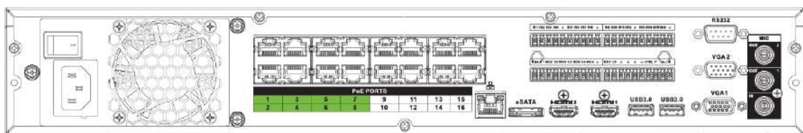
Figura 2-112 Panoul din spate
