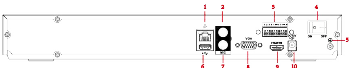
Figura 2-92 Panoul din spate
