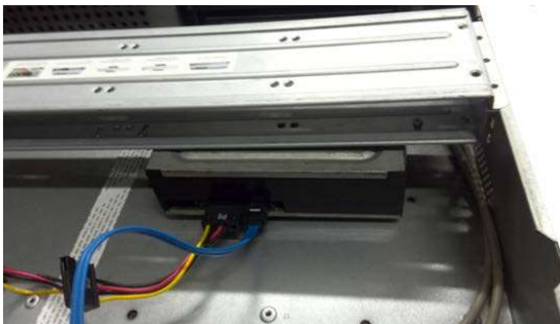
Figura 3-46 Conectați cablurile
