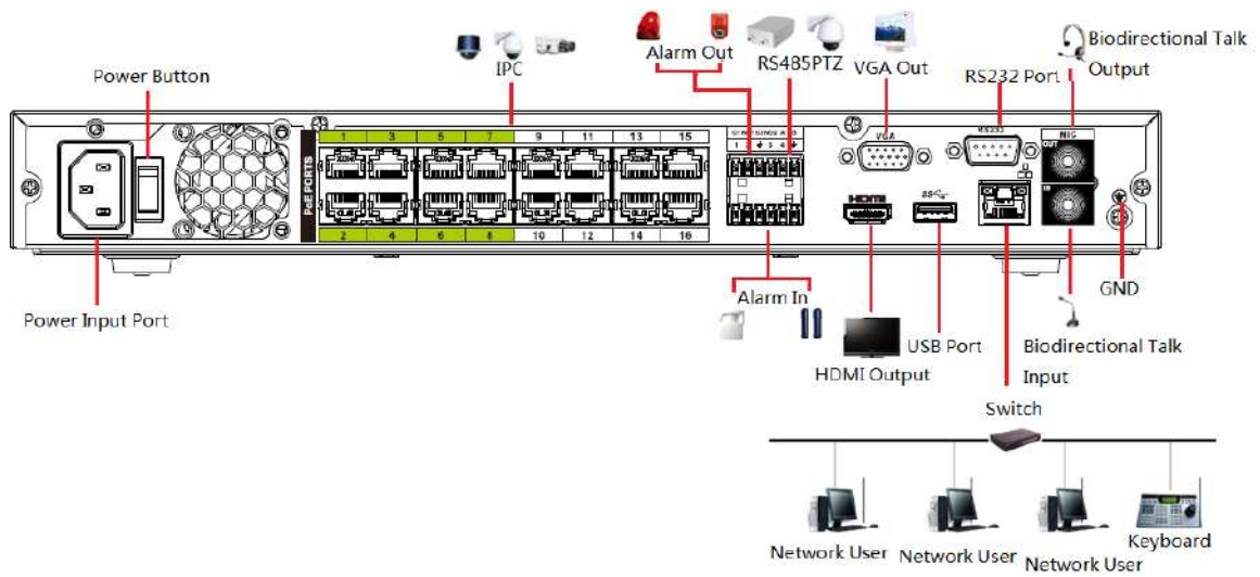
Figura 3-59 Conexiune tipică
