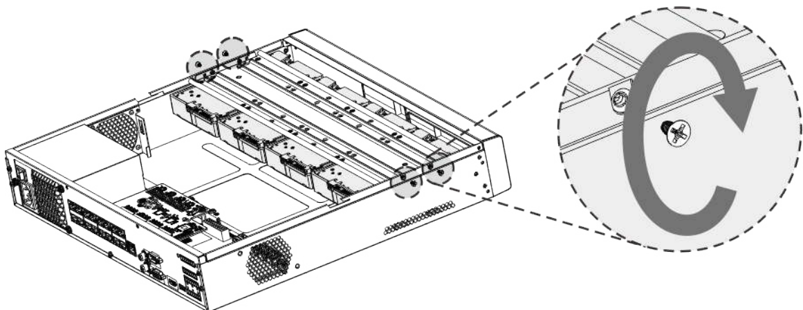
Figura 3-25 Fixați șuruburile
