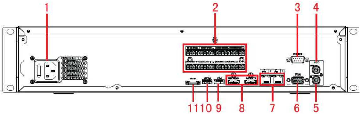
Figura 2-102 Panoul din spate (3)
