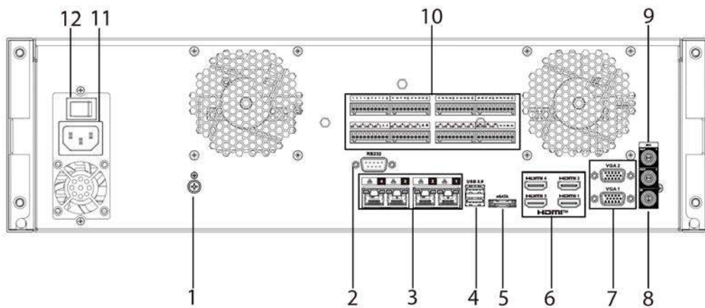
Figura 2-106 Panoul din spate
