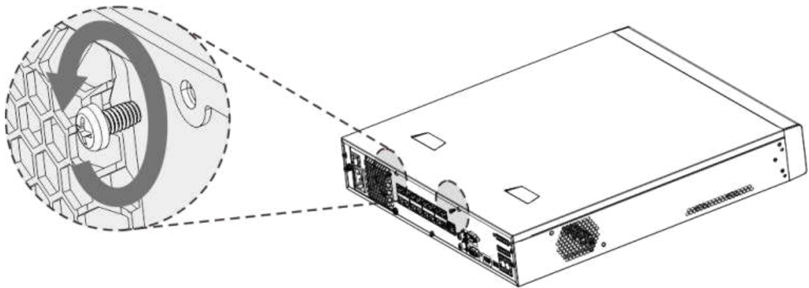
Figura 3-18 Scoateți șuruburile
