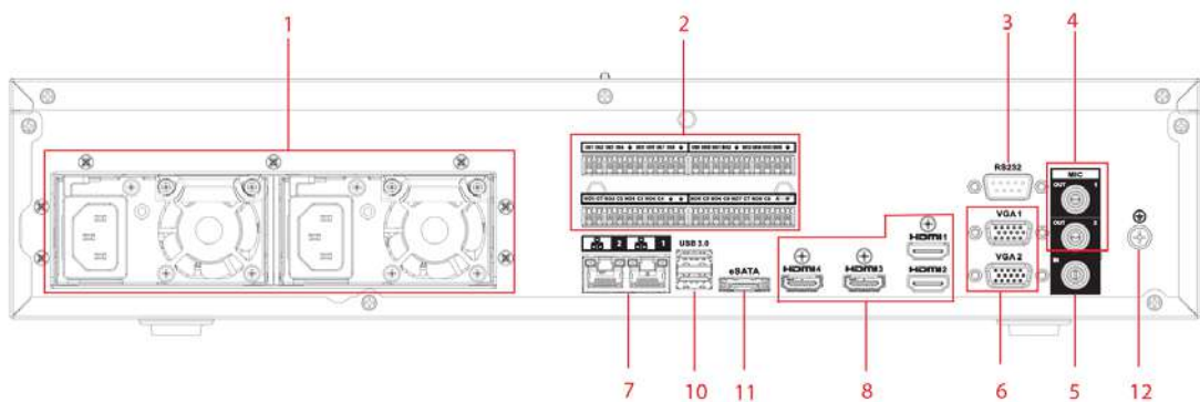
Figura 2-103 Panoul din spate (4)
