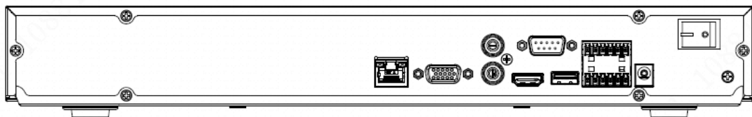
Figura 2-46 Panoul din spate
