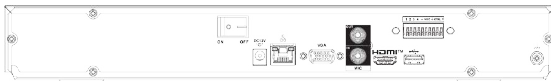
Figura 2-65 Panoul din spate
