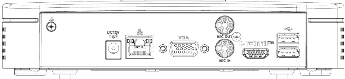
Figura 2-33 Panoul din spate
