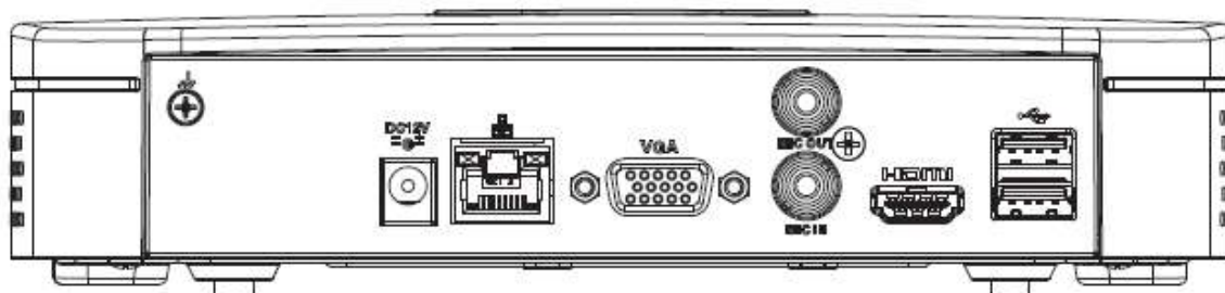
Figura 2-62 Panoul din spate
