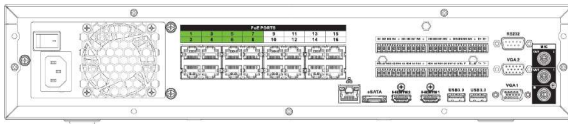
Figura 2-113 Panoul din spate
