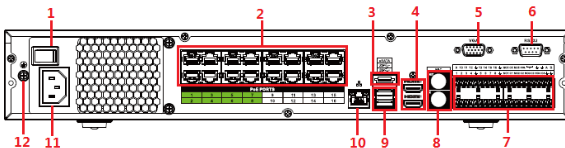
Figura 2-96 Panoul din spate
