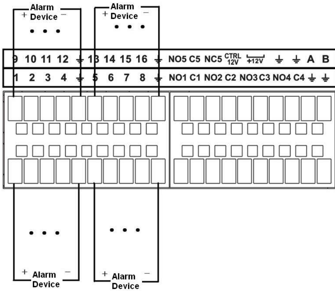
Figura 2-118 Port de intrare alarmă (1)
