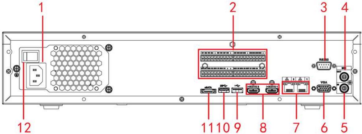
Figura 2-100 Panoul din spate (1)
