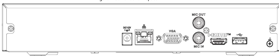
Figura 2-36 Panoul din spate
