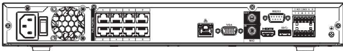
Figura 2-47 Panoul din spate
