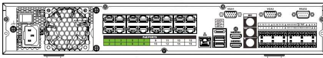
Figura 2-60 Panoul din spate
