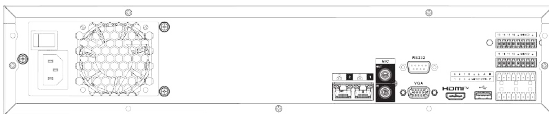
Figura 2-73 Panoul din spate
