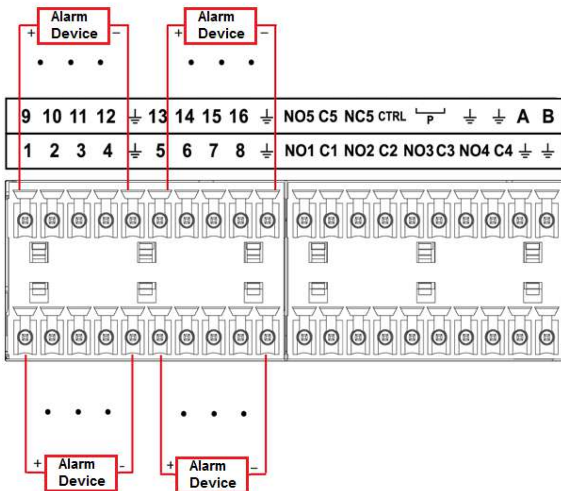
Figura 2-117 Port de intrare alarmă (2)
