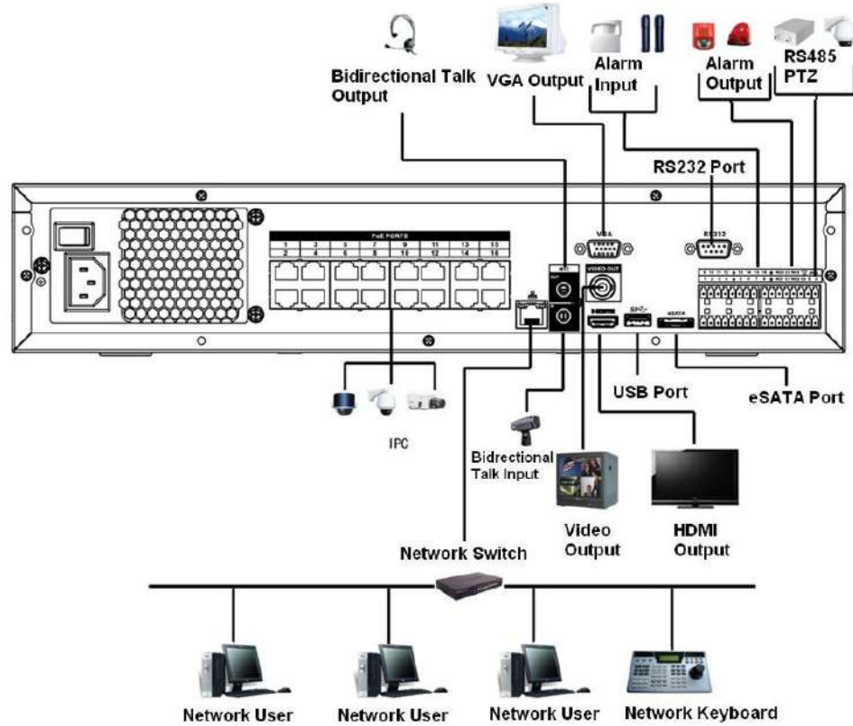
Figura 3-56 Conexiune tipică
