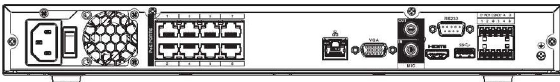
Figura 2-48 Panoul din spate
