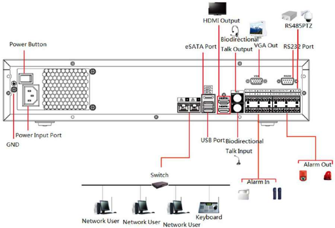
Figura 3-57 Conexiune tipică
