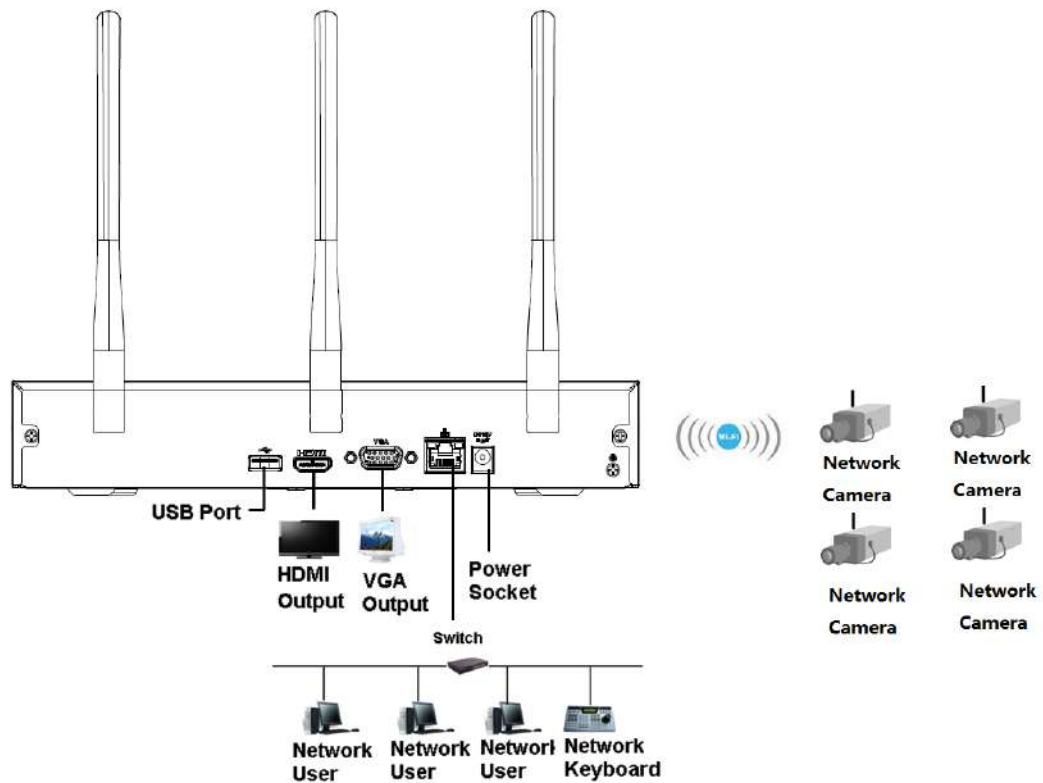
Figura 3-49 Conexiune tipică
