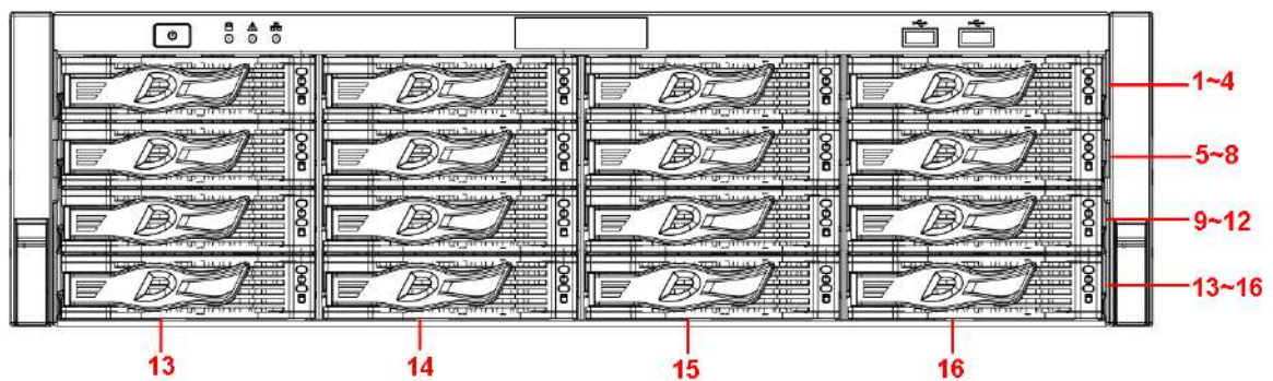
Figura 2-31 Panoul frontal
