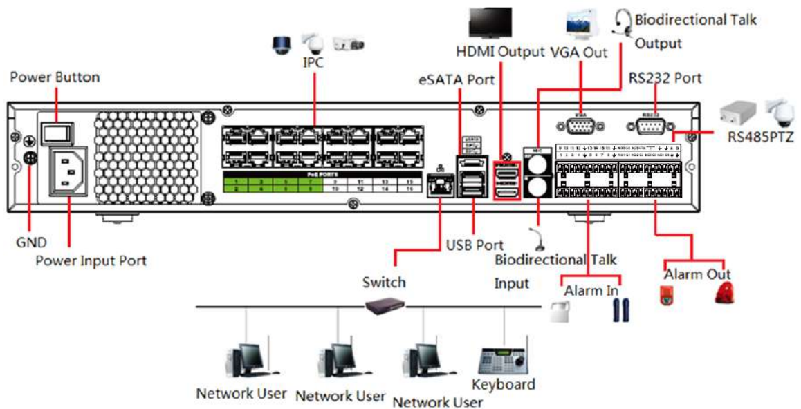
Figura 3-58 Conexiune tipică
