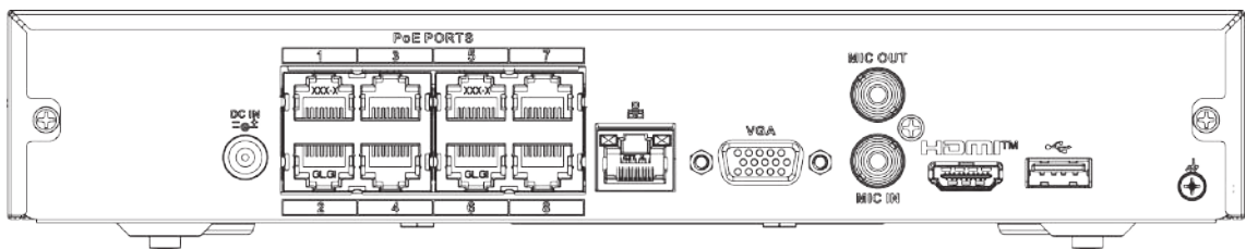
Figura 2-39 Panoul din spate
