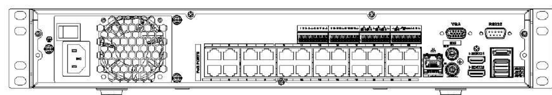
Figura 2-60 Panoul din spate
