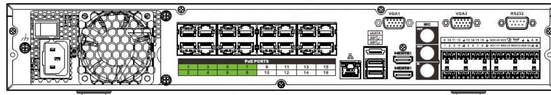
Figura 2-61 Panoul din spate
