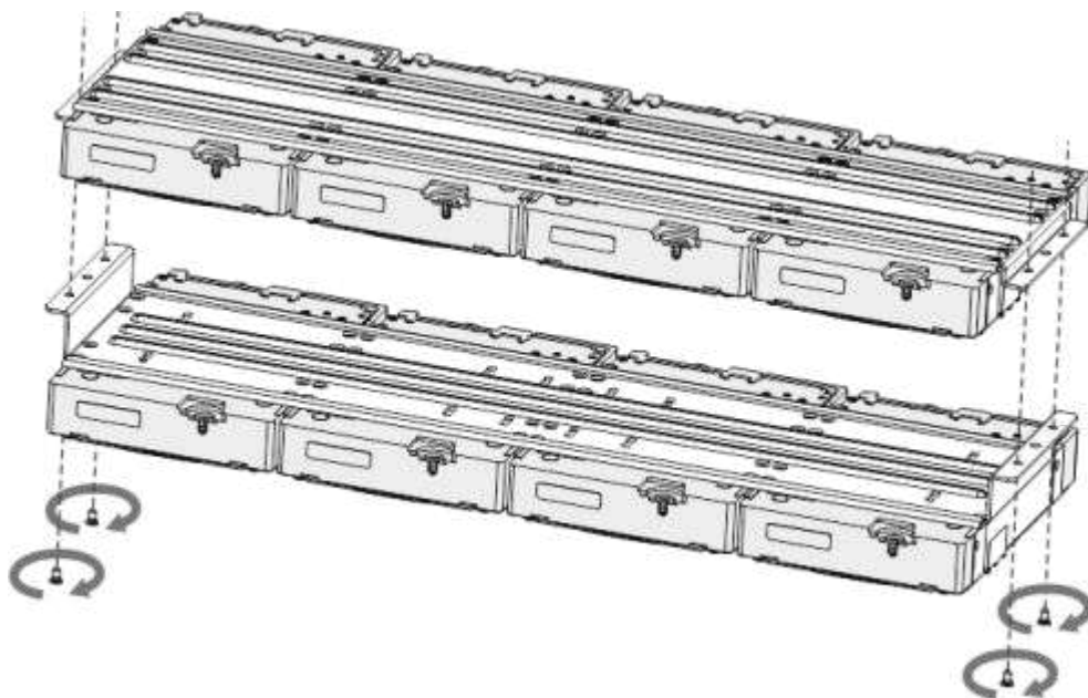
Figura 3-24 Blocare paranteze
