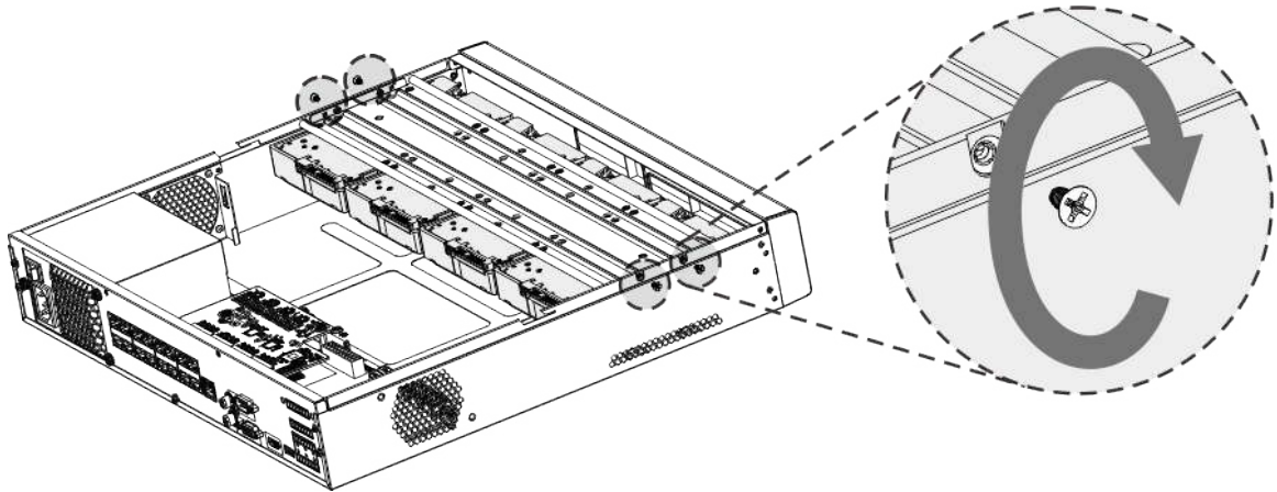
Figura 3-25 Fixați șuruburile
