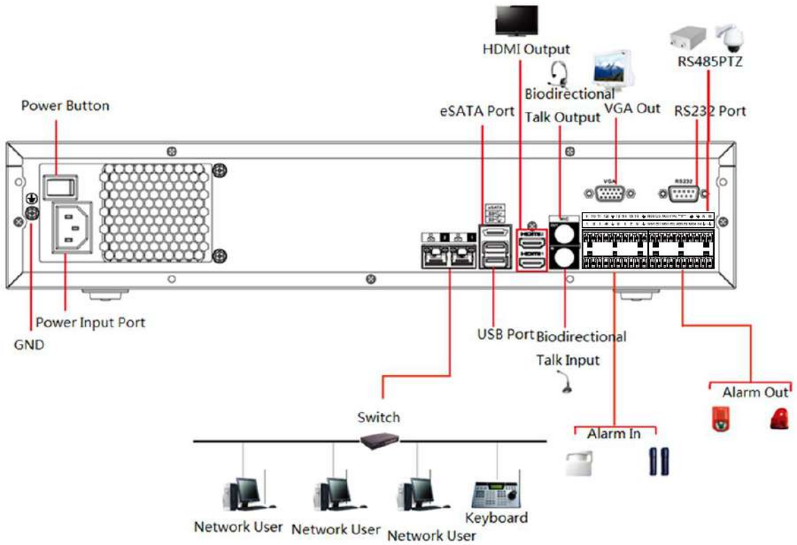
Figura 3-57 Conexiune tipică
