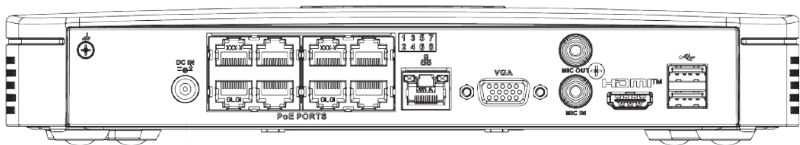
Figura 2-36 Panoul din spate
