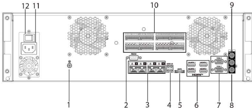
Figura 2-104 Panoul din spate
