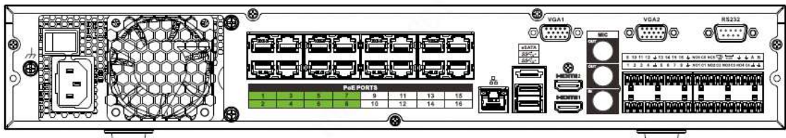
Figura 2-61 Panoul din spate
