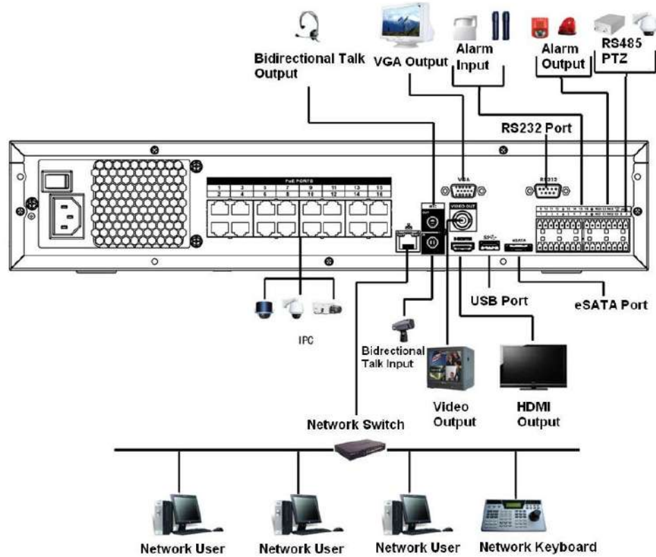
Figura 3-56 Conexiune tipică
