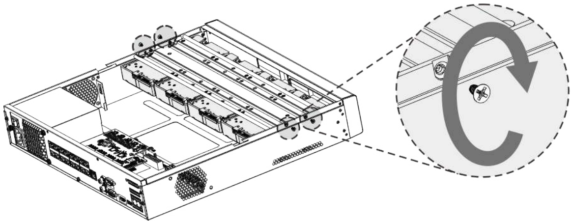
Figura 3-25 Fixați șuruburile
