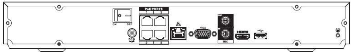
Figura 2-41 Panoul din spate
