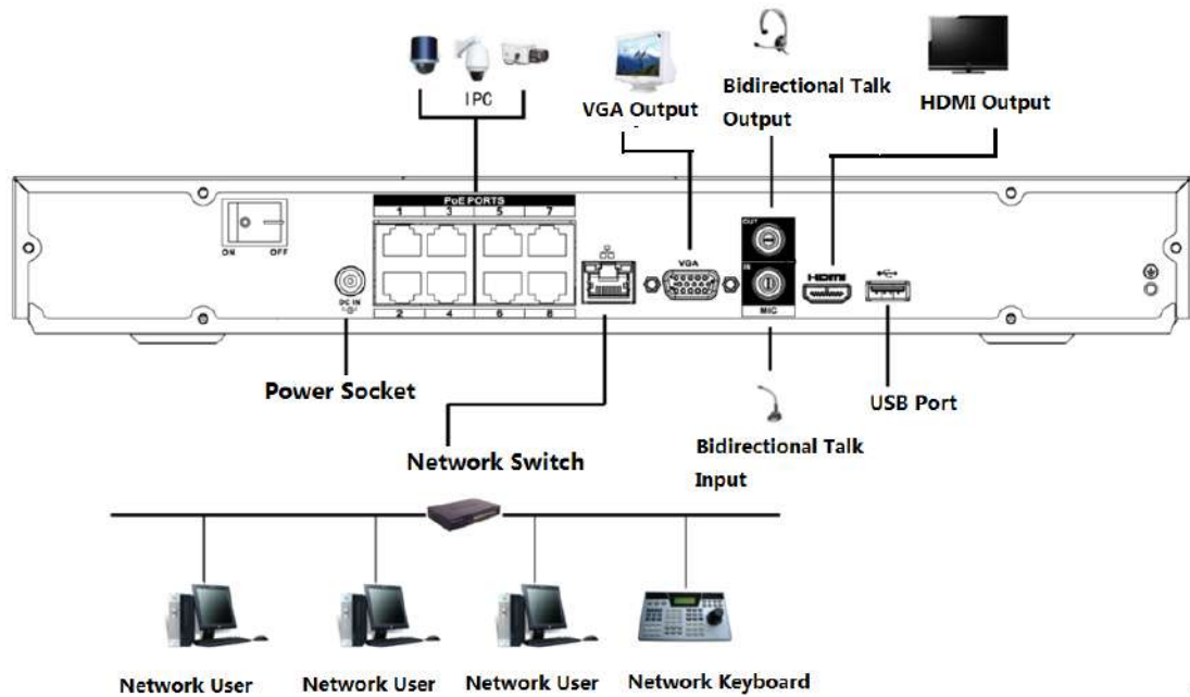
Figura 3-51 Conexiune tipică
