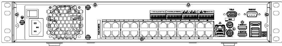
Figura 2-60 Panoul din spate
