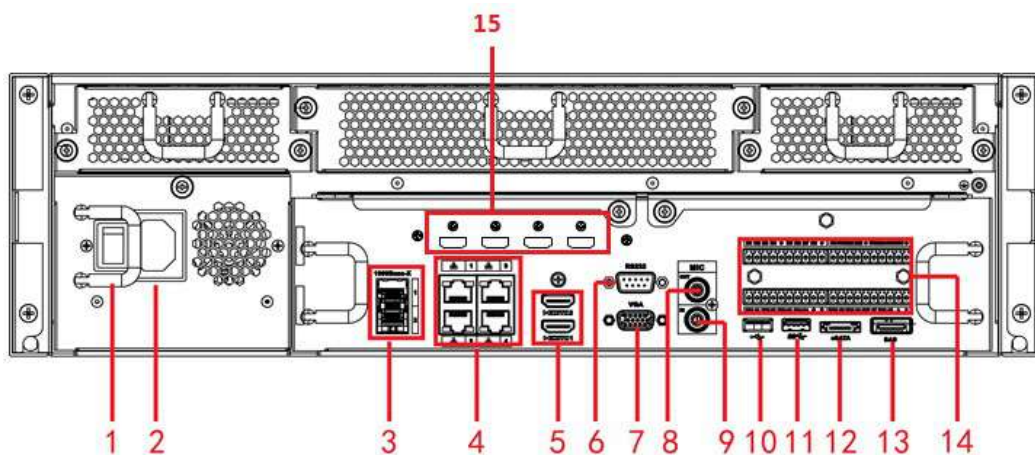
Figura 2-102 Panoul din spate
