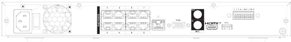
Figura 2-68 Panoul din spate
