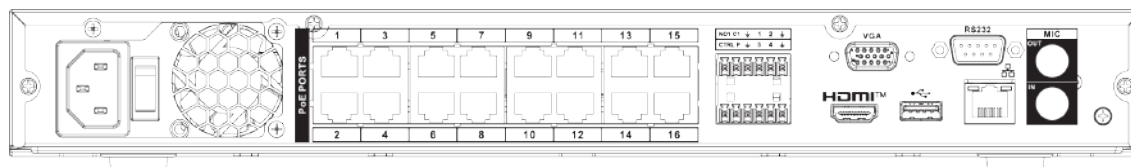
Figura 2-49 Panoul din spate
