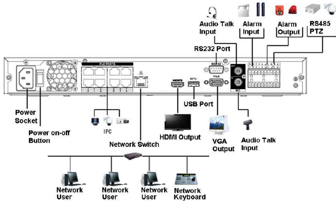
Figura 3-53 Conexiune tipică
