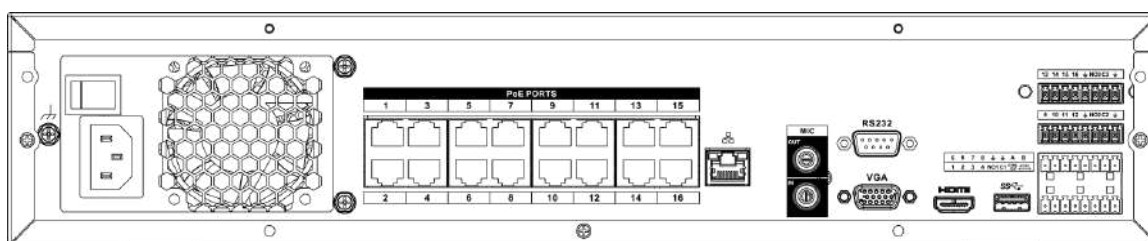
Figura 2-74 Panoul din spate
