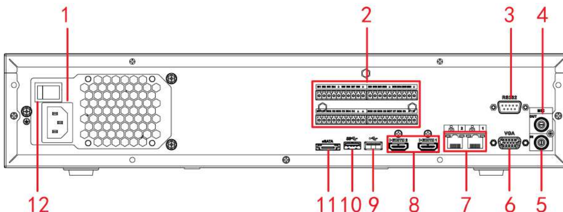
Figura 2-98 Panoul din spate (1)
