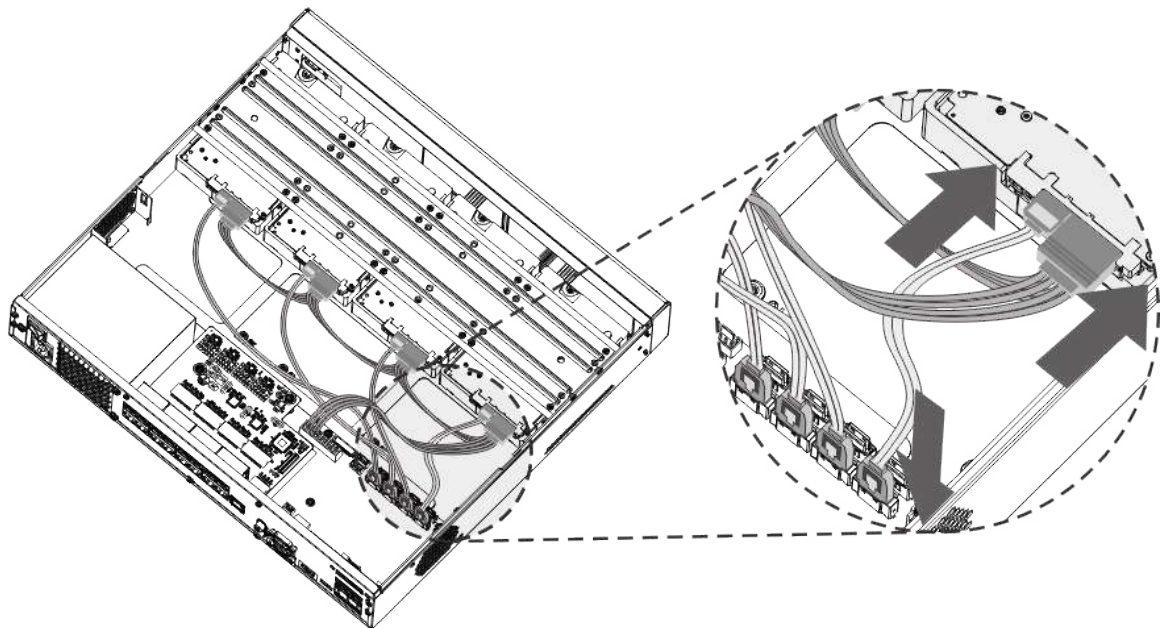
Figura 3-26 Conectați cablurile
