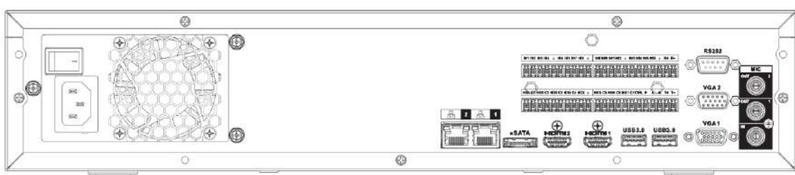
Figura 2-109 Panoul din spate
