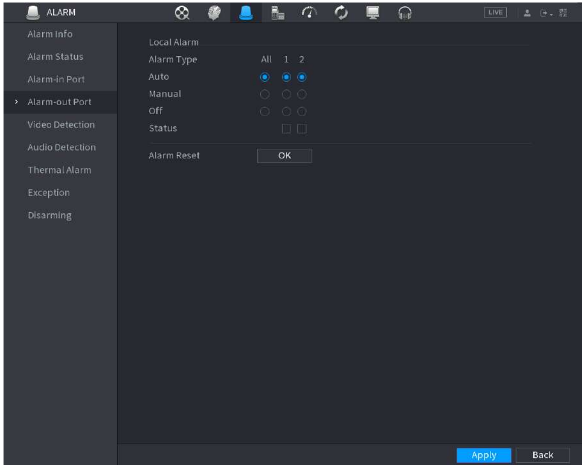
Figura 5-208 Port de ieșire alarmă
