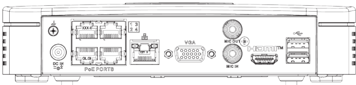
Figura 2-81 Panoul din spate
