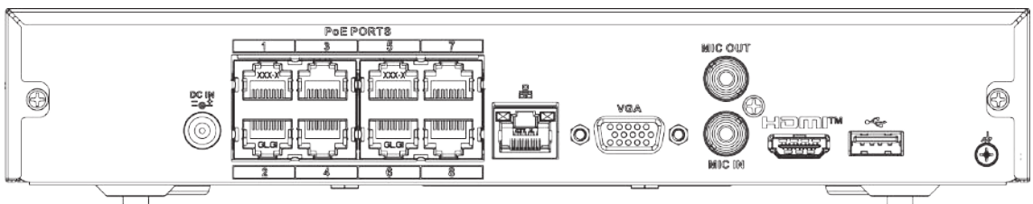
Figura 2-39 Panoul din spate
