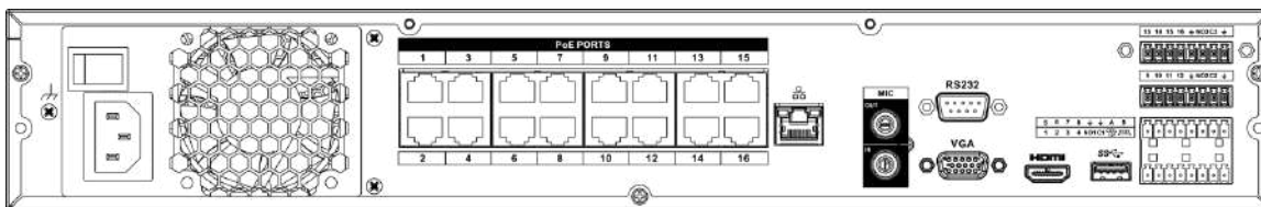
Figura 2-71 Panoul din spate
