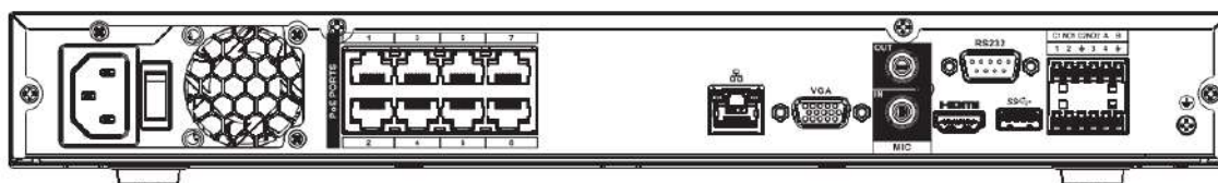
Figura 2-48 Panoul din spate
