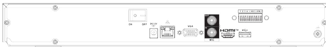
Figura 2-66 Panoul din spate
