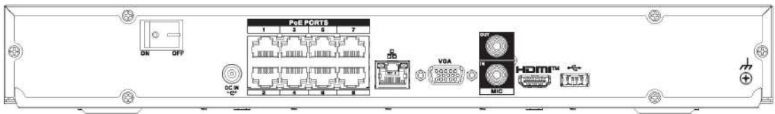
Figura 2-45 Panoul din spate
