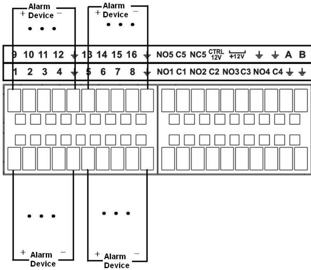
Figura 2-116 Port de intrare alarmă (1)
