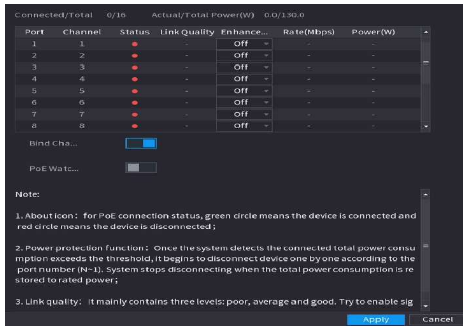
Figura 5-76 PoE
