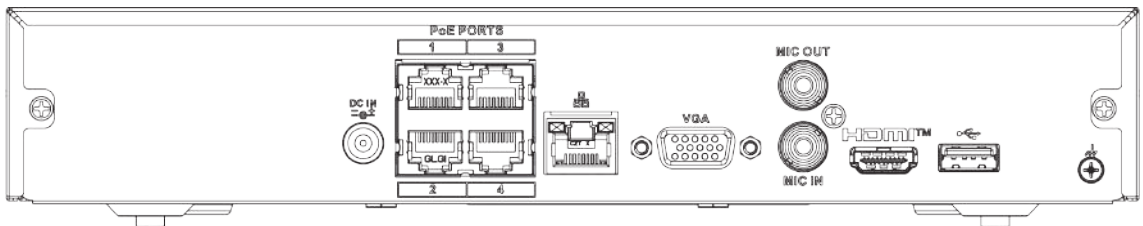
Figura 2-38 Panoul din spate
