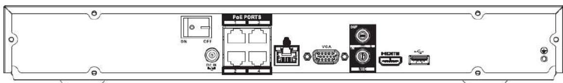
Figura 2-82 Panoul din spate
