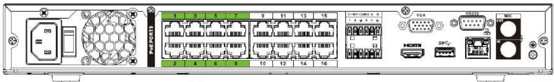
Figura 2-51 Panoul din spate
