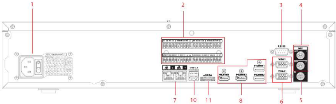
Figura 2-100 Panoul din spate (3)
