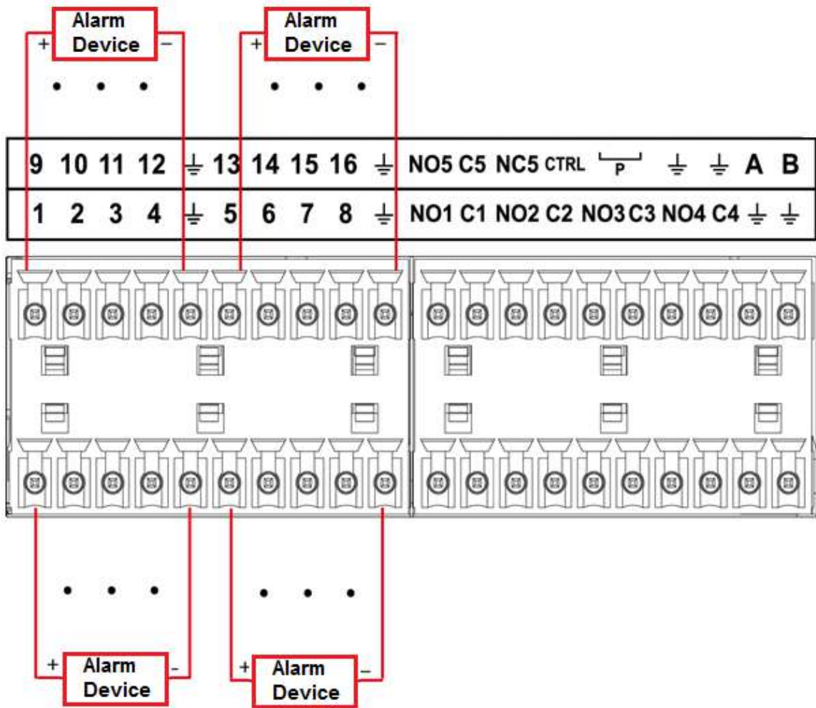
Figura 2-117 Port de intrare alarmă (2)
