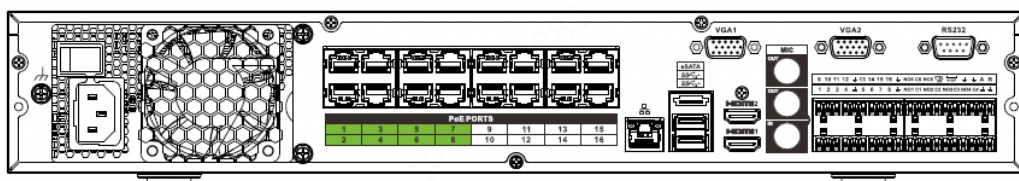
Figura 2-42 Panoul din spate
