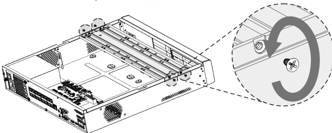
Figura 3-21 Scoateți șuruburile (2U)
