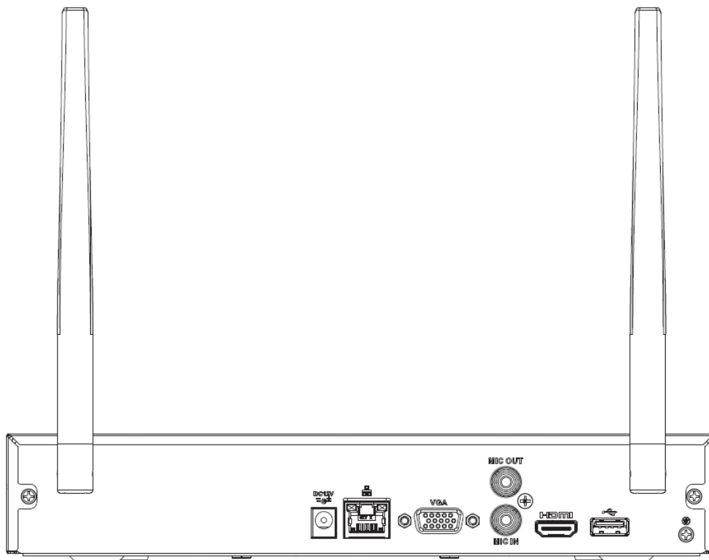
Figura 2-80 Panoul din spate
