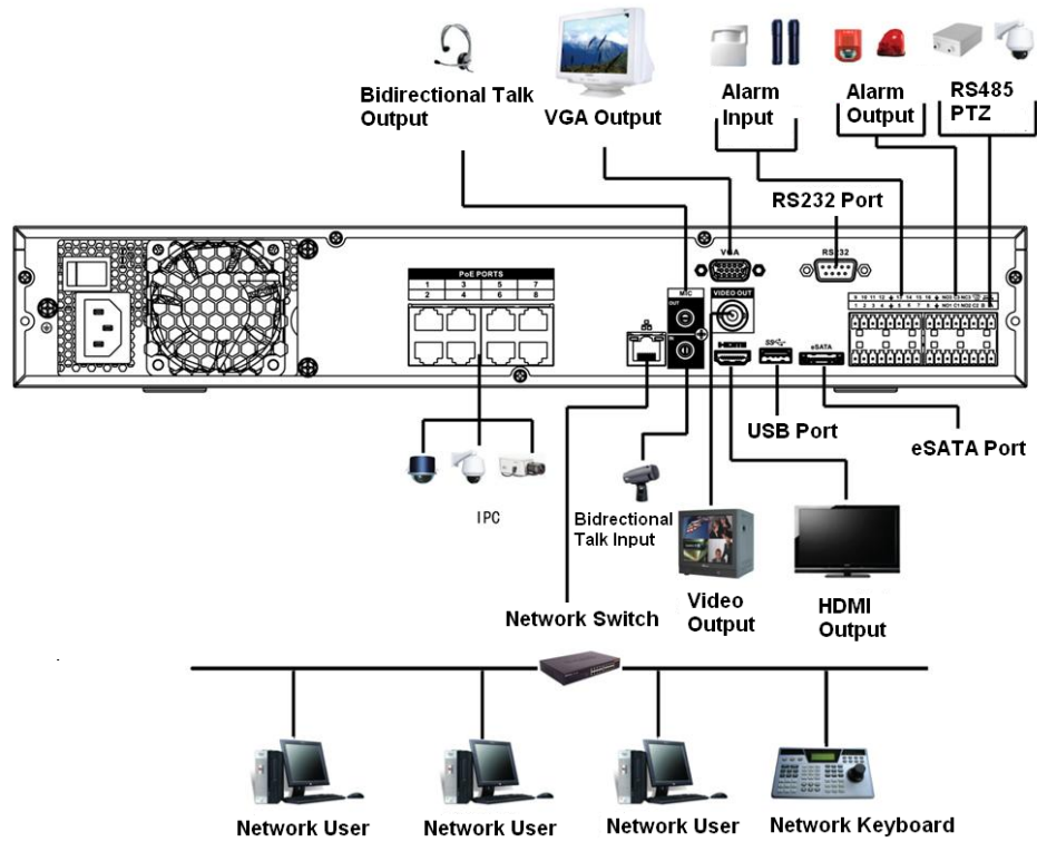
Figura 3-55 Conexiune tipică
