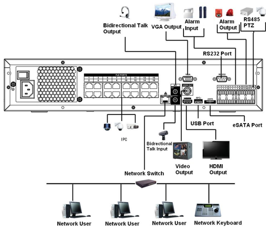
Figura 3-56 Conexiune tipică
