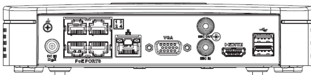
Figura 2-26 Panoul din spate
