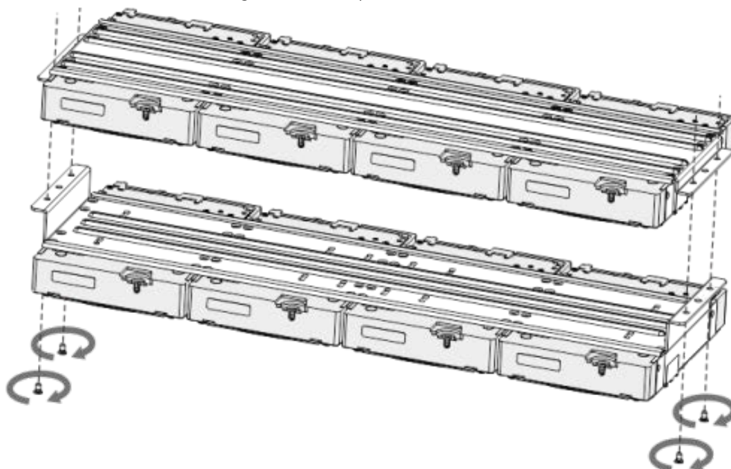
Figura 3-24 Blocare paranteze
