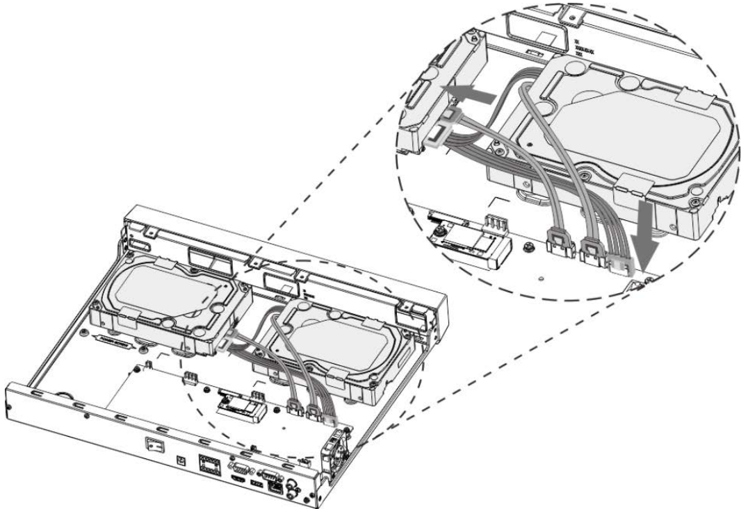
Figura 3-16 Conectați cablurile
