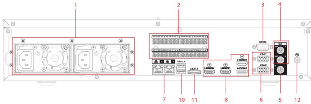
Figura 2-77 Panoul din spate (4)
