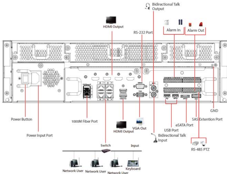
Figura 3-62 Conexiune tipică
