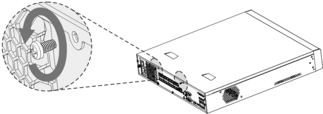
Figura 3-18 Scoateți șuruburile
