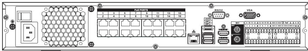
Figura 2-40 Panoul din spate
