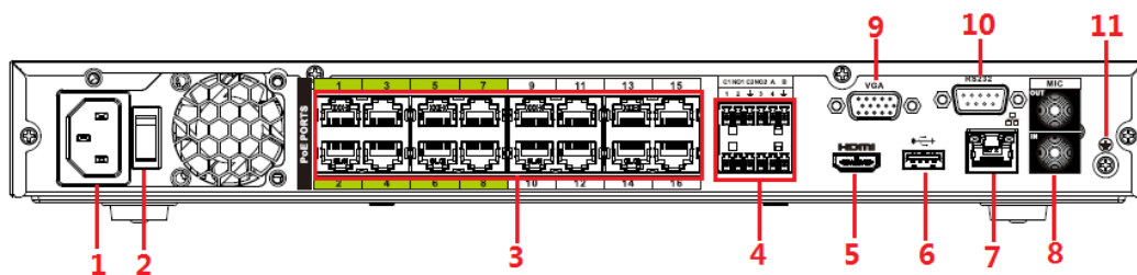
Figura 2-71 Panoul din spate
