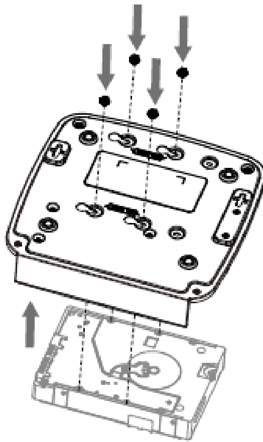
Figura 3-4 Fixați șuruburile
