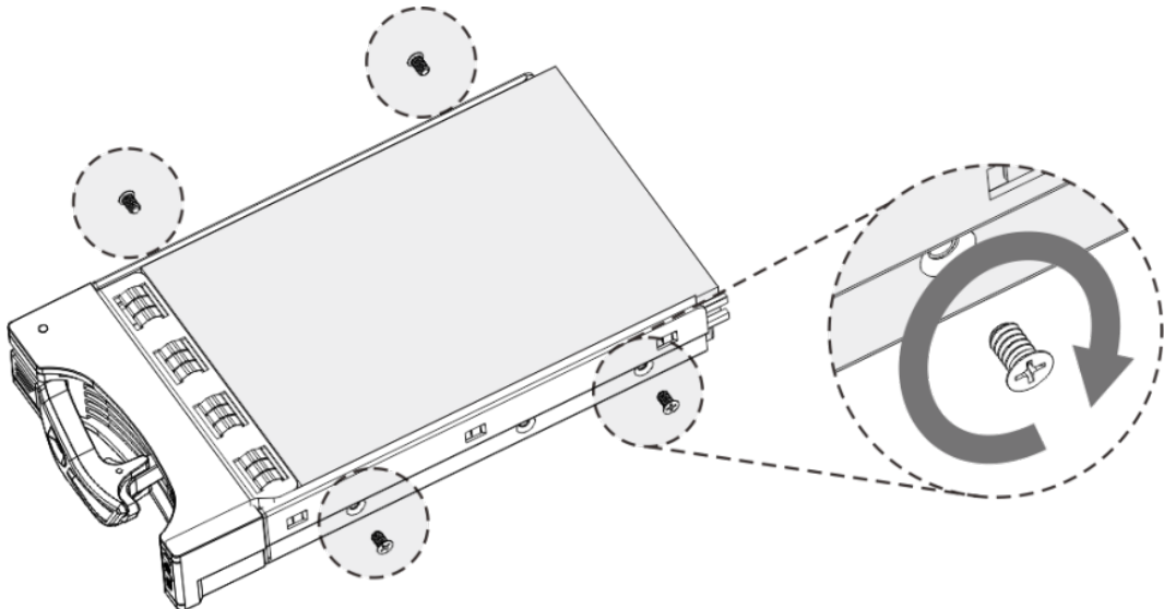
Figura 3-35 Fixați șuruburile
