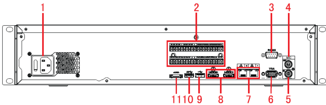
Figura 2-76 Panoul din spate (3)
