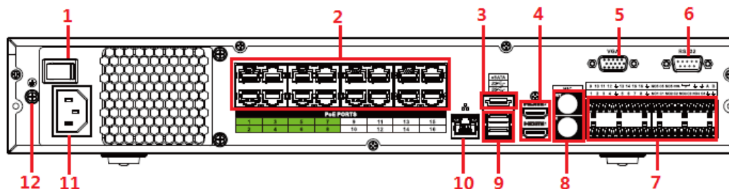
Figura 2-70 Panoul din spate
