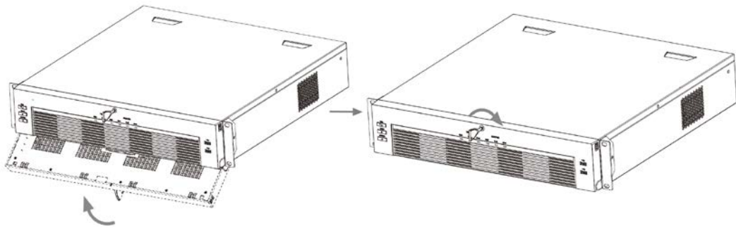
Figura 3-32 Blocarea panoului frontal
