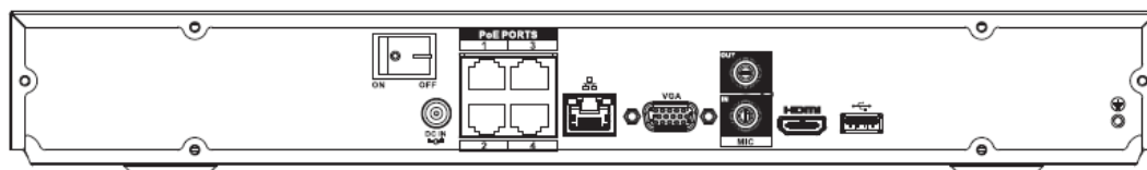
Figura 2-32 Panoul din spate
