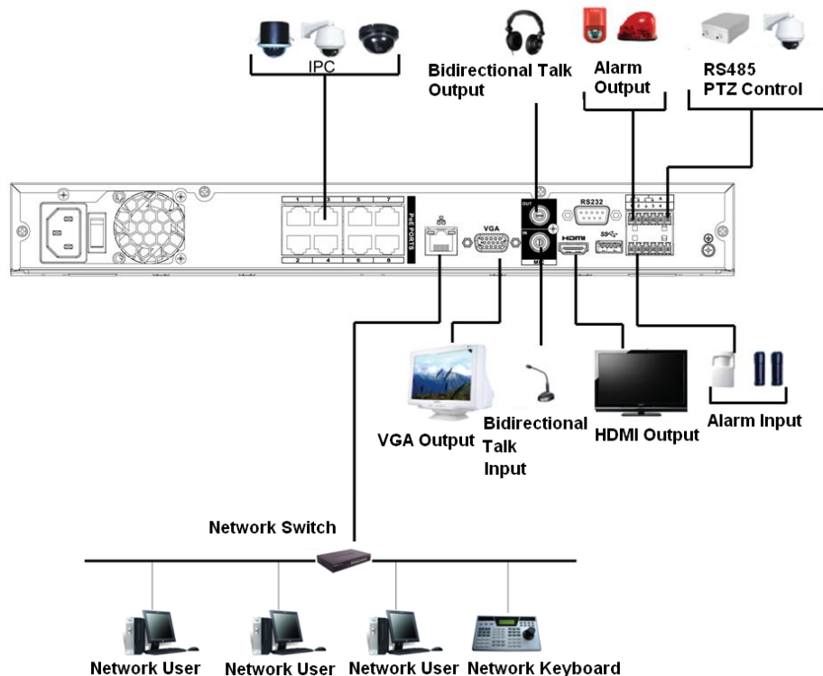
Figura 3-52 Conexiune tipică
