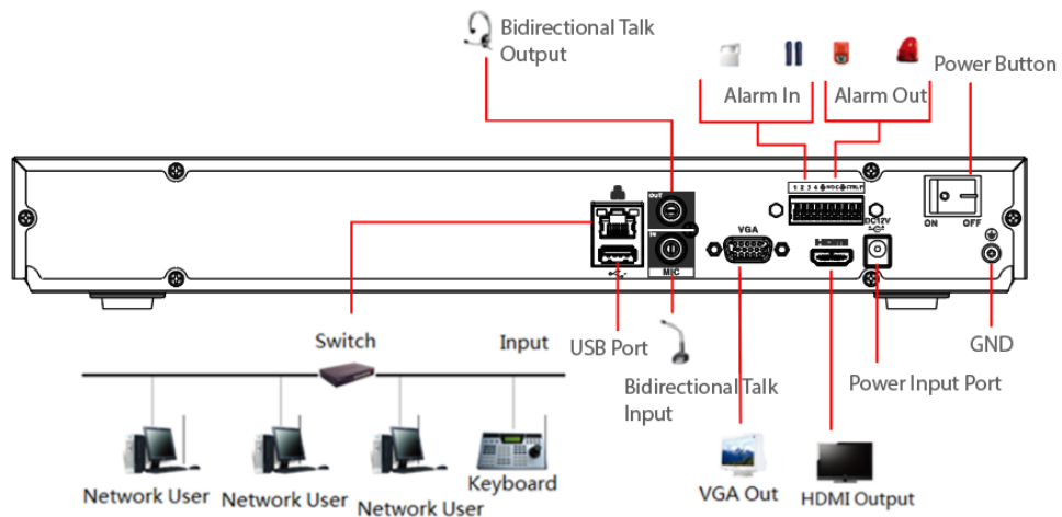
Figura 3-60 Conexiune tipică
