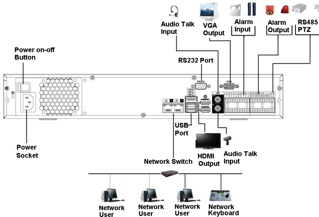
Figura 3-54 Conexiune tipică
