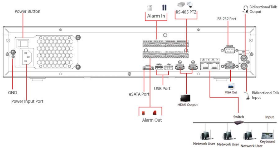
Figura 3-61 Conexiune tipică
