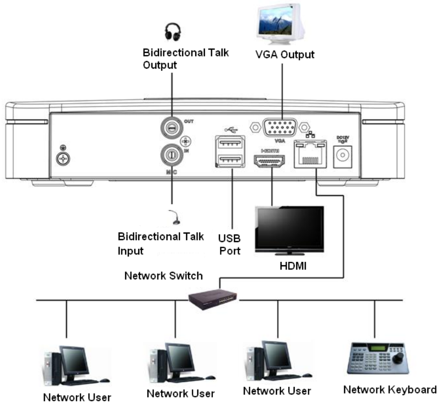
Figura 3-48 Conexiune tipică
