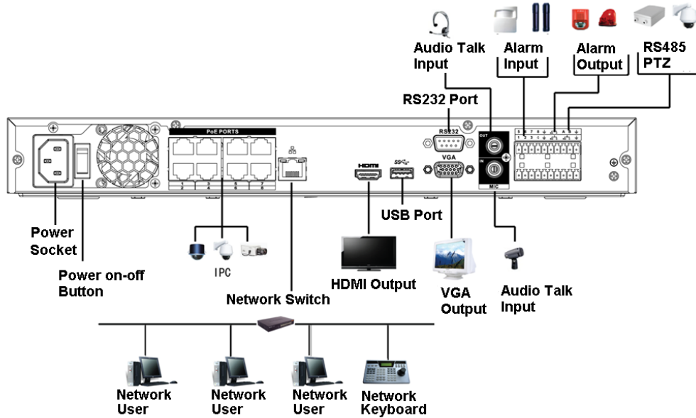
Figura 3-53 Conexiune tipică
