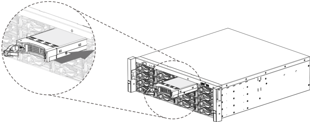
Figura 3-36 Închideți mânerul
