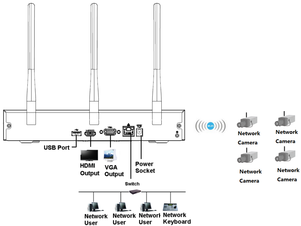
Figura 3-49 Conexiune tipică
