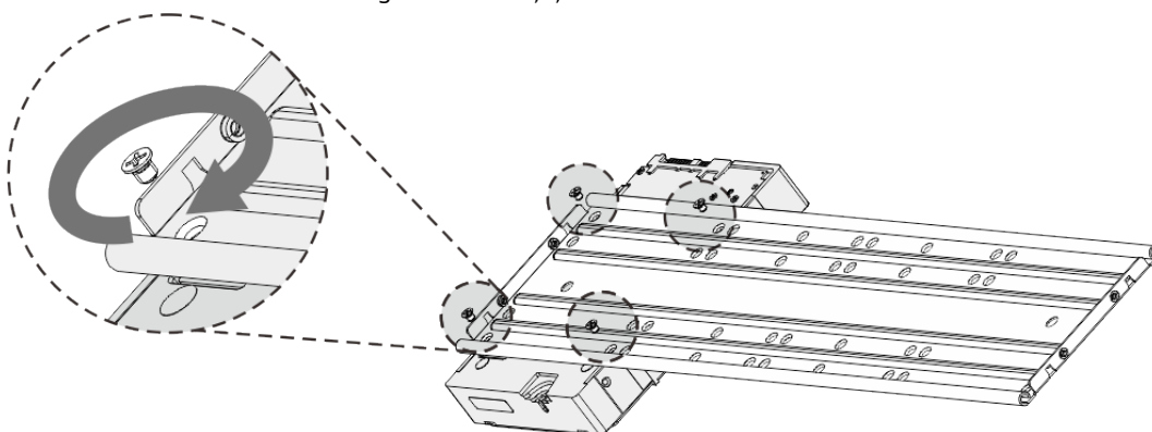
Figura 3-22 Fixați șuruburile
