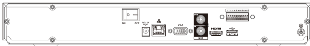
Figura 2-47 Panoul din spate
