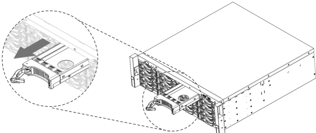
Figura 3-33 Scoateți caseta HDD
