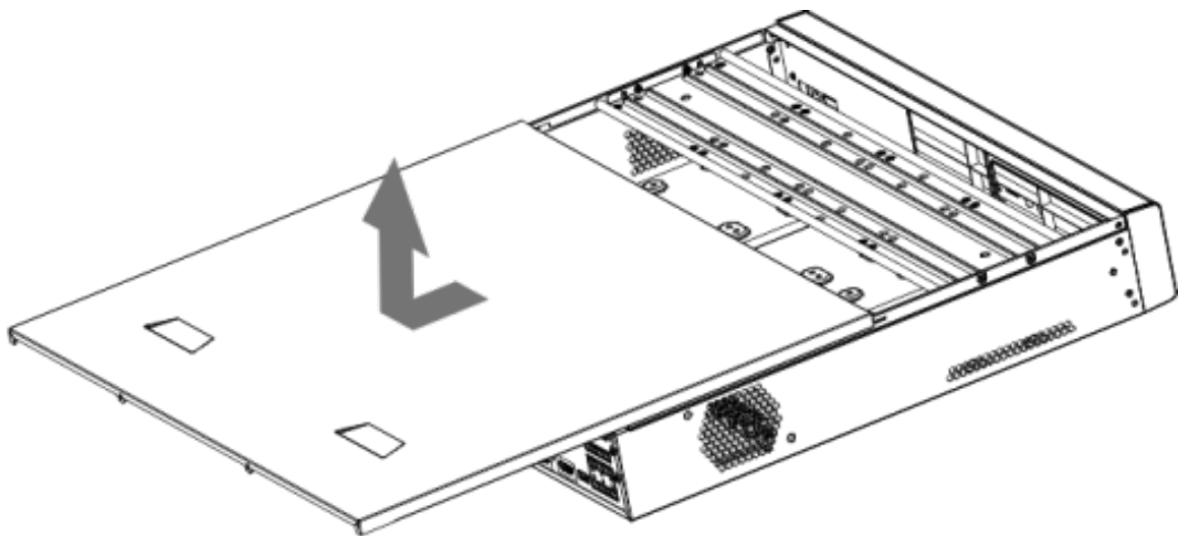
Figura 3-19 Scoateți capacul
