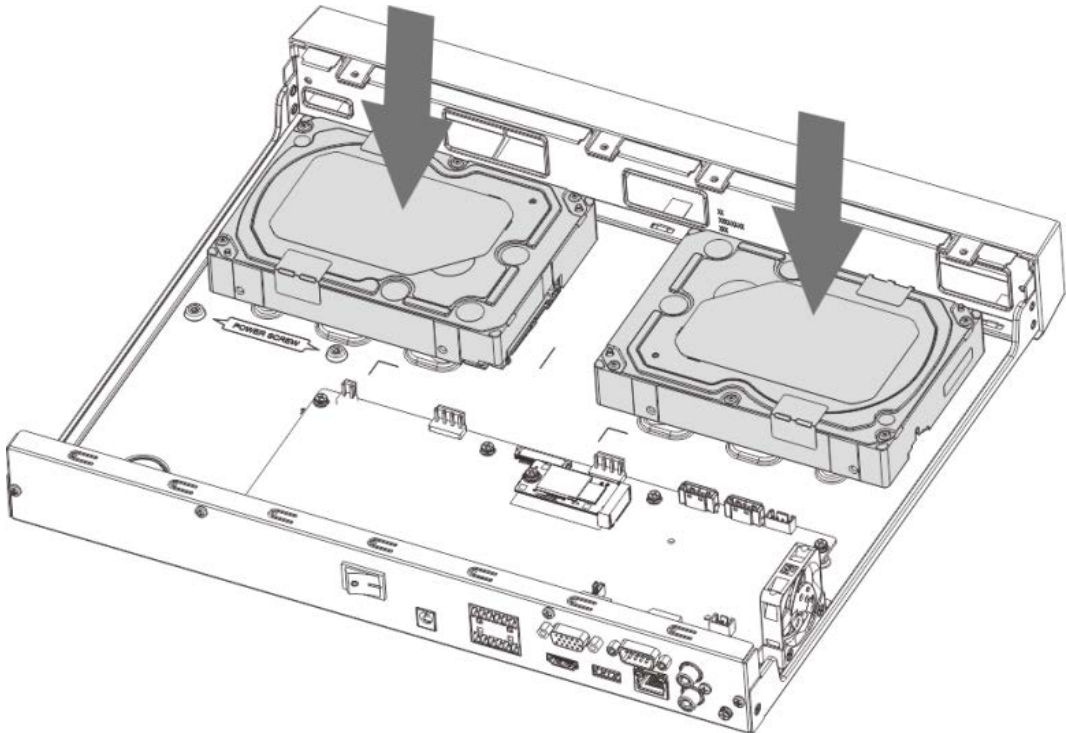
Figura 3-14 Aliniați HDD
