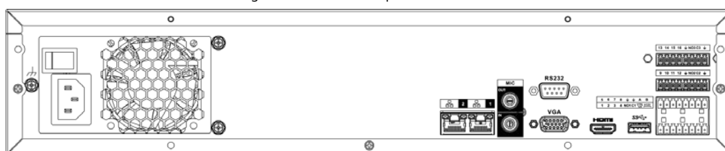
Figura 2-53 Panoul din spate
