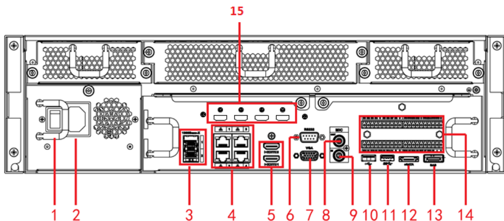
Figura 2-78 Panoul din spate
