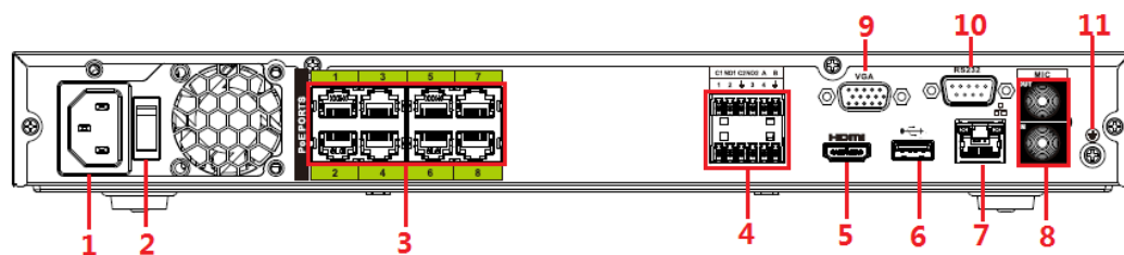
Figura 2-72 Panoul din spate
