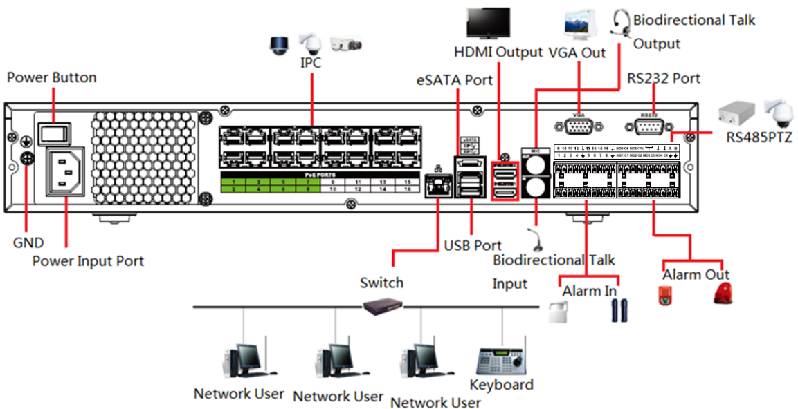
Figura 3-58 Conexiune tipică
