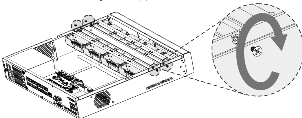
Figura 3-25 Fixați șuruburile
