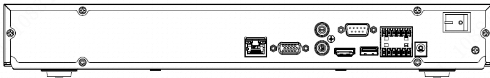
Figura 2-34 Panoul din spate
