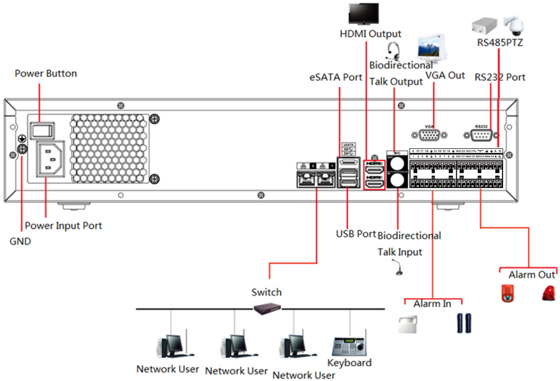
Figura 3-57 Conexiune tipică
