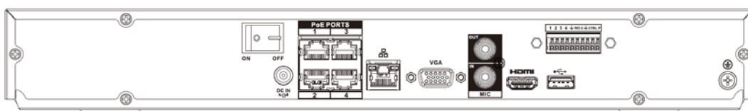
Figura 2-48 Panoul din spate
