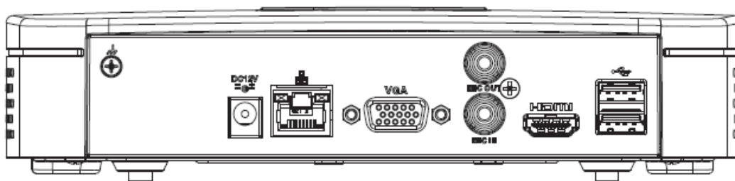
Figura 2-25 Panoul din spate
