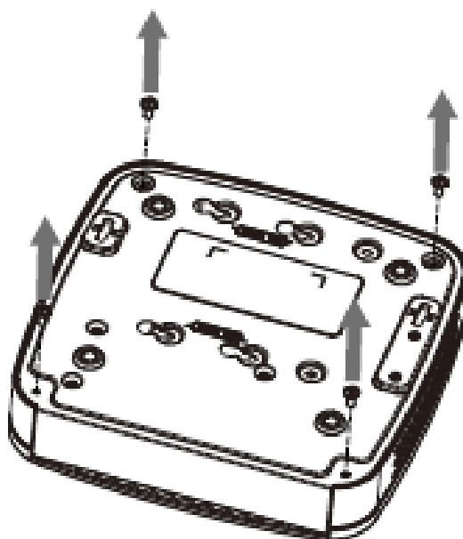
Figura 3-2 Losen șuruburi
