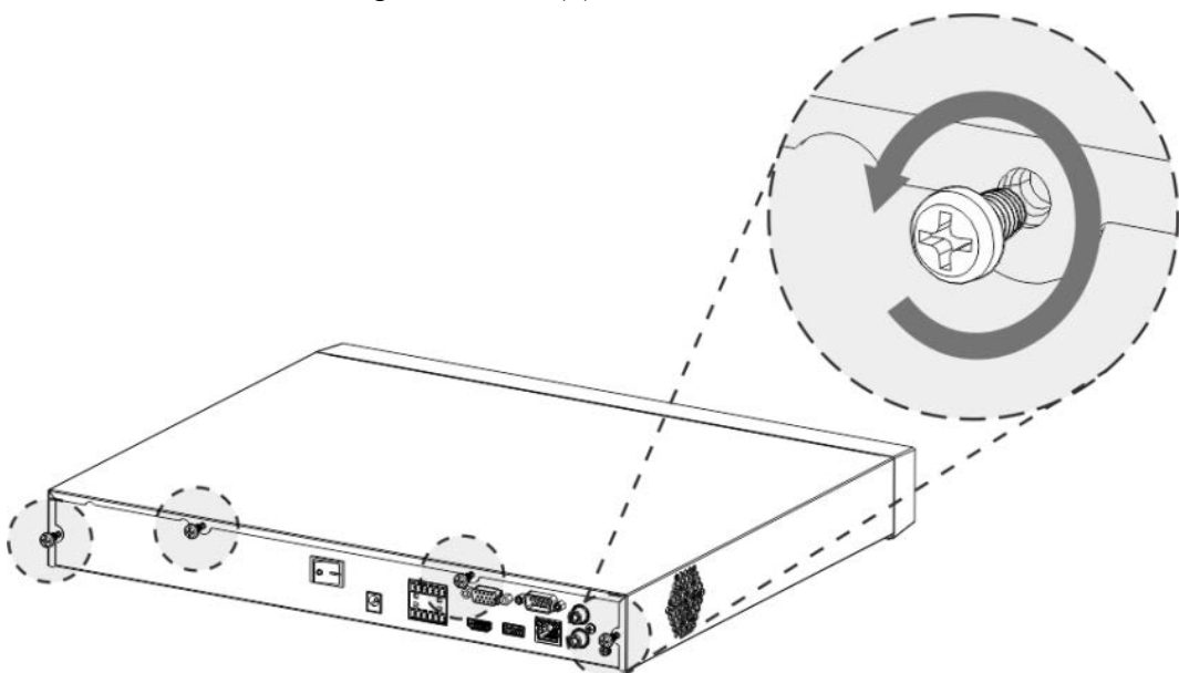
Figura 3-12 Scoateți șuruburile
