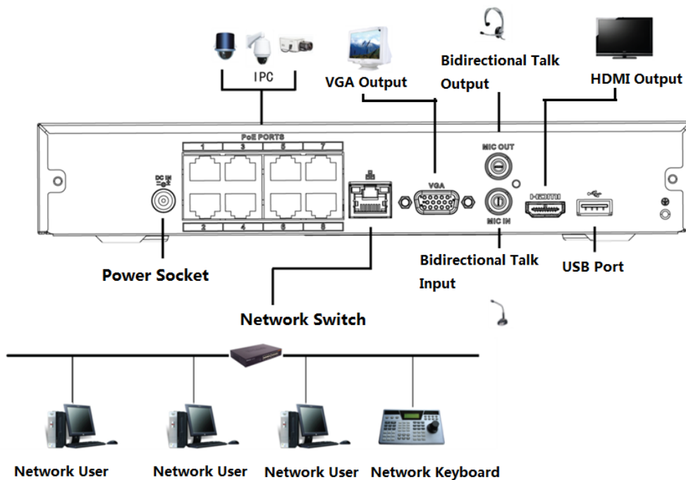
Figura 3-50 Conexiune tipică
