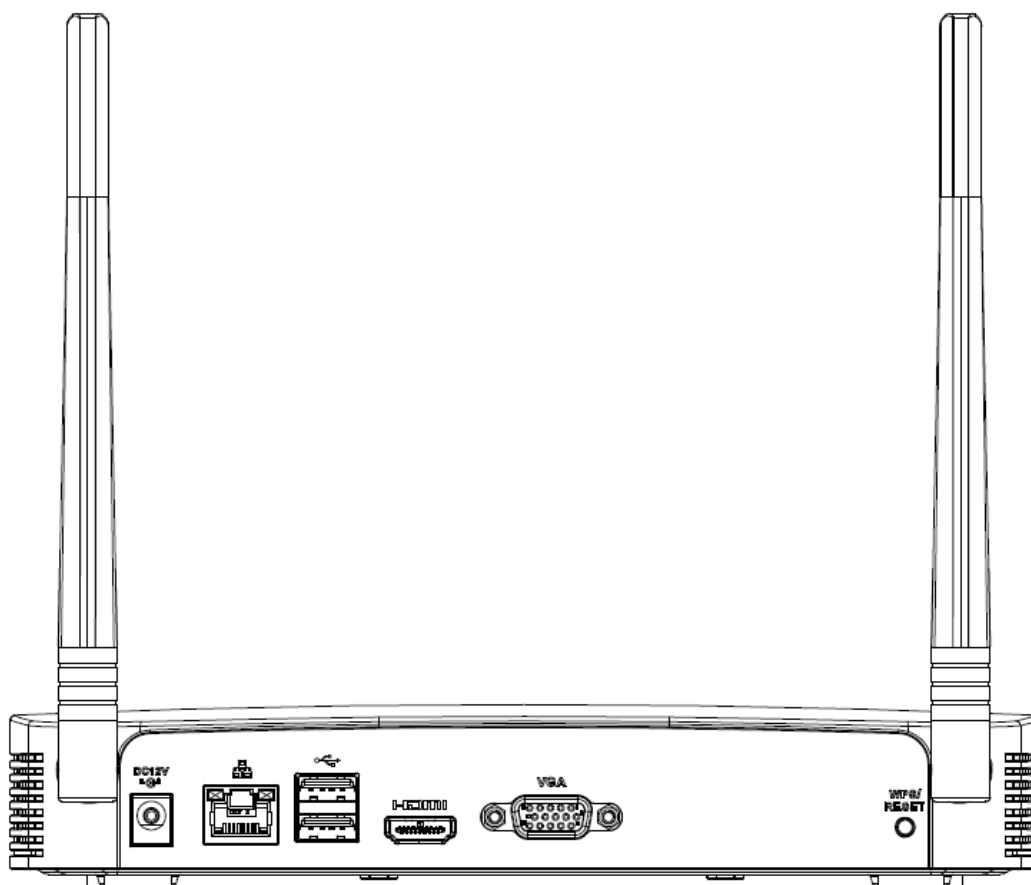
Figura 2-55 Panoul din spate
