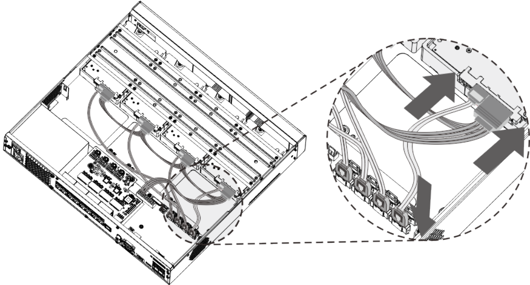
Figura 3-26 Conectați cablurile
