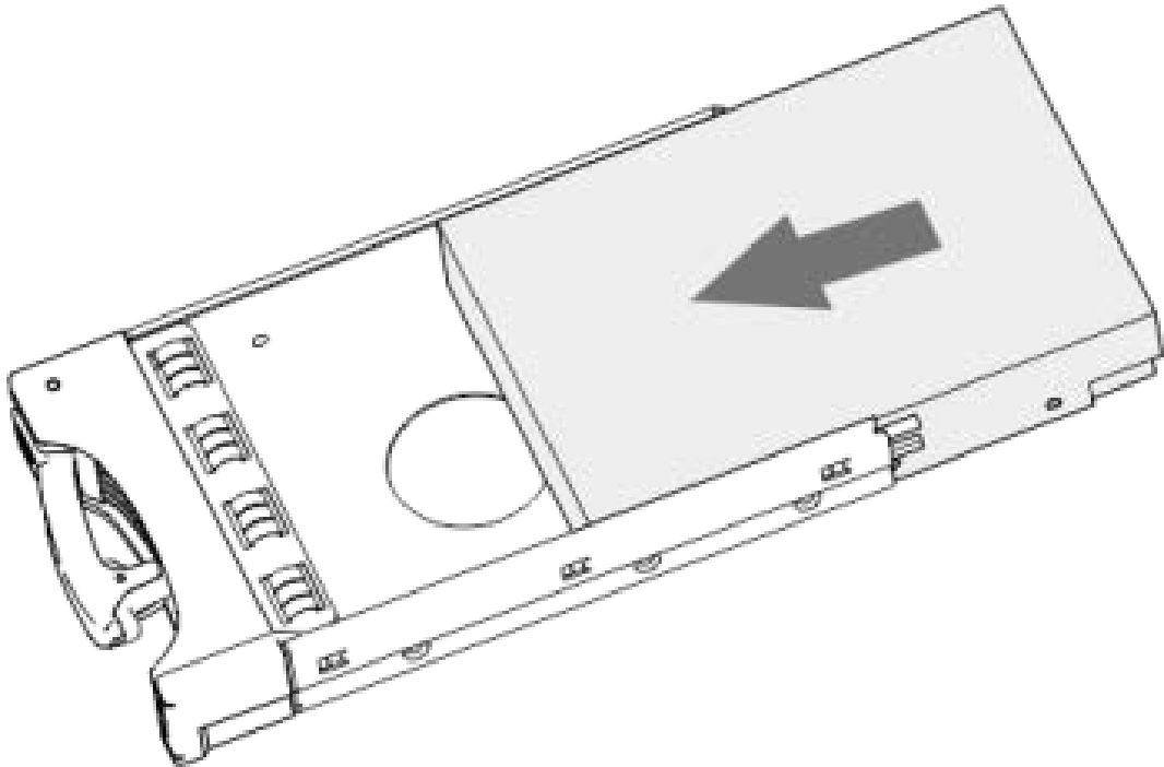
Figura 3-34 Pune HDD în casetă
