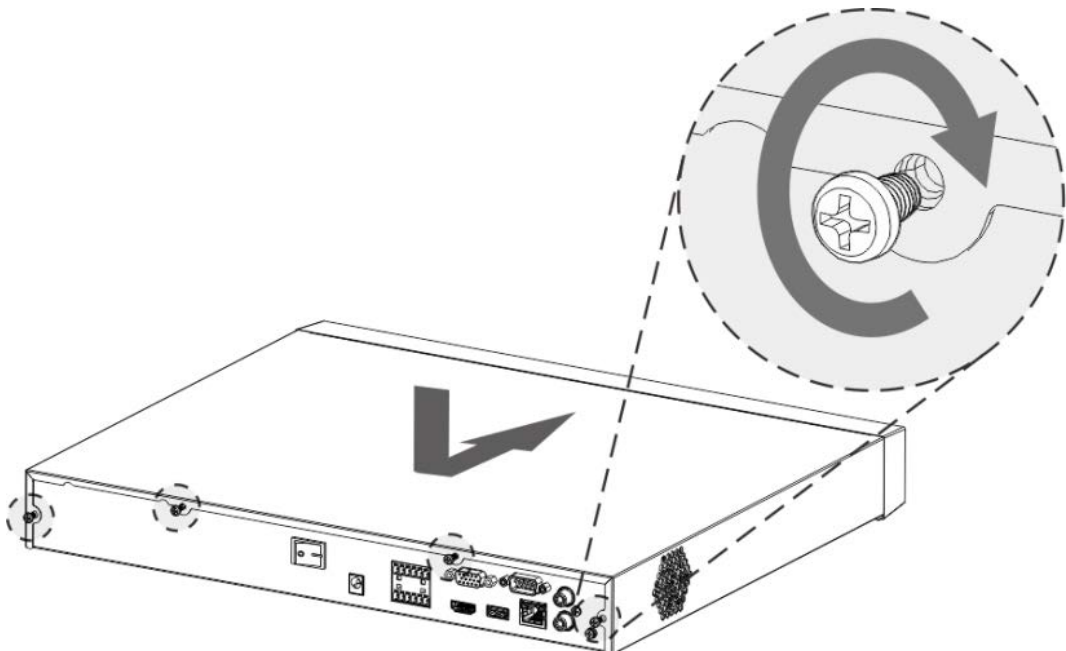
Figura 3-17 Puneți capacul din spate
