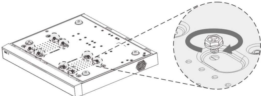
Figura 3-15 Fixați șuruburile
