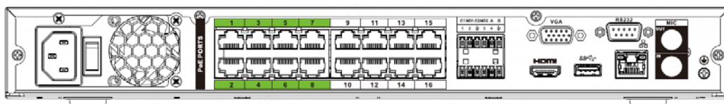
Figura 2-38 Panoul din spate
