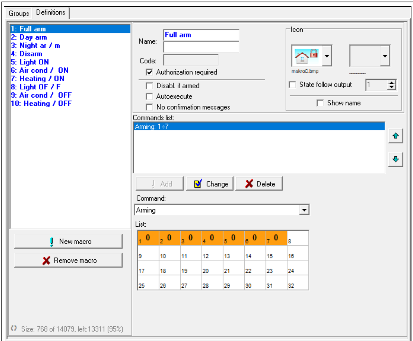
Fig. 11. DLOADX program: “Definitions” tab.
