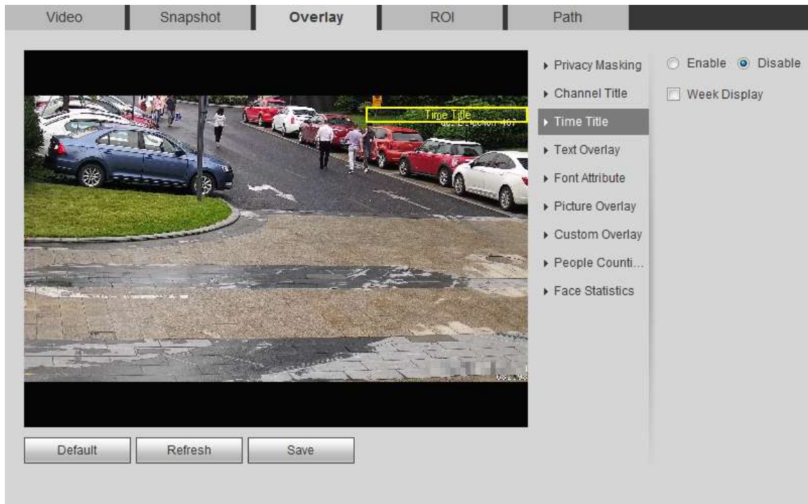
Figura 4-59 Titlul timpului
