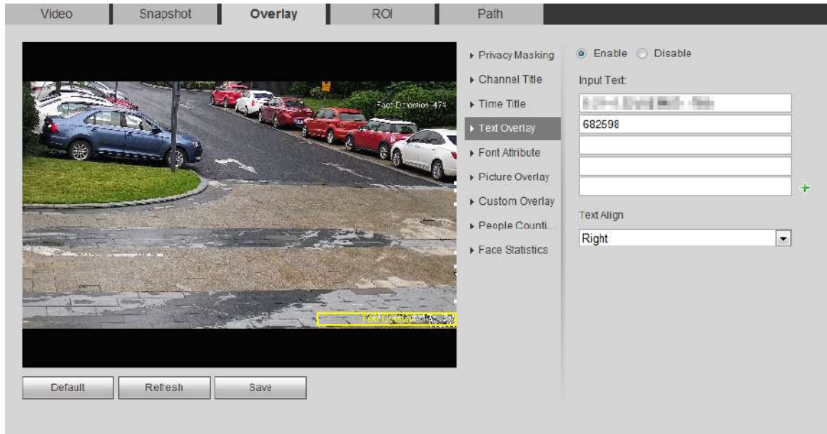
Figura 4-60 Suprapunere text
