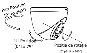
Figura 2-9 Ajustare pe 3 axe
