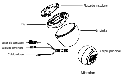
Figura 1-5 Prezentare generală a camerei de tip V
