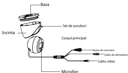
Figura 1-4 Prezentare generală a camerei de tip IV
