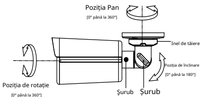
Figura 2-2 Ajustarea pe 3 axe
