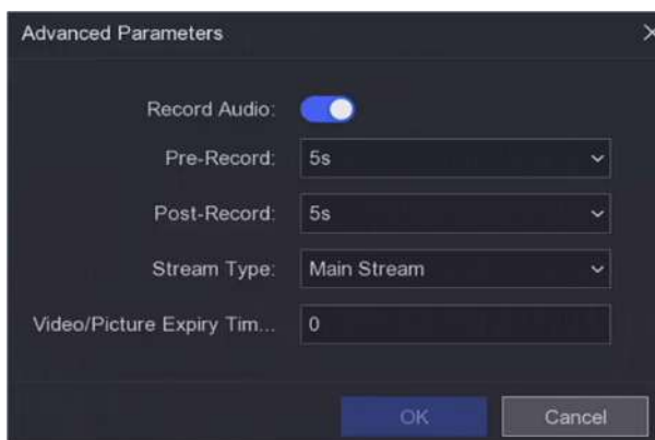
Figura 6-28 Parametri avansati
