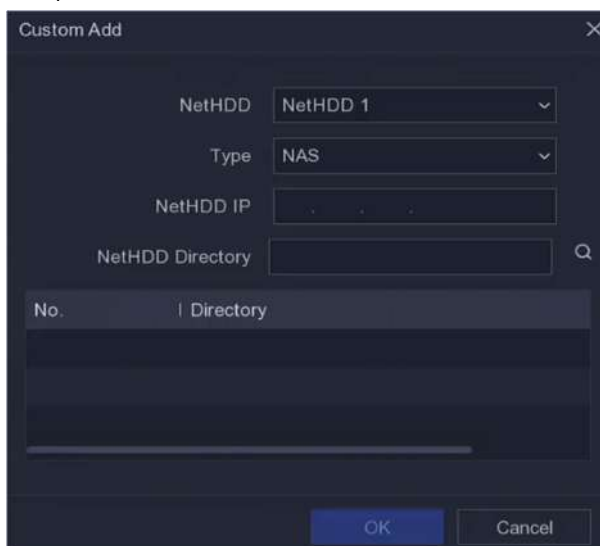
Figura 6-29 Adăugați NetHDD
