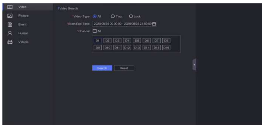
Figura 4-1 Căutare
