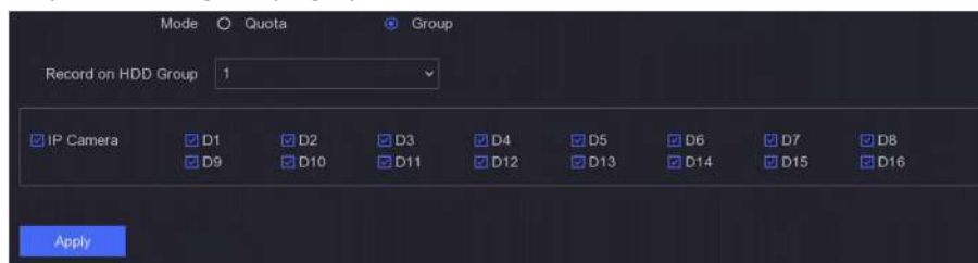
Figura 6-30 Grup
