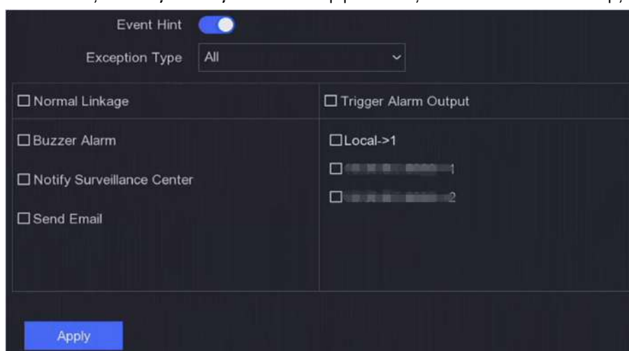
Figura 5-3 Excepții
