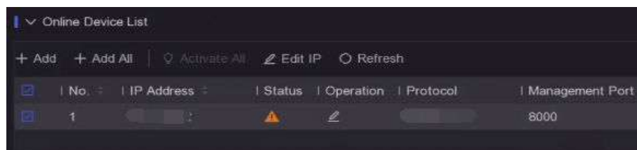
Figura 6-11 Dispozitiv online
