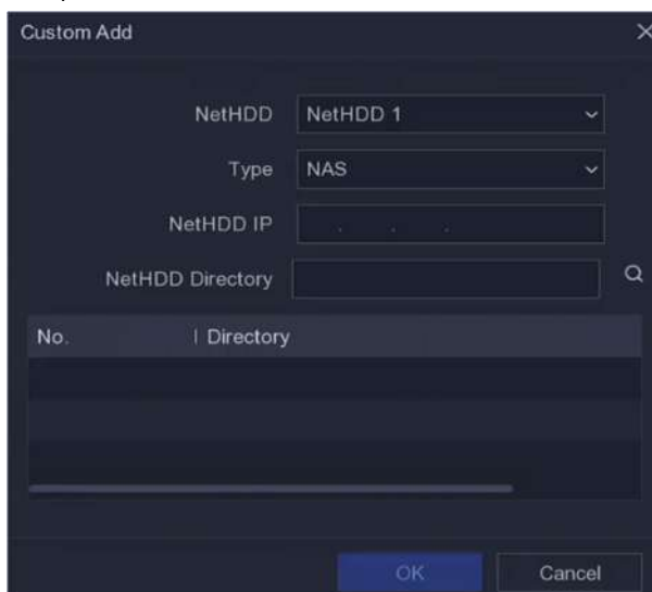
Figura 5-12 Adăugați NetHDD
