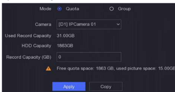
Figura 6-31 Cotă
