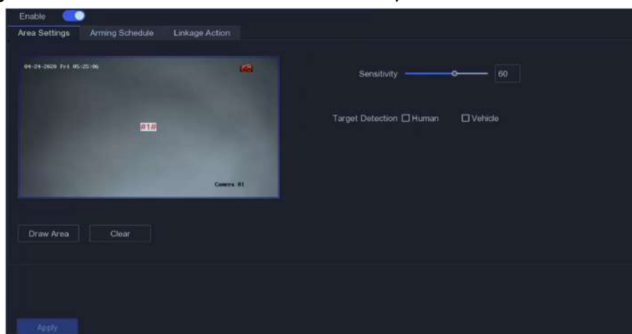
Figura 5-10 Detectarea mișcării
