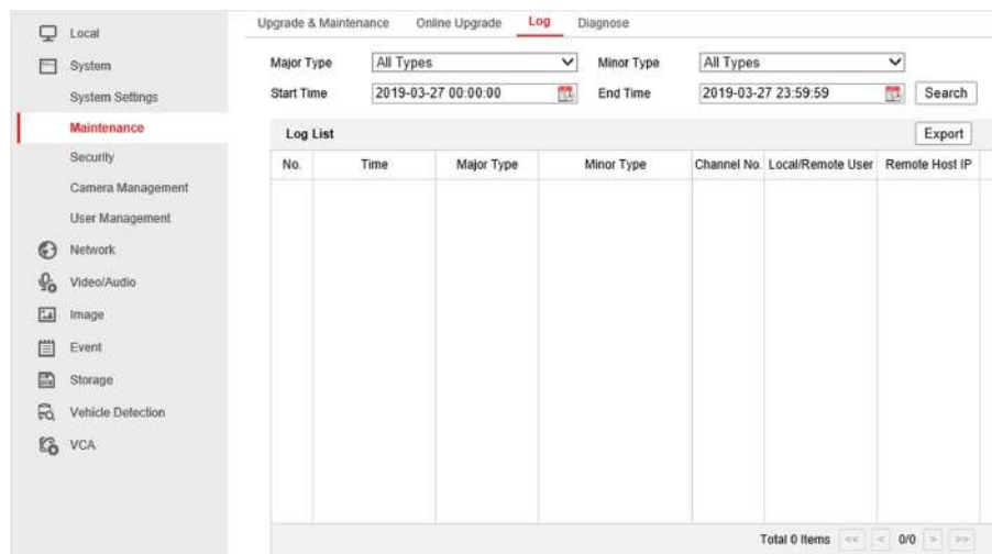
Figura 9-5 Jurnal
