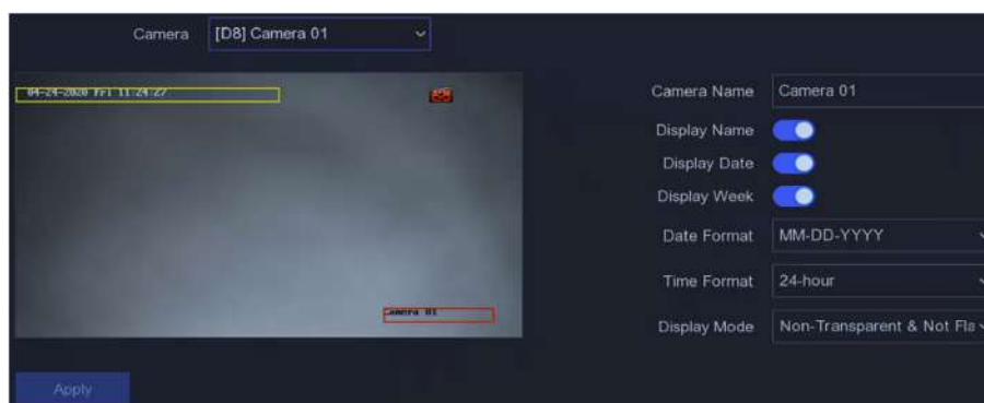
Figura 5-9 OSD
