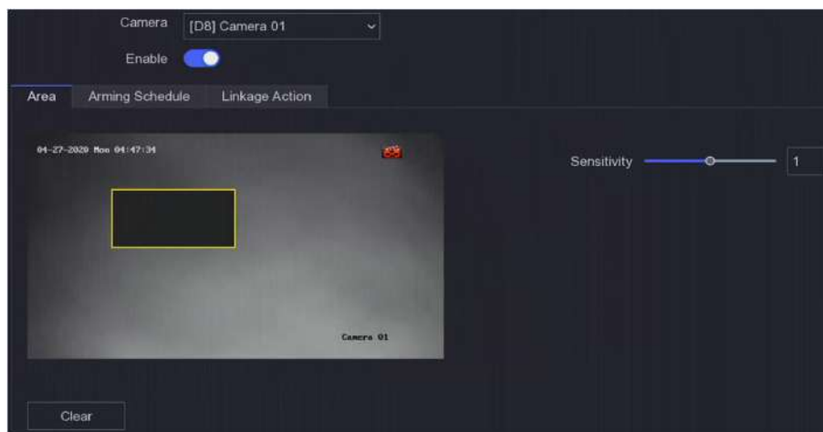
Figura 6-19 Modificare video
