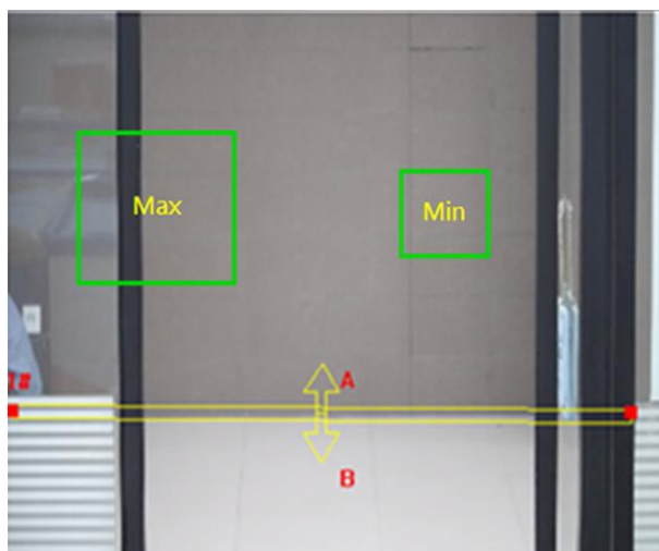
Figura 6-5 Setează regula
