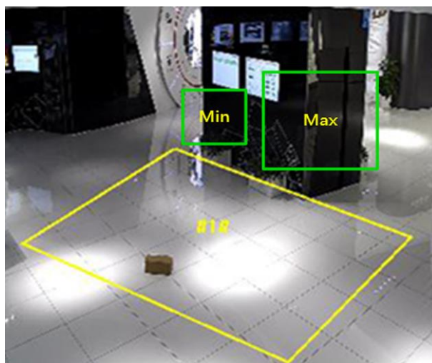
Figura 6-8 Setează regula
