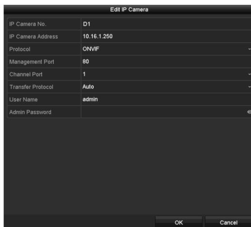
Figura 2-40 Editare cameră IP
