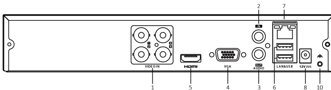
Figura 1-4 Panoul din spate al HWD-6100MH-G2
