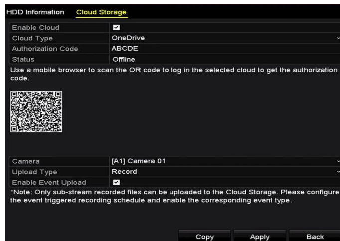
Figura 12-20 Încărcare în interfața de stocare în cloud
