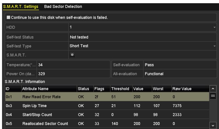
Figura 12-28 Interfața de setări SMART
