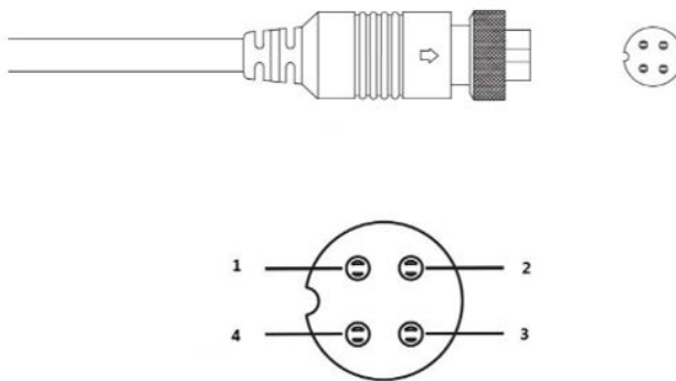
Figura 2-9 Conector pentru aviație HDCVI
