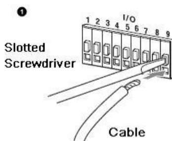
Figura 8-4 Instalați cablul
