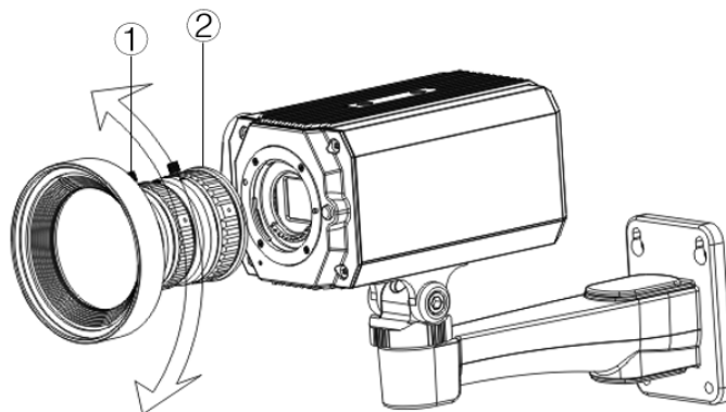
Figura 8-3 Instalarea obiectivului (2)
