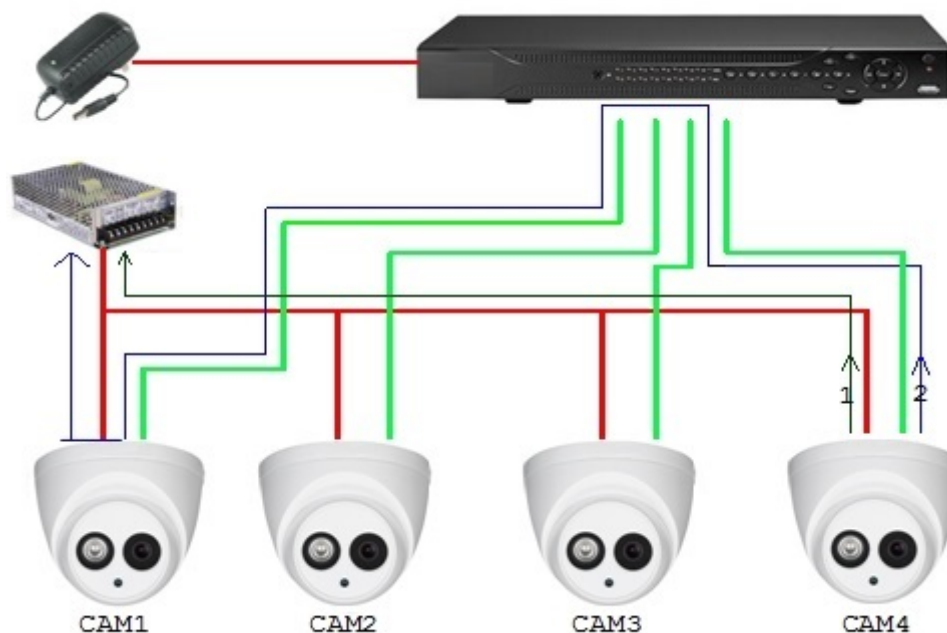
Figura 10-1 Principiul alimentării centralizate
