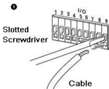
Figura 9-4 Instalați cablul
