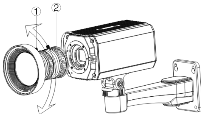
Figura 9-3 Instalarea obiectivului (2)
