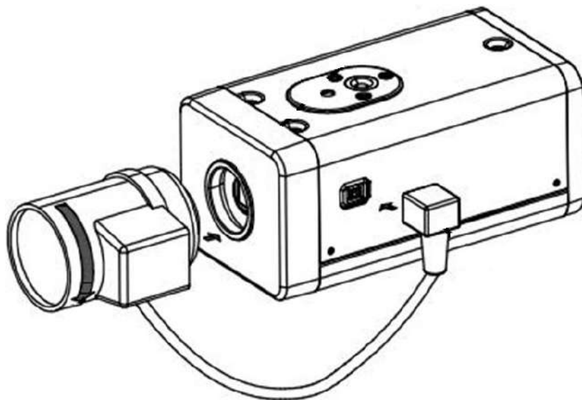
Figura 9-1 Instalarea obiectivului (1)
