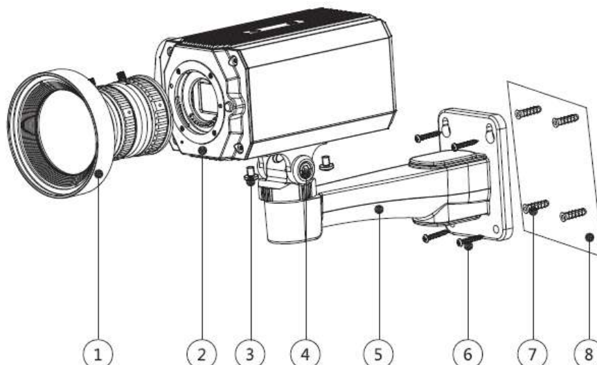
Figura 9-6 Componentele dispozitivului
