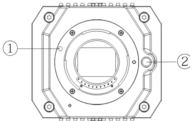
Figura 9-2 Panoul frontal
