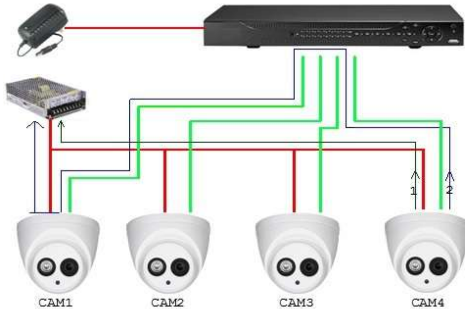
Figura 11-1 Principiul alimentării centralizate
