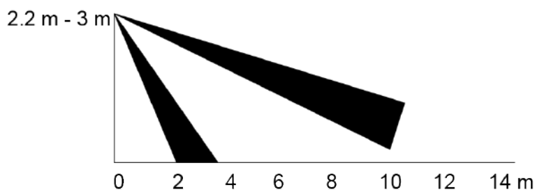
Figura 7-2 Distanța de detectare verticală
