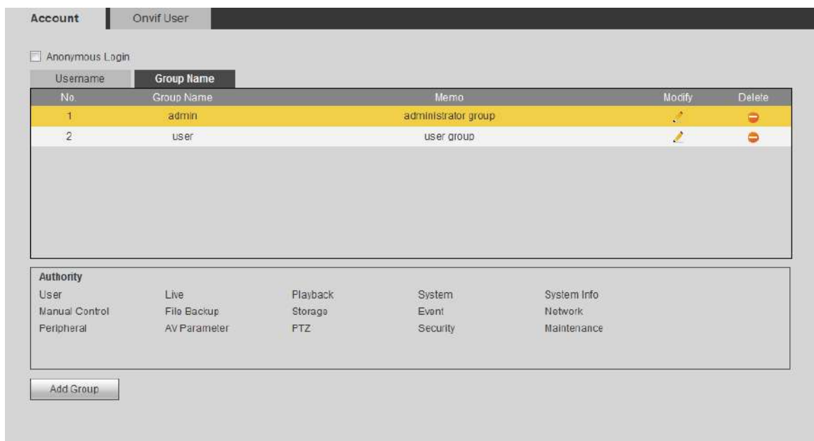
Figura 4-107 Nume grup
