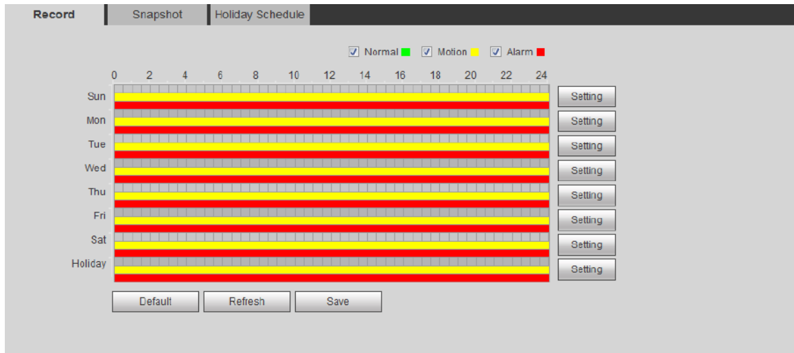
Figura 5-3 Înregistrare
