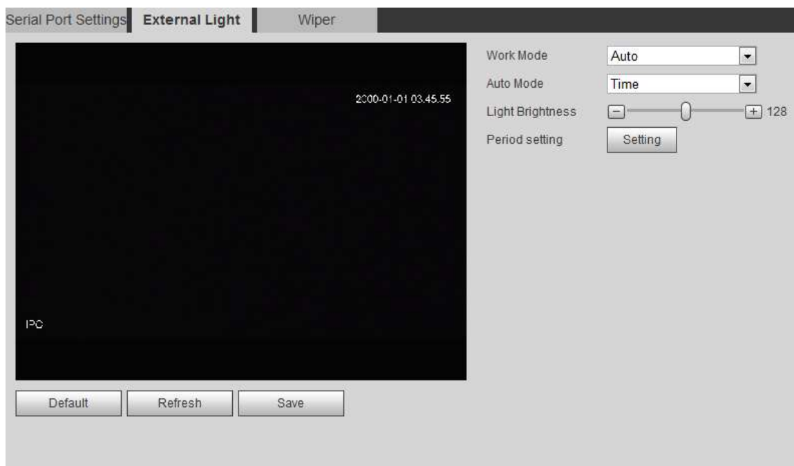
Figura 4-126 Lumină externă
