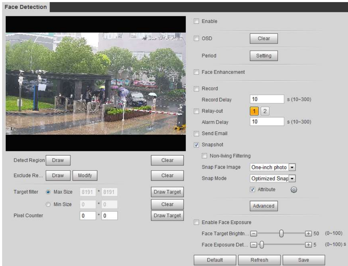
Figura 5-62 Detectarea feței
