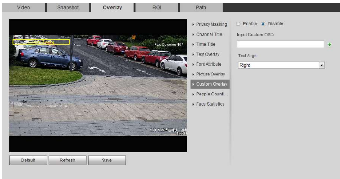
Figura 4-63 Suprapunere personalizată
