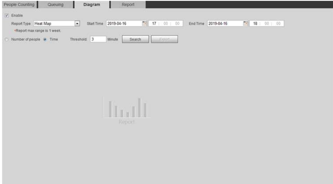
Figura 5-70 Diagrama
