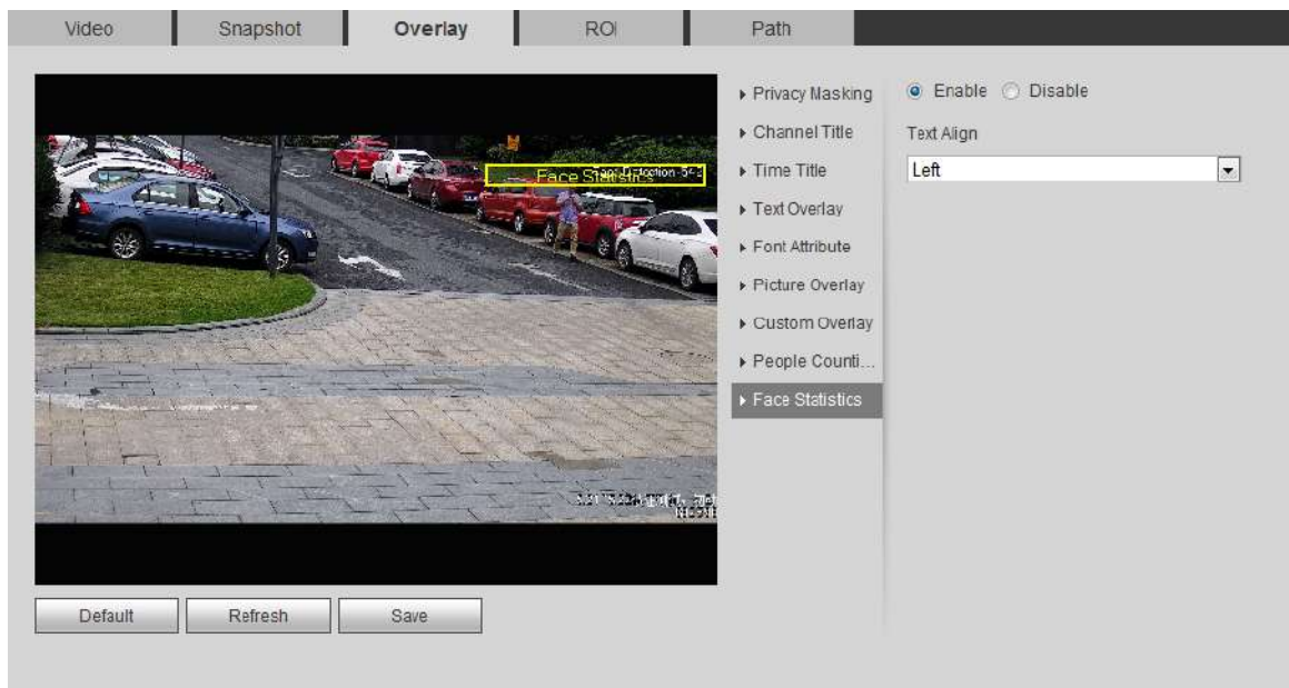
Figura 4-70 Statistici faciale
