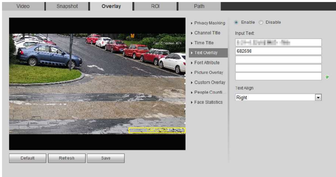
Figura 4-60 Suprapunere text
