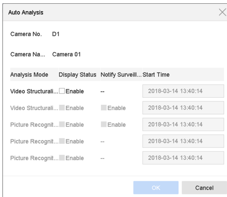
Figura 5-2 Analiză automată
