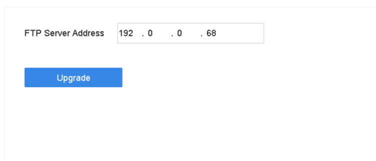
Figura 12-11 Actualizare FTP
