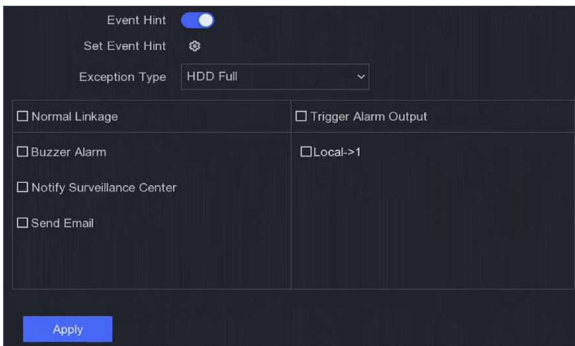
Figura 6-21 Excepții
