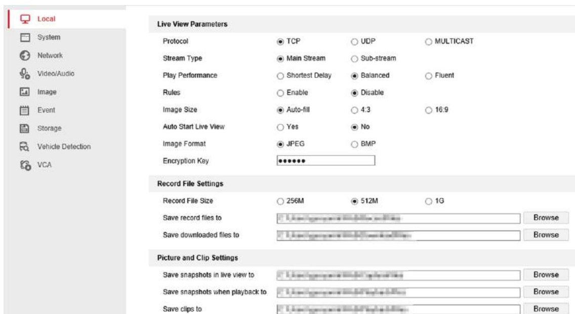
Figura 9-4 Configurare
