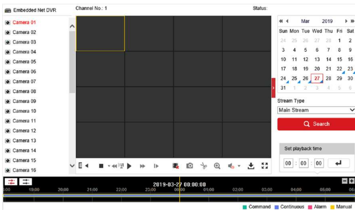
Figura 9-3 Redare
