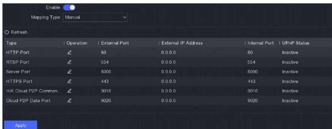
Figura 6-5 NAT
