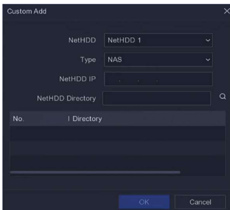
Figura 5-13 Adăugați NetHDD
