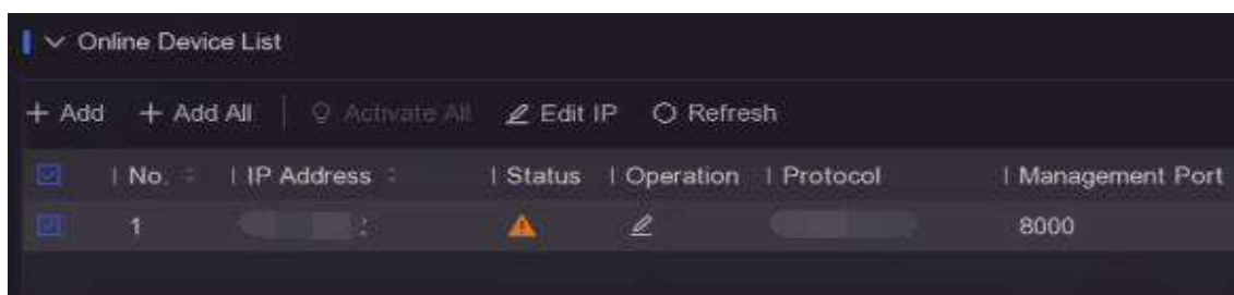
Figura 6-12 Dispozitiv online
