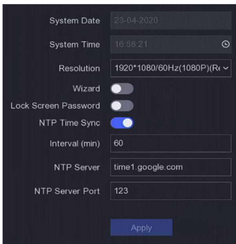
Figura 5-1 Setări generale
