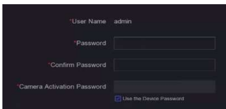
Figura 1-1 Activare
