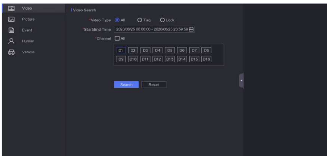
Figura 4-1 Căutare
