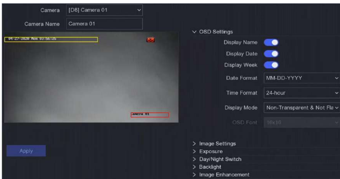
Figura 6-14 OSD
