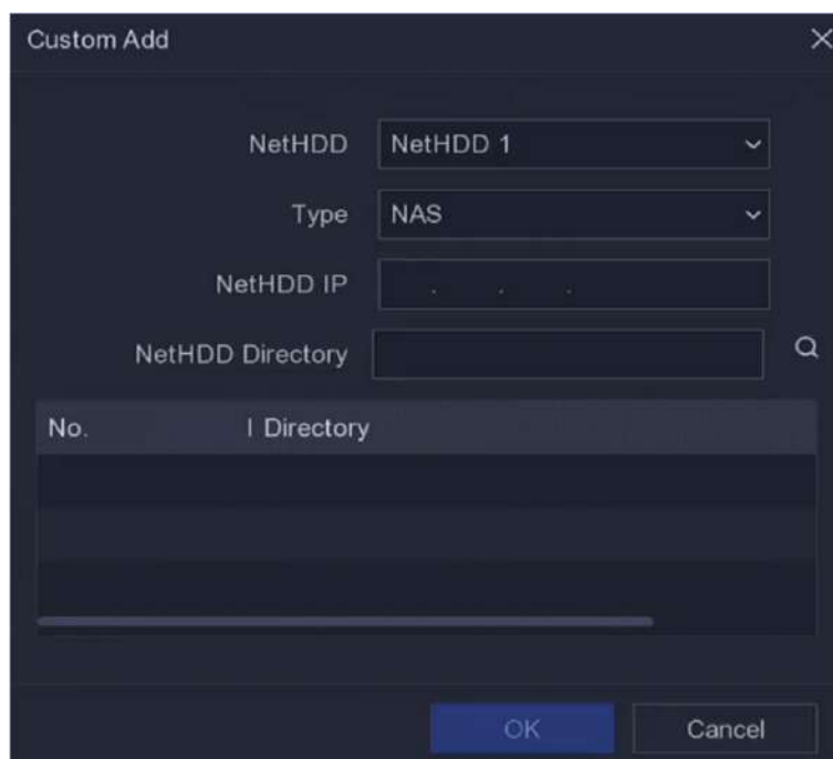
Figura 6-28 Adăugați NetHDD
