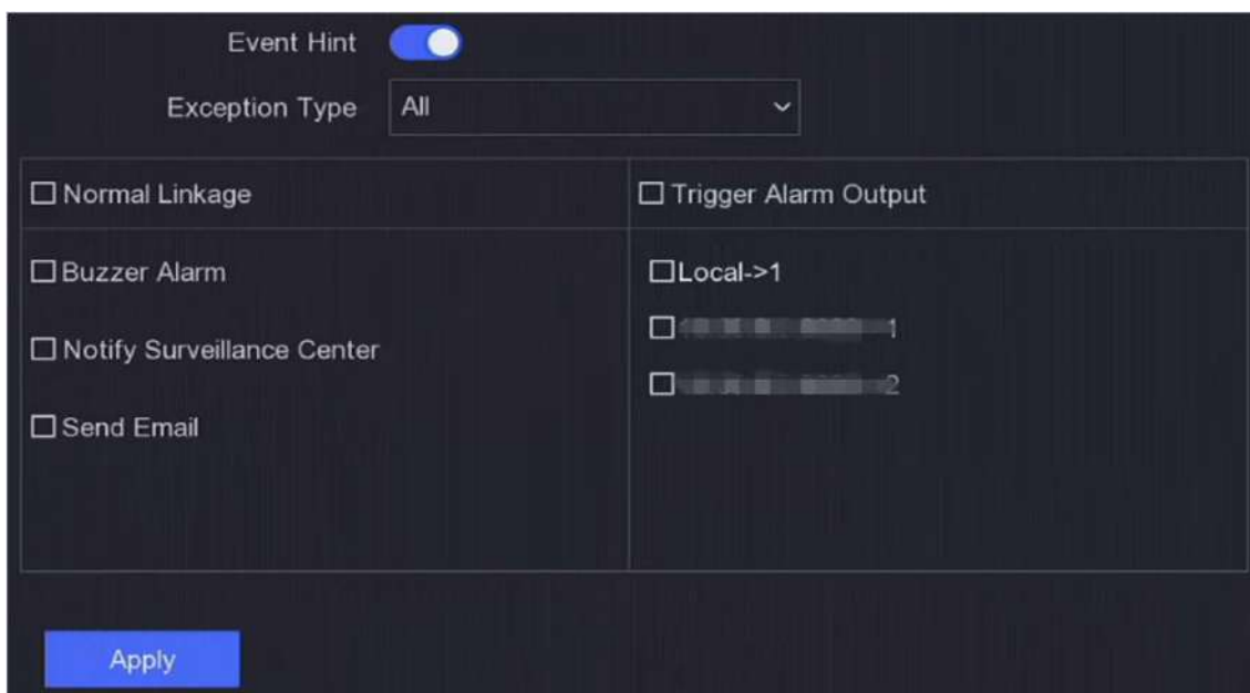
Figura 5-3 Excepții
