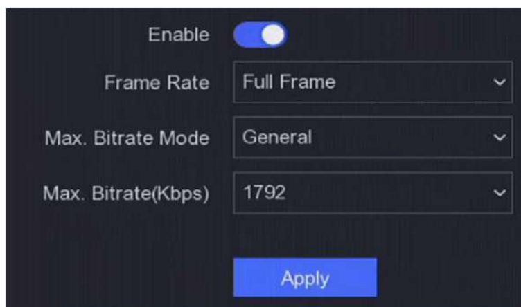
Figura 6-3 Canal-Zero
