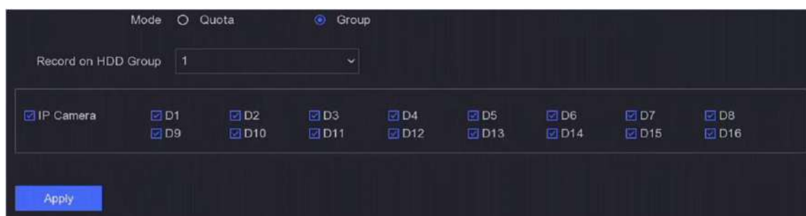
Figura 6-29 Grup
