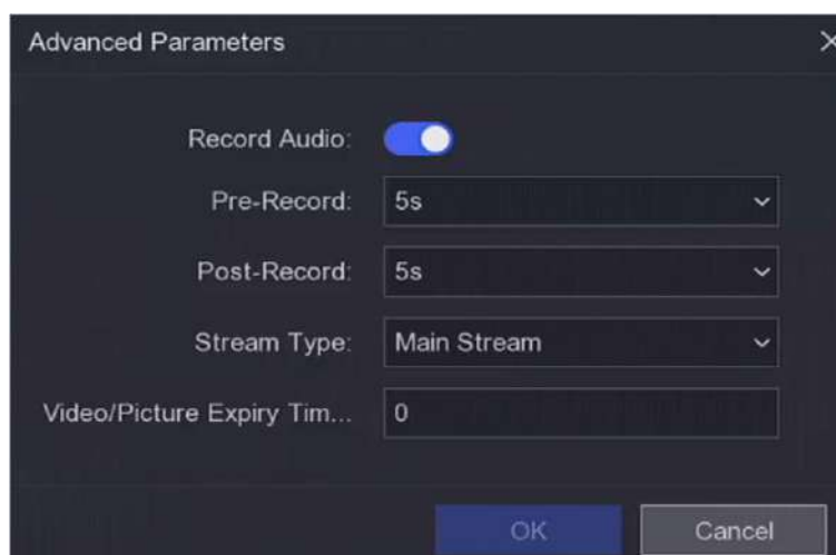
Figura 6-27 Parametri avansati
