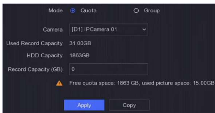
Figura 6-30 Cotă
