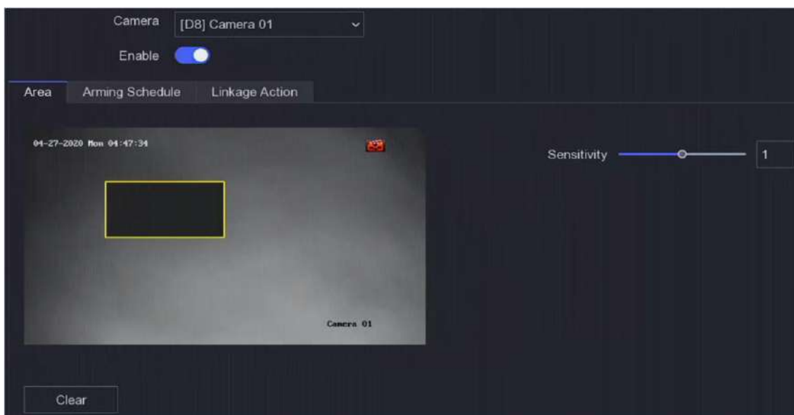
Figura 6-16 Modificare video
