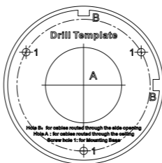
Figura 2-41 Șablon de foraj pentru cutia de jonctiune
