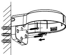
Figura 2-66 Fixați corpul principal pe perete
