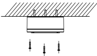
Figura 2-43 Combinați capacul și corpul cutiei de jonctiune
