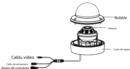
Figura 1-3 Cameră de tip II cu alimentare prin coaxială Cablul
