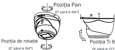
Figura 2-19 Reglare pe 3 axe
