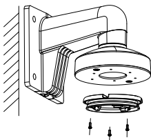
Figura 2-14 Fixați baza
