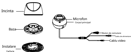
Figura 1-3 Prezentare generală a camerei de tip III
