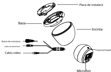
Figura 1-5 Prezentare generală a camerei de tip V
