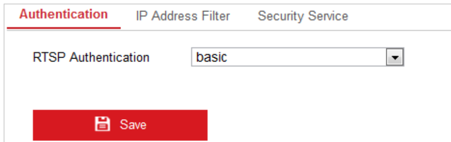
Figura 6-12 Autentificare RTSP
