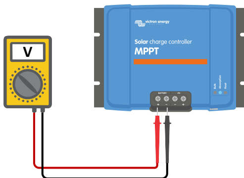
Măsurarea tensiunii bateriei la bornele bateriei regulatorului
