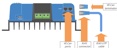
Port VE.Can, conector, cutie terminală și cablu
