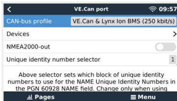
Ecranul GX afișează setarea profilului CAN-bus
