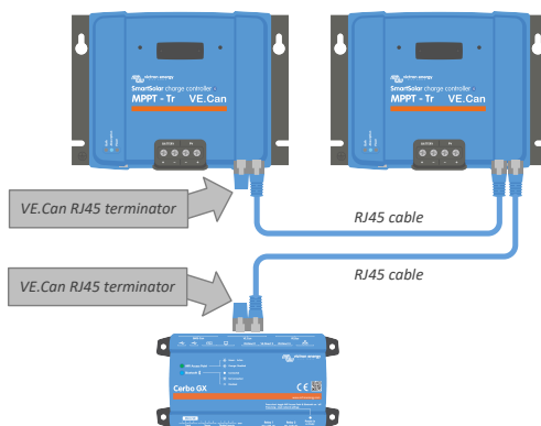
Exemplu de două încărcătoare solare VE.Can conectate la un singur dispozitiv GX
