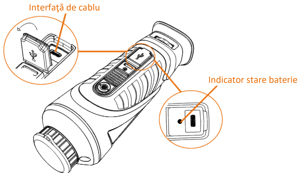
Figura 2-1 Interfață de cablu
