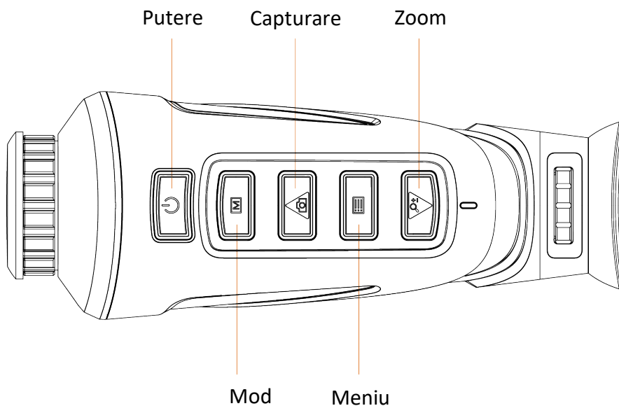
Figura 1-1 Butoane pe dispozitiv
