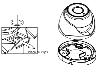
FIG ură 2-8 Scoateți placa de cleme
