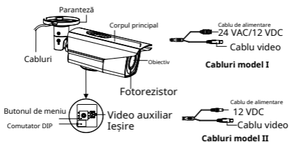
Figura 1-1 Prezentare generală a camerei de tip I
