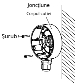
Figura 2-5 Fixați camera de tavan
