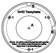
Figura 2-1 Șablon de foraj
