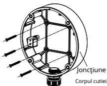
Figura 2-14 Fixați corpul cutiei de joncțiune pe perete /Tavan
