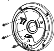
Figura 2-13 Șuruburi de fixare pe capacul cutiei de joncțiune
