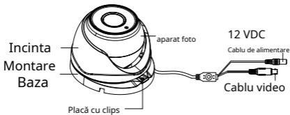
Figura 1-2 Prezentare generală a camerei de tip II
