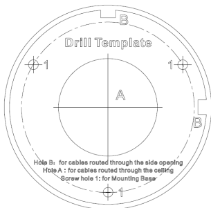
Figura 7, Șablon de foraj al cutiei de jonctiune
