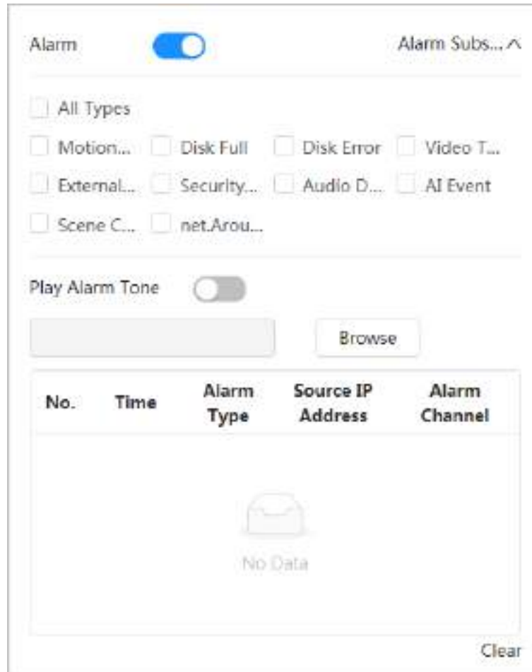
Figure 4-66 Alarm (subscription)
