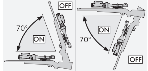
Kiinnitettävä lämpökuvantamislaitte
