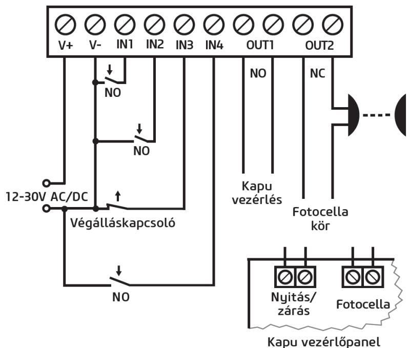
Egy kapu bekötése végálláskapcsolóval és fotocella érzékelőkör-megszakítással (3. vezérlési mód)
