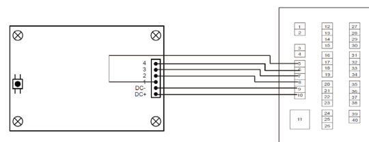
Conectare controler de acces cu taste VZ-FC03
