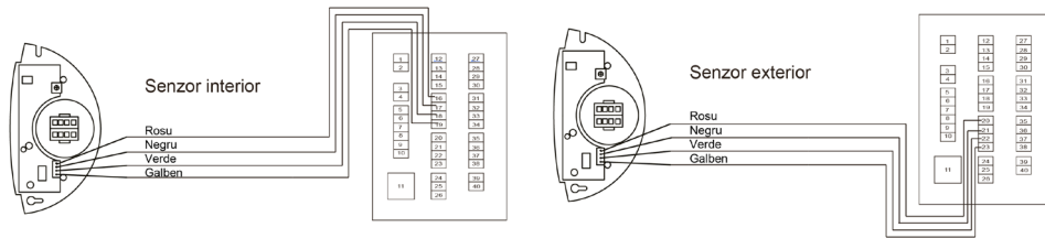
Conectare senzori comanda intrare/iesire
