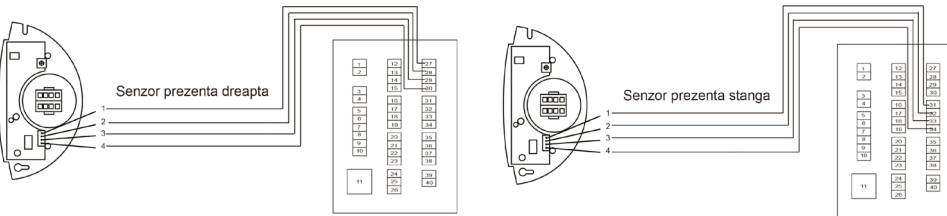
Conectare senzori prezenta
