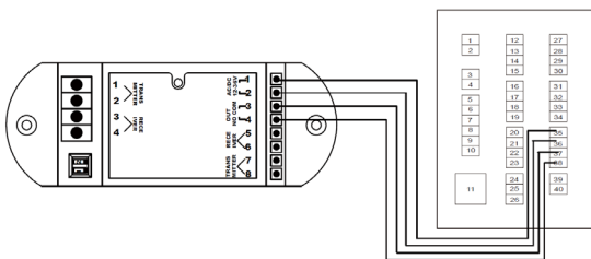
Conectare fotocelule VZ-PT02
