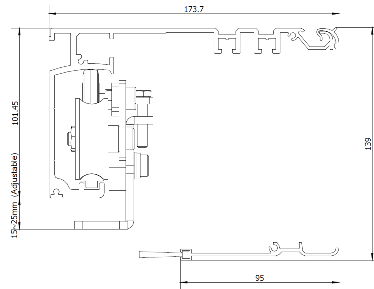
Vedere in sectiune
