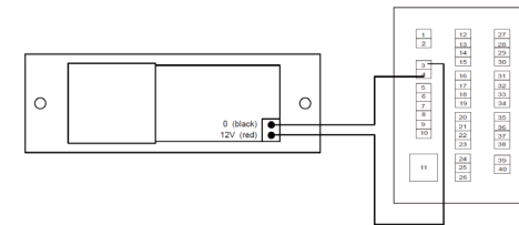
Conectare incuietoare electromagnetica
