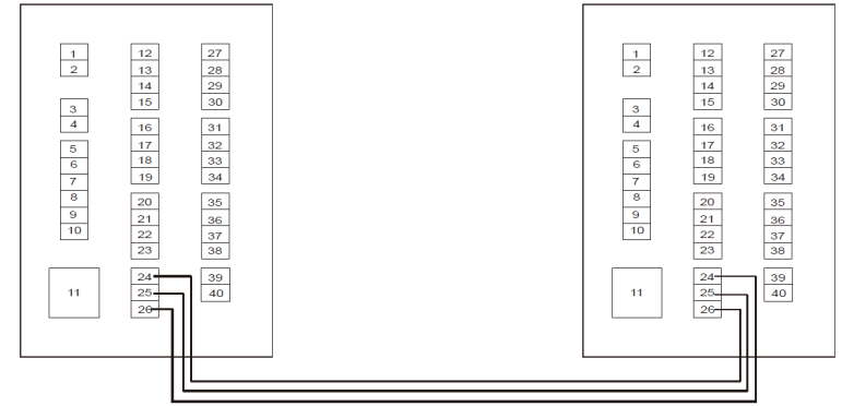
Conectare controler de acces (max. 12Vcc/2A)
