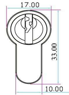
Cilindru standard
