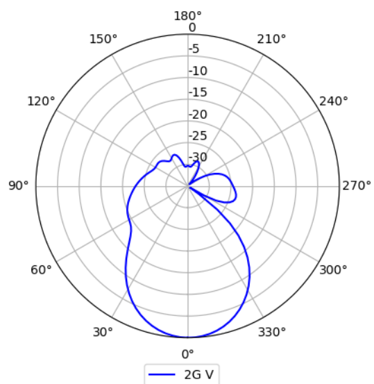
5GHz (Vertical)
